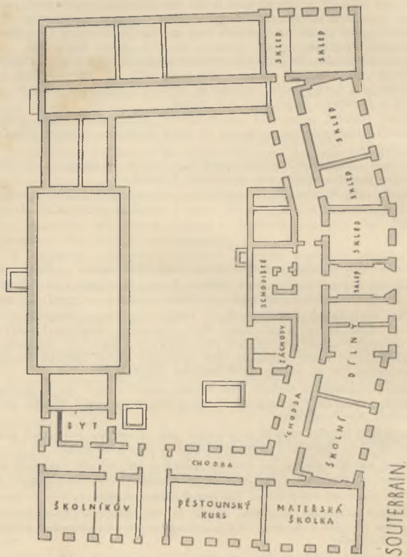
Plán školní budovy.
