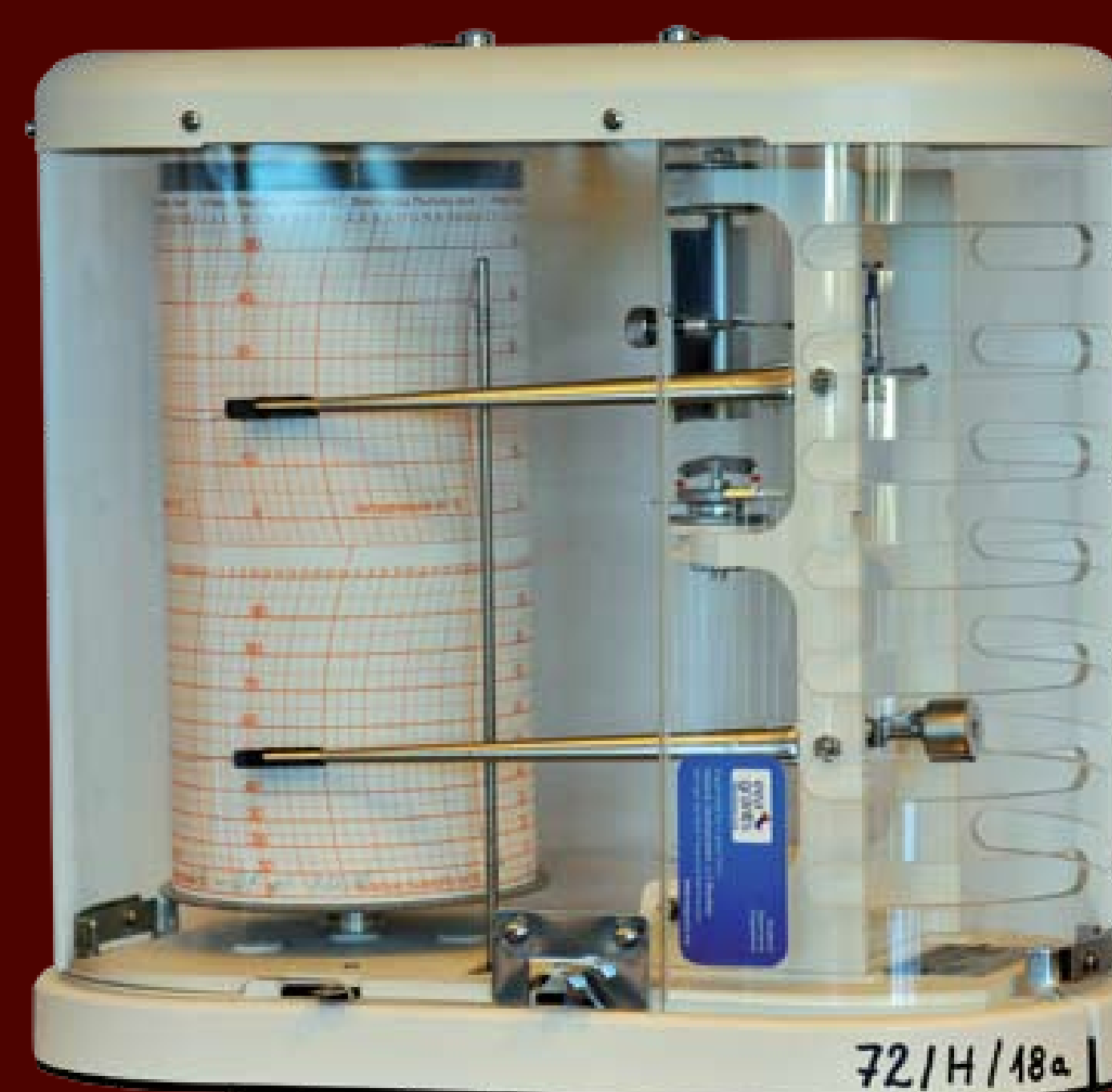
Urządzenia do kontroli warunków klimatycznych (na zdjęciach widoczne są termohigrograf oraz wizualizacja pomiarów pochodzących z zainstalowanego w Książnicy Cieszyńskiej elektronicznego systemu monitoringu temperatury i wilgotności powietrza).
