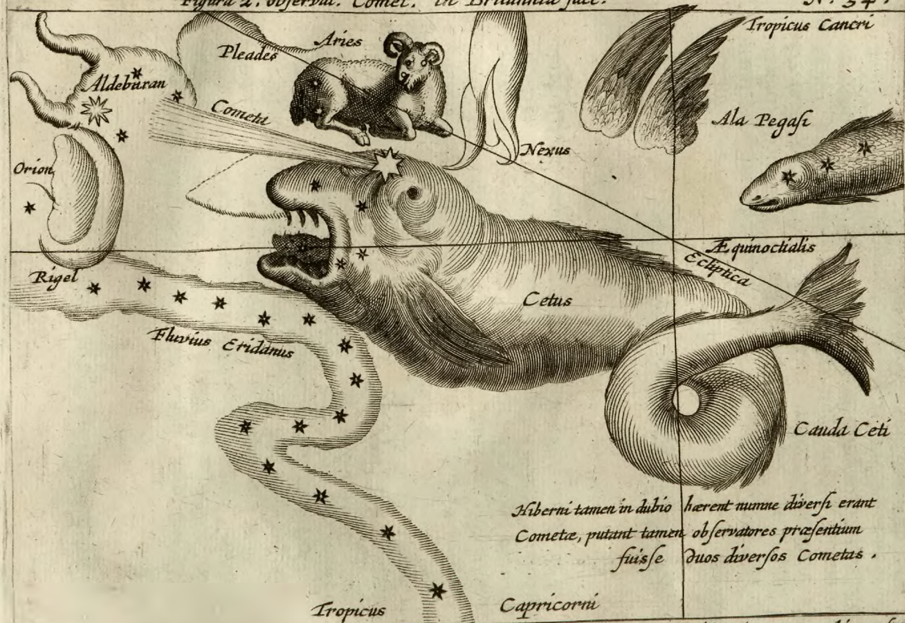
Figura 2. observat. Comet. in Britannia fact.
