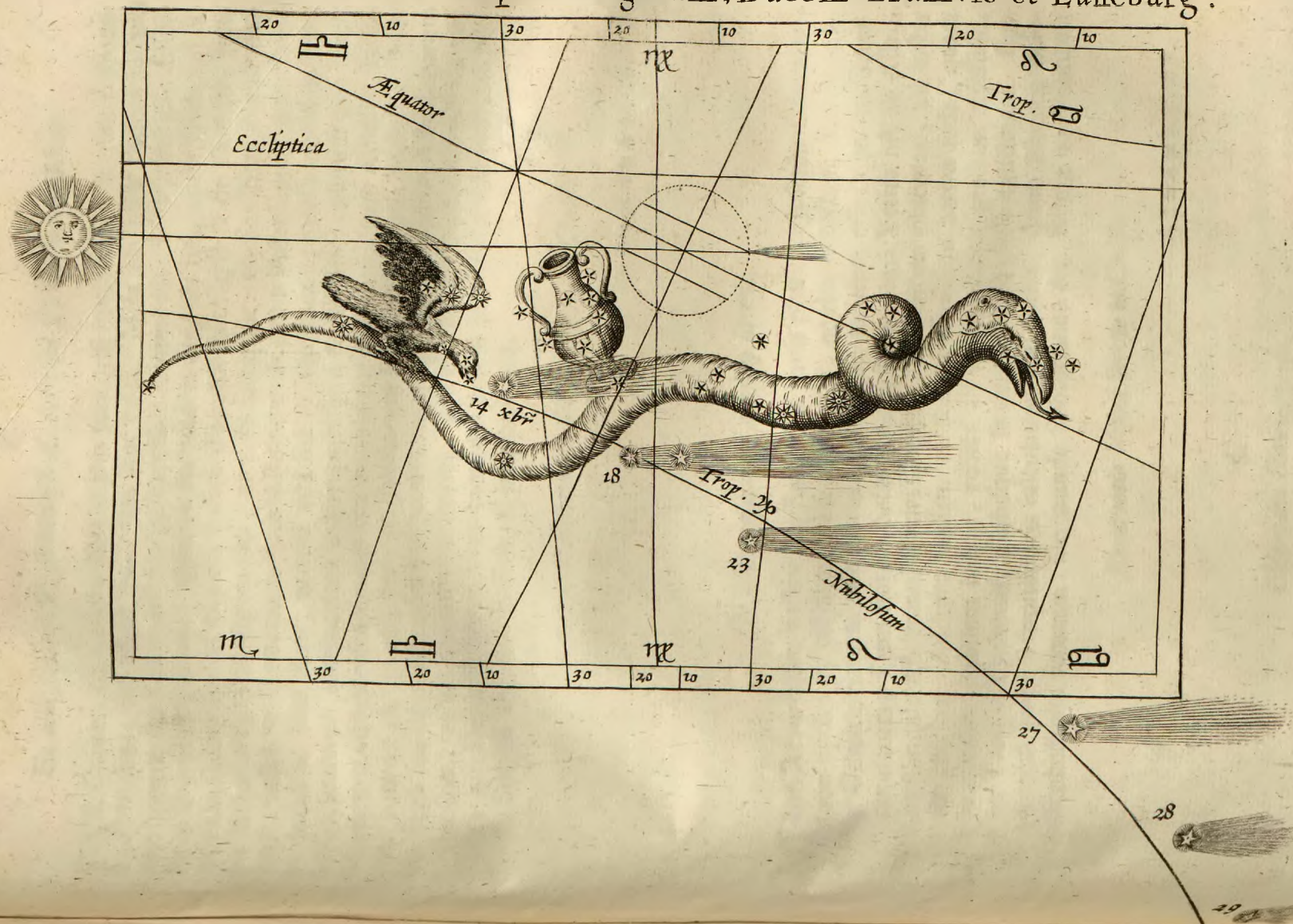
Figura 2. Observat. cometicar. a R. P. A. KIRCHERO. ad communicat. R. P. C. SCHOTTJ. Iter Cometæ Anni 1664 a 14. Decemb. usque ad 30. Romæ observatum Ad Serenissimum Principem Augustum, Ducem Brunsvic. et Luneburg.
