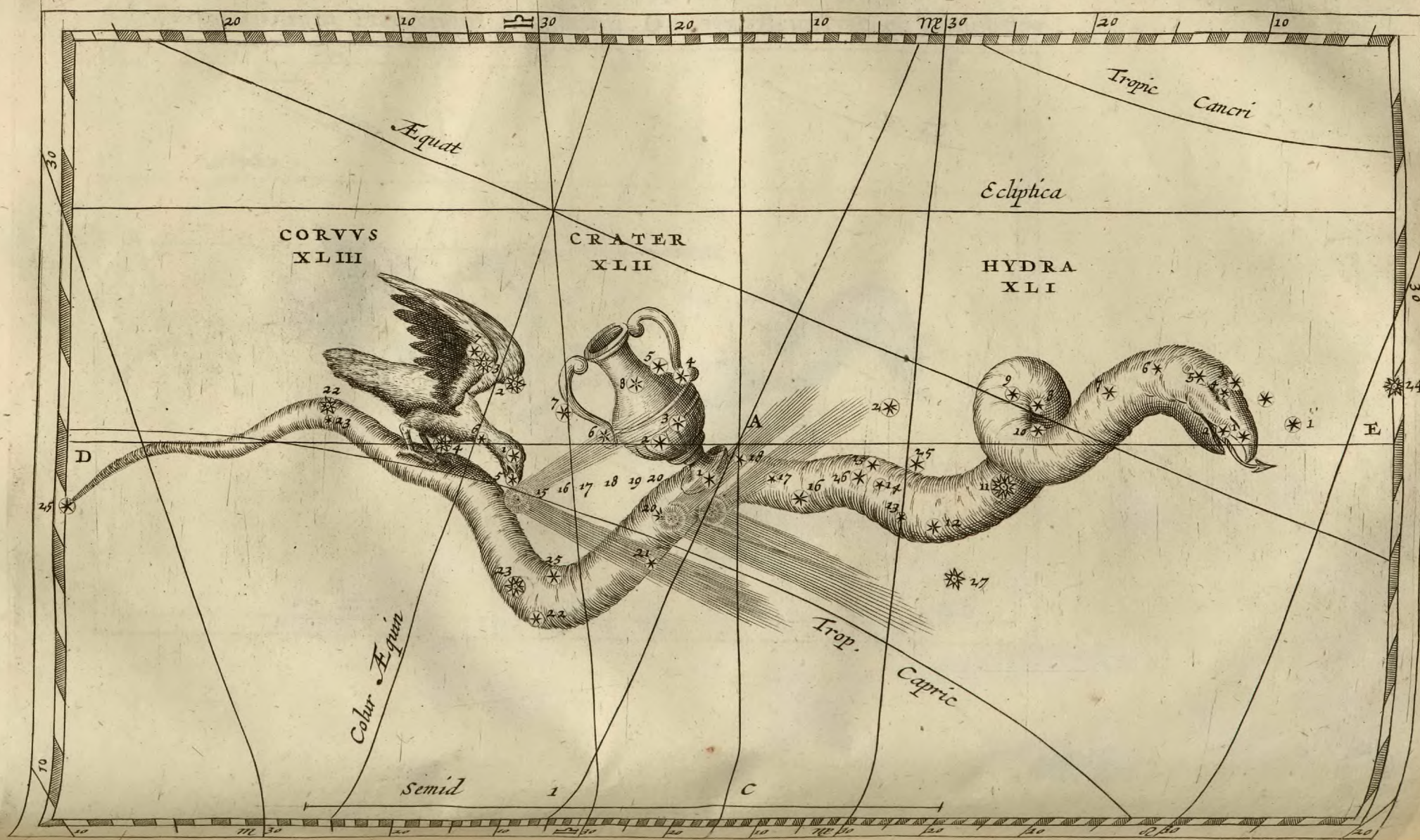
N. XVI. Figura I observat Cometar. Romæ factar ad Communicat R.P.A. Kircheri pertinens.
