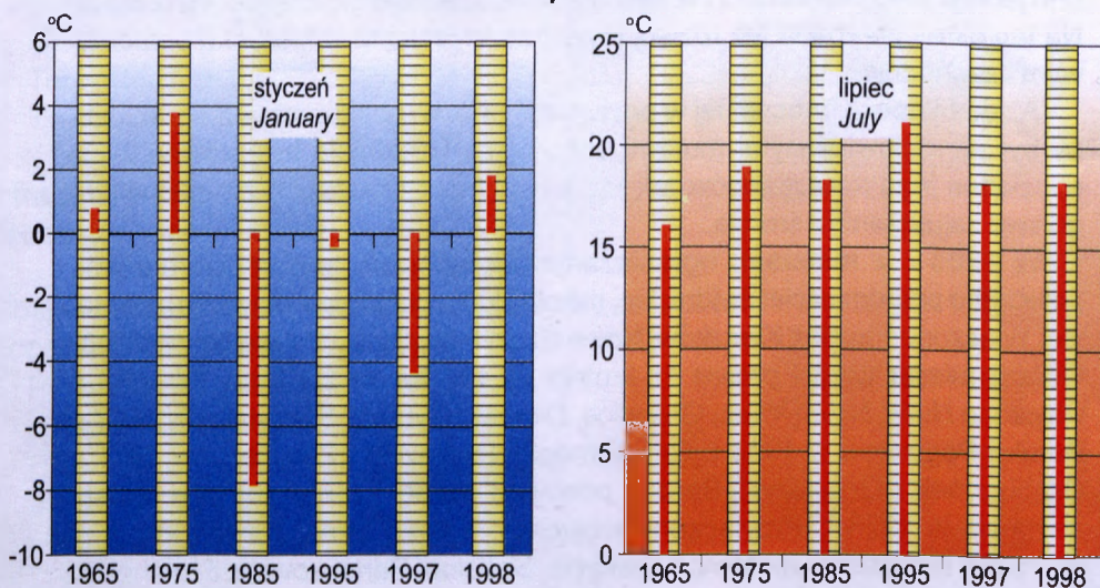
Temperatury powietrza Air temperatures
