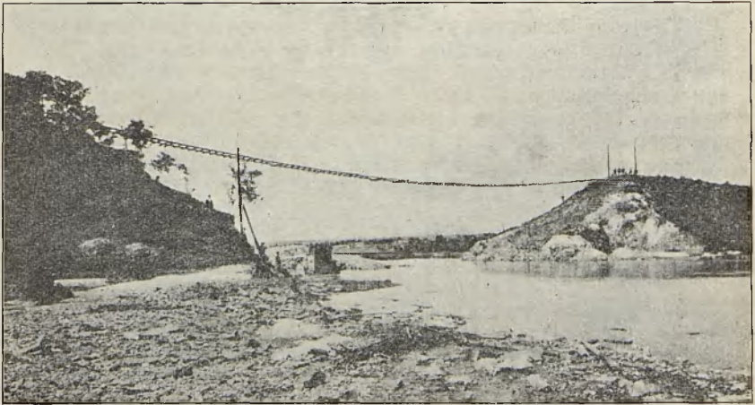
Der Bahndammbruch bei Dt. Rasselwitz im Jahre 1903.
