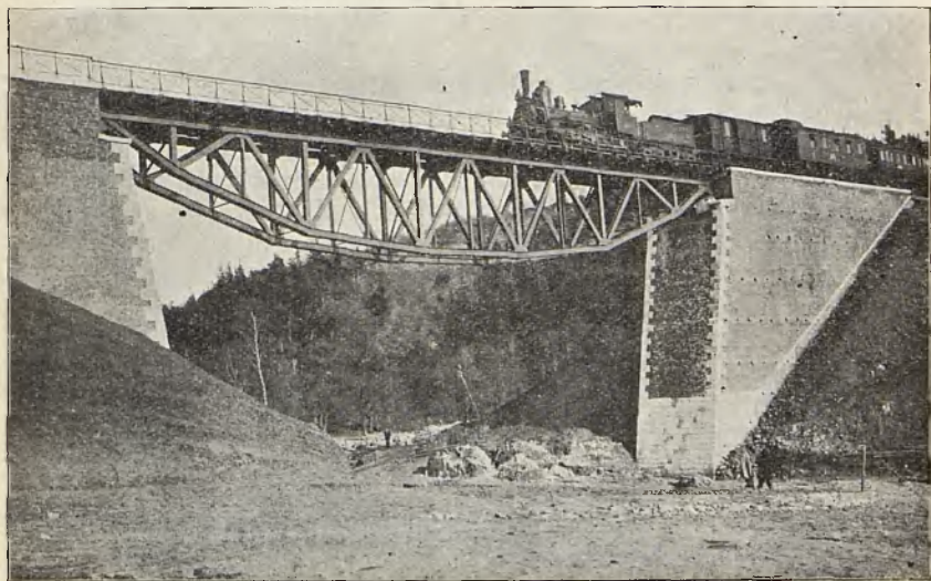
Neue Eisenbahnbrücke bei Dt. Rasselwik.
