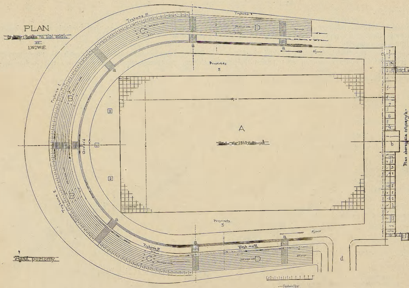
Boisko złotowe. — Rzut poziomy.
