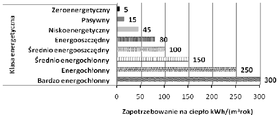
Rys. 1. Wskaźnik sezonowego zapotrzebowania na ciepło dla różnych klas budynków wg Stowarzyszenia na Rzecz Zrównoważonego Rozwoju [3]
