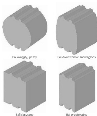
Rys. 1. Rodzaje bali pełnych [2]
