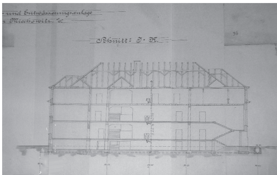
5. Projekt systemu kanalizacyjno-wodociągowego z 1913 roku (nie uwzględnia systemu wietzenia z charakterystyczną wieżyczką)-przekrój.
