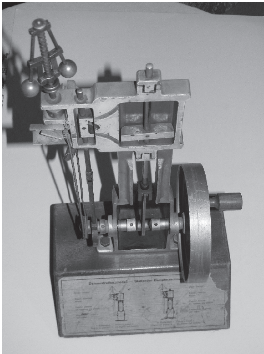
12. Oryginalny model – przekrój maszyny parowej z lat 20. zakupiony w Lipsku
