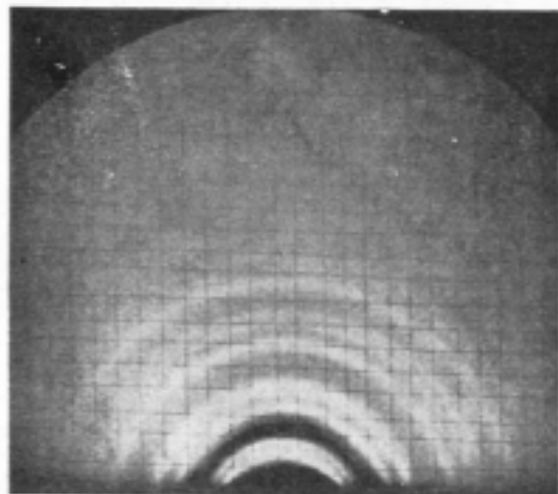
Rys. 3. Pierścienie dyfrakcyjne, wywołane przez elektrony, odbite od małej blaszki złotej (G. P. Thomson).
