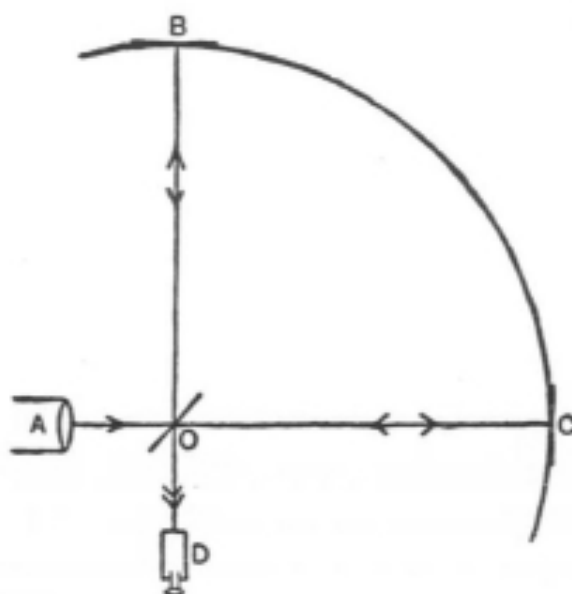
Rys. 1. Wykres, ilustrujący doświadczenie Michelsona-Morley'a.
