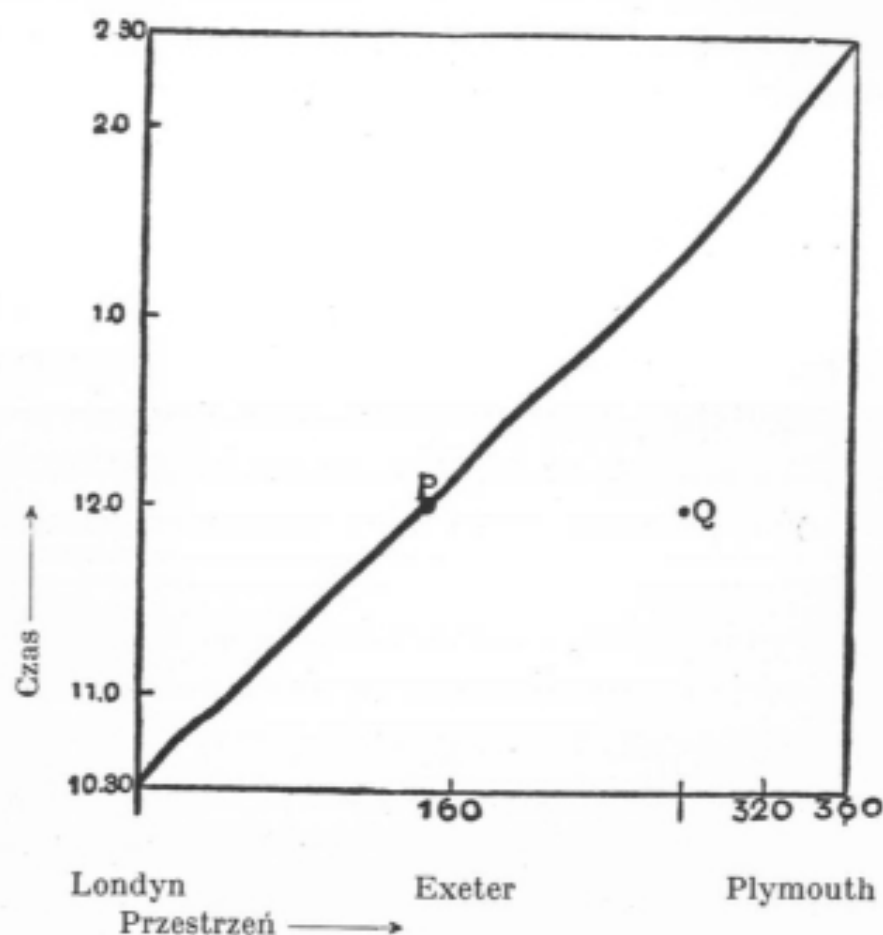
Rys. 2. Wykres, ilustrujący bieg pociągu w czasie i przestrzeni.
