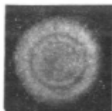
Rys. 1. Pierścienie dyfrakcyjne, wywołane przez światło, przechodzące przez mały otwór w ekranie (N. R. Fowler).
