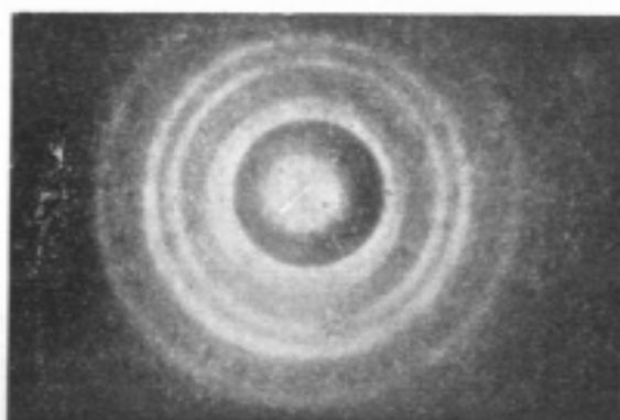
Rys. 2. Pierścienie dyfrakcyjne, wywołane przez elektrony, przechodzące przez małą błonkę ze złota (G. P. Thomson).
