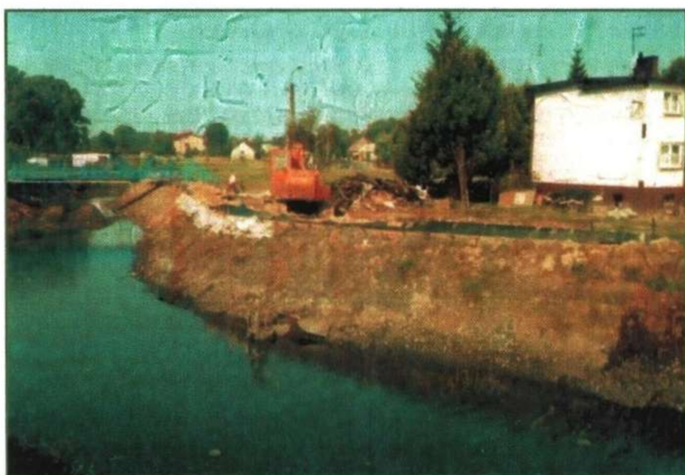
Poszerzanie koryta Pszczynki na dolnej wsi
