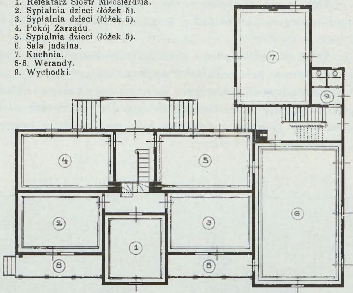
Plan parteru.
