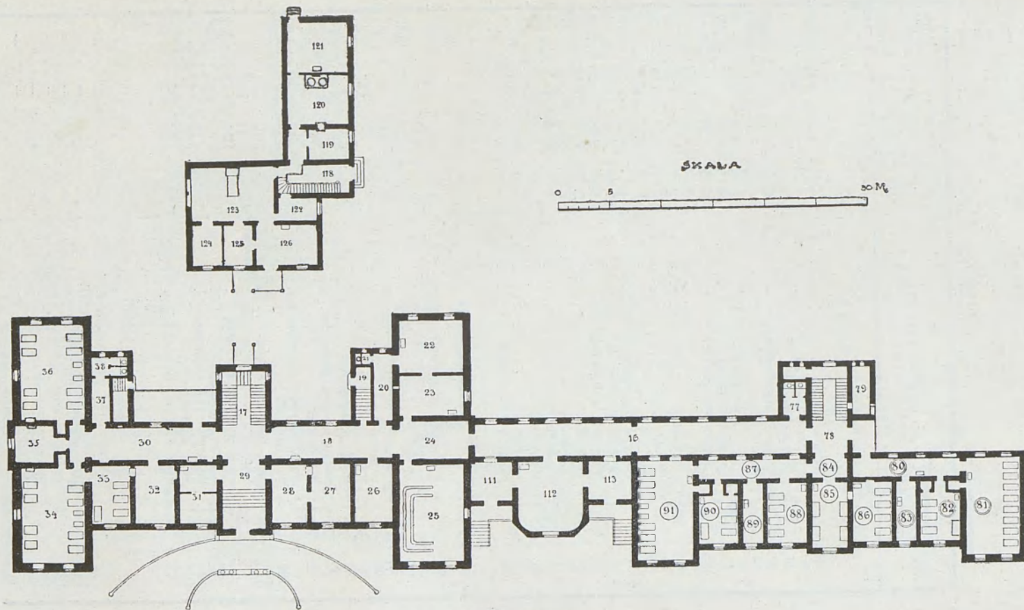
Plan parteru.
