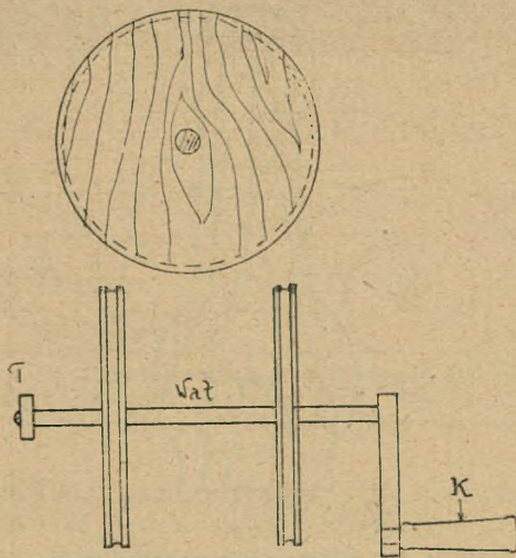
Rys. 11. Napęd. T = tarczka nie pozwalająca na wysuwanie się wału, K = korba
