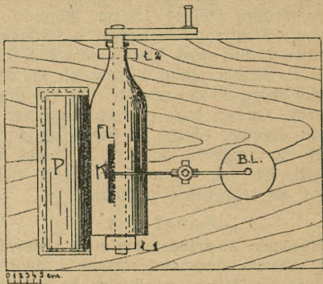
Rys. 3. Widok maszyny Wintery z góry.
