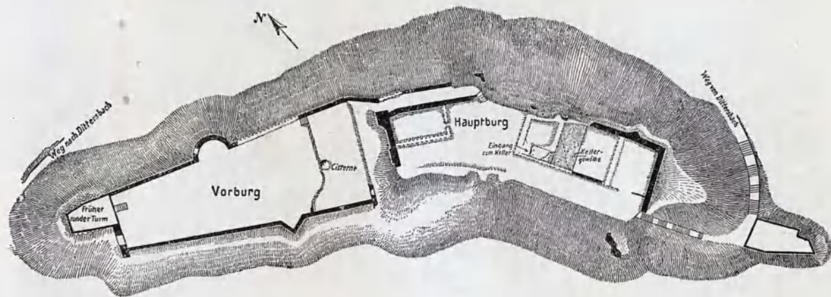
Plan der Burg Neuhaus.
