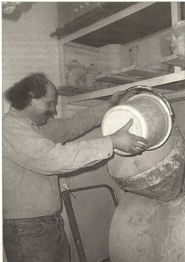
Młyn kulowy w środku wykonany z porcelany. Młyn zasypuje się różnego rodzaju gatunkami glin, kwarcem, skaleniem i wlewa minimalną ilość wody. Dodaje się elektrolity i porcelitowa masa gotowa
