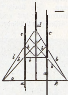
Dachkonstruktion in Holtaalen (Norwegen) in Wang (Schlesien). a Mittelsäulen, b Dachsparren und Giebtühl, c Giebtühl des Dachreiters, d Mastbaum des Dachreiters, e Decke des Schiffes.
