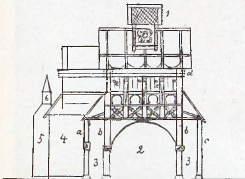
Längsdurchschnitt einer vierstüligen Stabkirche (Lomen) mit Dachreiter (Hurum) aber ohne Gangangang.
