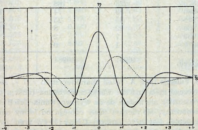
Ryc. 9. Funkcje \varphi_3 (linia ciągła) i \varphi_4 (linia przerywana). Na osi odciętych zaznaczone wartości zmiennej niezależnej \xi . (Według Charliera).
