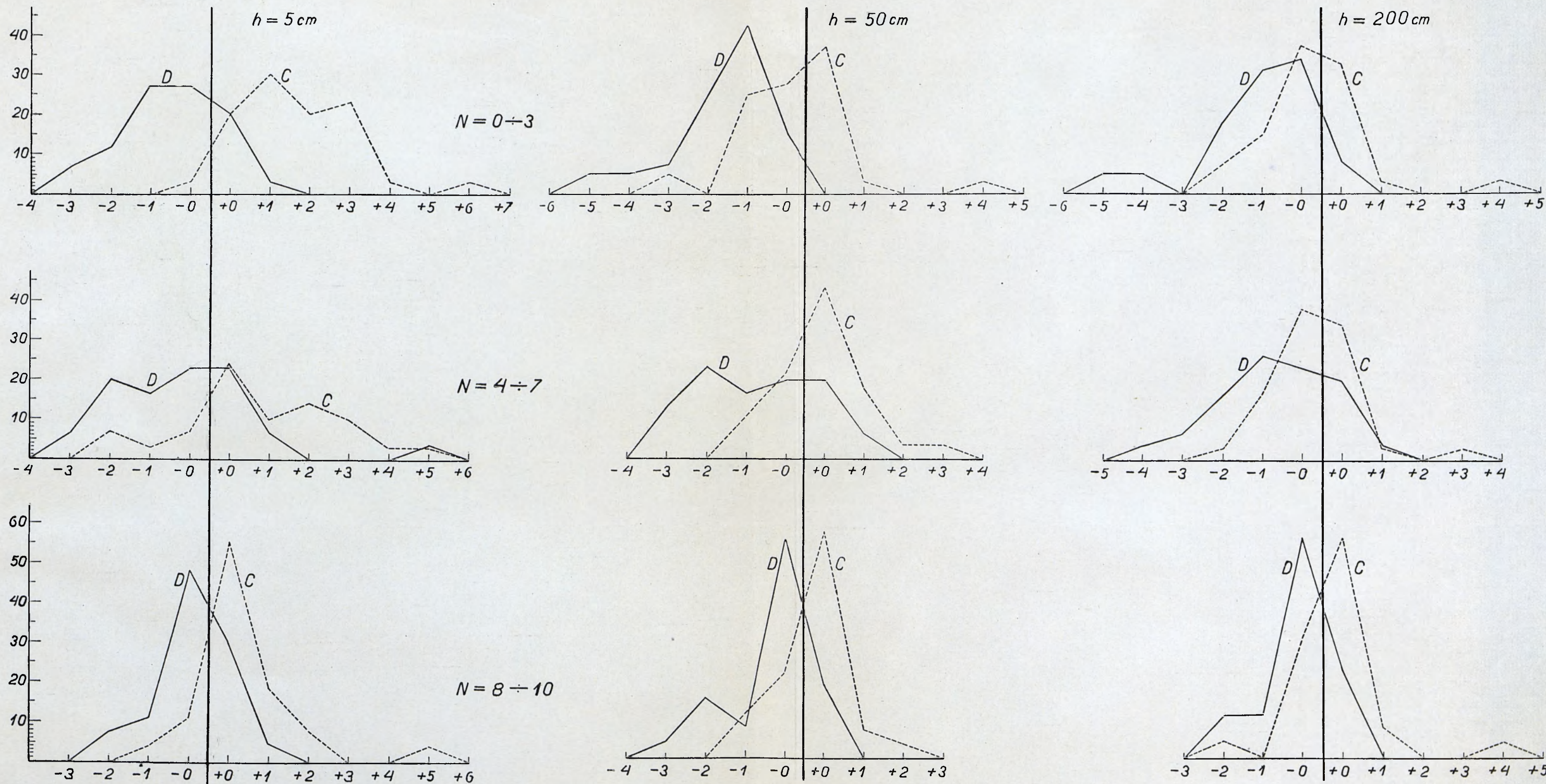
Ryc. 2. Częstość różnic w temperaturach submaksymalnych powietrza między stanowiskami C i D a stanowiskiem A (w %). N oznacza zachmurzenie, h — poziom nad powierzchnią gruntu.
