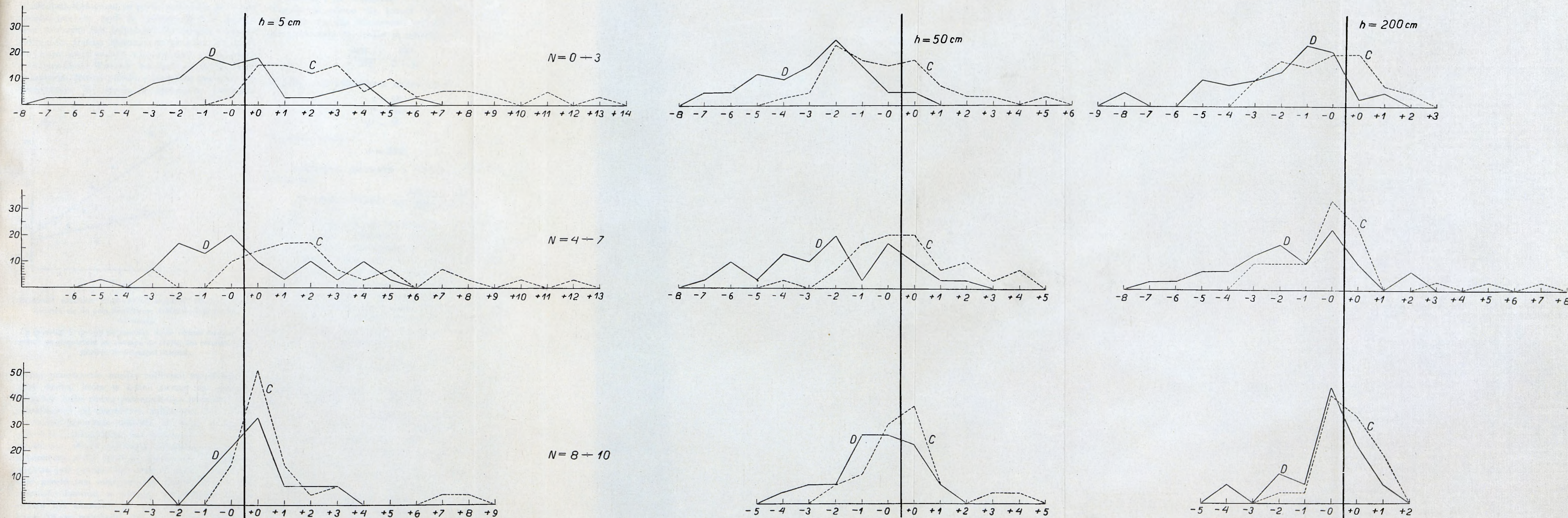
Ryc. 7. Częstość różnic we wskaźniku parowania między stanowiskami C i D a stanowiskiem A (w ‰). N oznacza zachmurzenie, h — poziom nad powierzchnią gruntu. Fréquence des différences entre les indices d'évaporation des stations C et D et ceux de la station A (en ‰). N signifie la nébulosité, h — le niveau au-dessus du sol.
