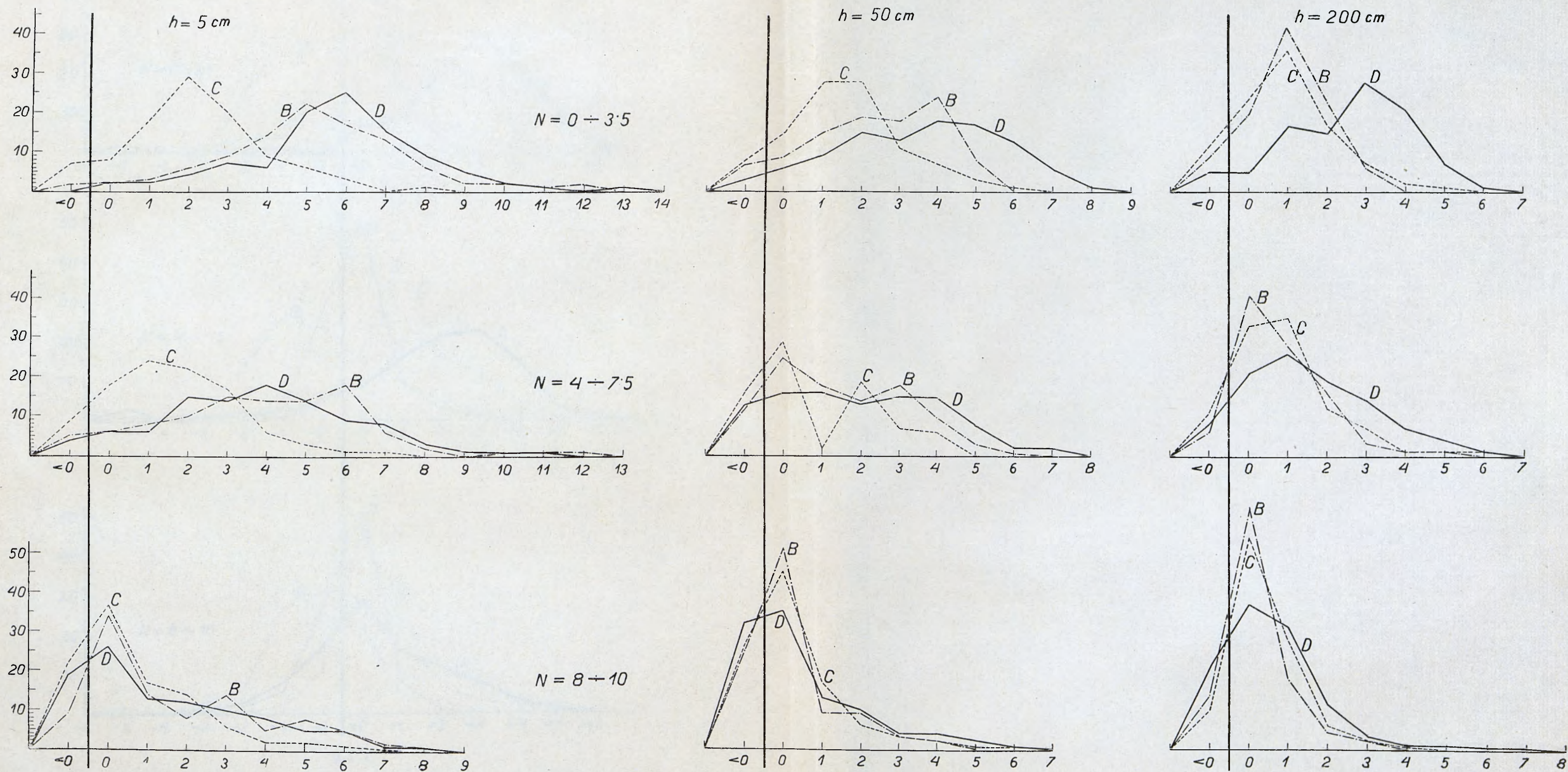
Ryc. 3. Częstość różnic w temperaturach minimalnych powietrza między stanowiskami B, C i D a stanowiskiem A (w ‰). N oznacza zachmurzenie, h — poziom nad powierzchnią gruntu.
