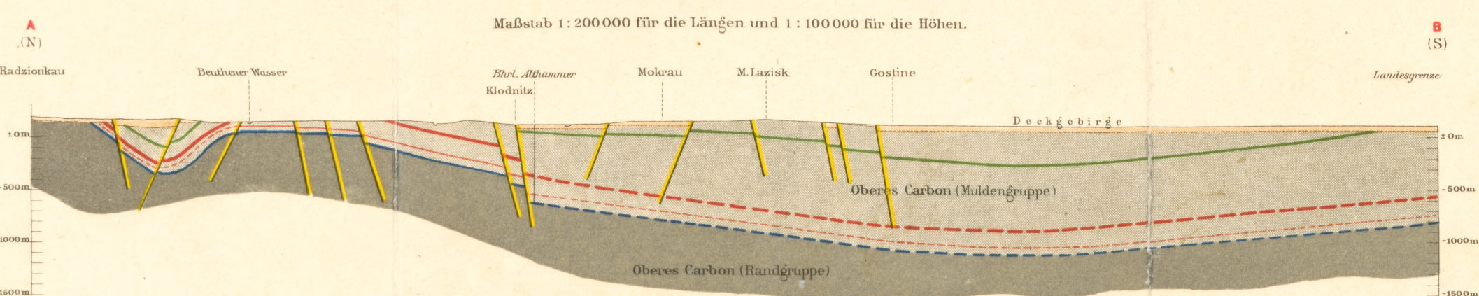
Profil A-B.
