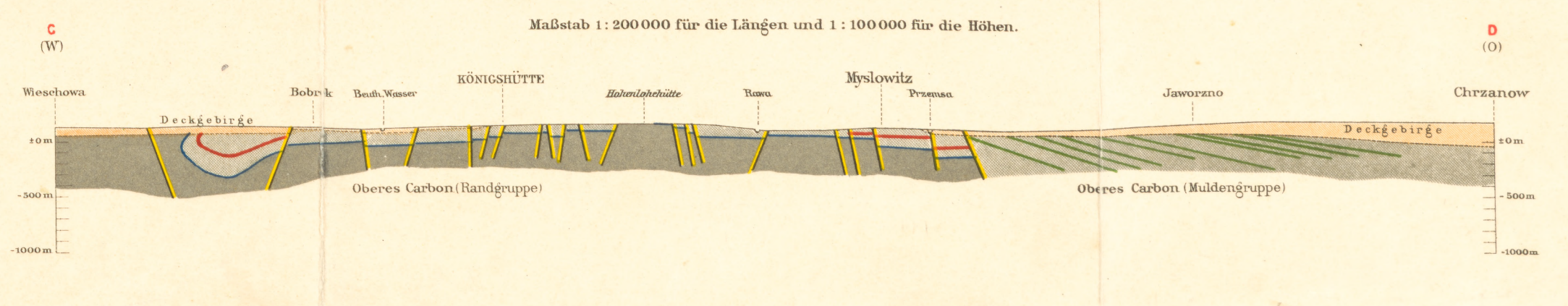
Profil C-D.
