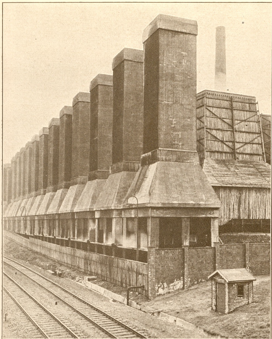
Kühltürme der Elektrizitätszentrale Chorzow
