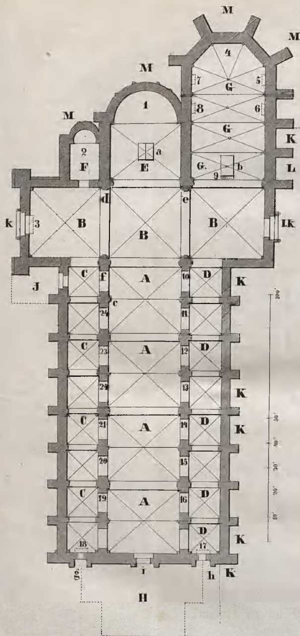
Grundriss der Klosterkirche in Trebnitz.
