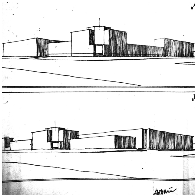
Fot. 6. Projekt wstępny Ośrodka Wychowania Fizycznego przy ul. Raciborskiej w Katowicach (dwie alternatywy); proj. Fryderyk Daun, 12 IV 1934 r. (AUMK, zbiór akt bez inwentarza)
