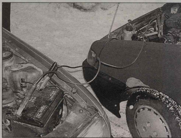
Przy podłączaniu kabli ważne jest zachowanie właściwej kolejności. Pomyłka grozi awarią
