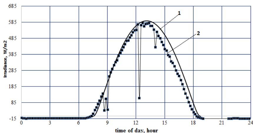
Рис. 2. Расчет и сравнение с экспериментом интенсивности солнечного излучения 28.09.2017, г. Киев: 1 - модель ASHRAE 01; 2 - результаты эксперимента г. Киев
