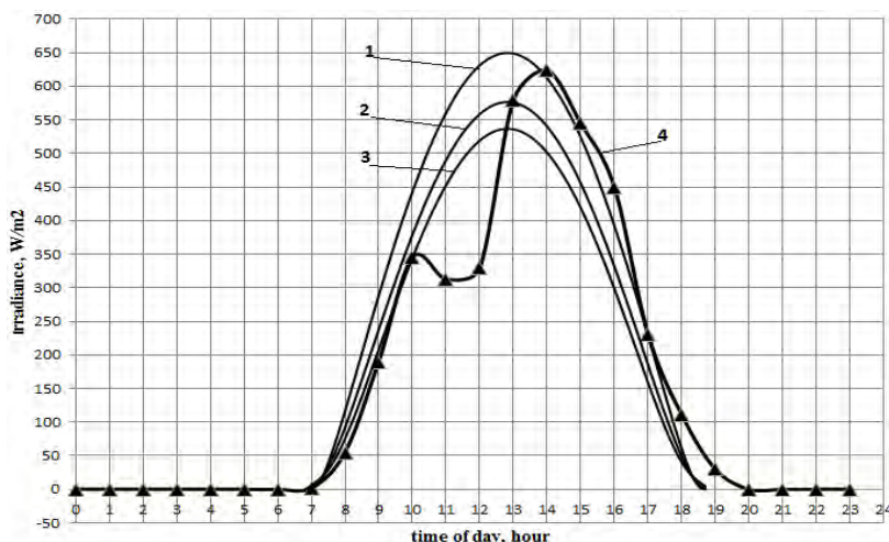
Рис. 1. Расчет и сравнение с экспериментом интенсивности солнечного излучения в марте (весеннее равноденствие, для Одессы: 1 - модель ASHRAE 01; 2 - модель ASHRAE 09; 3 - модель Hottel 1976 г., 4 (▲-точки) - результаты эксперимента в Одессе (выпадение точек в 11 и в 12 часов объясняется появлением облачности)
