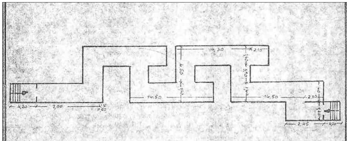
Przekrój szczeliny przeciwlotniczej na Placu Żeromskiego
