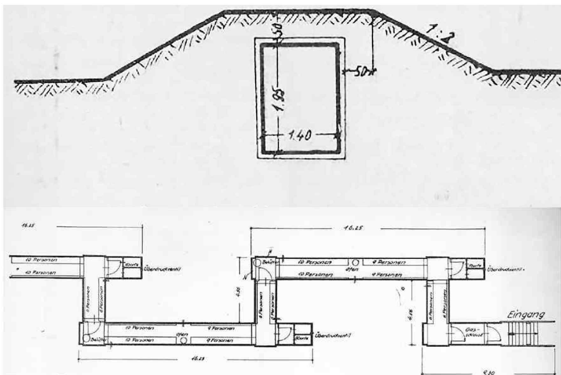
Projekt budowy szczelin przeciwlotniczych według wytycznych z marca 1943 roku
