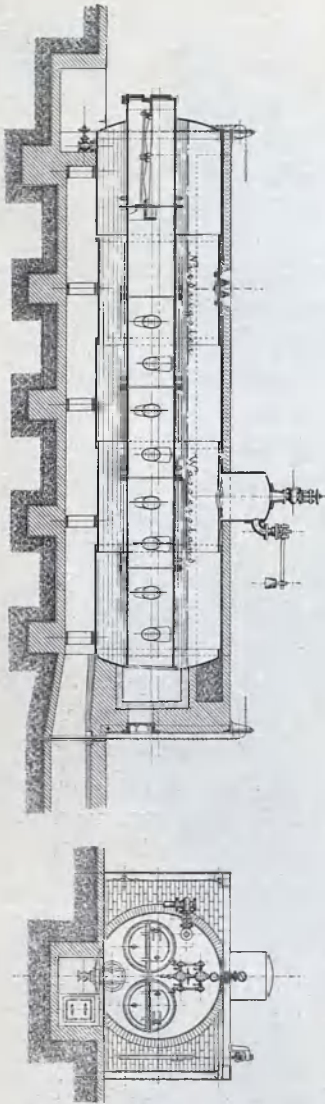
Zweiflammenrohrkessel mit Gallowayrohren.
