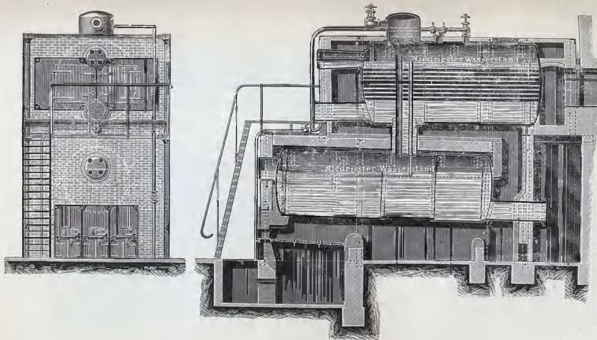
Kombinierter Dampfkessel.
