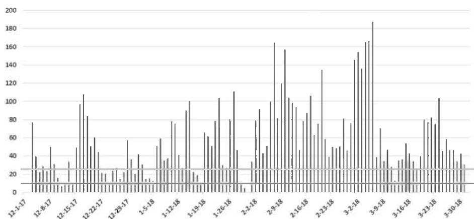
PM2,5 - średnia dzienna – Bystra, ul. Jasna 1.12.2017 - 31.03.2018
