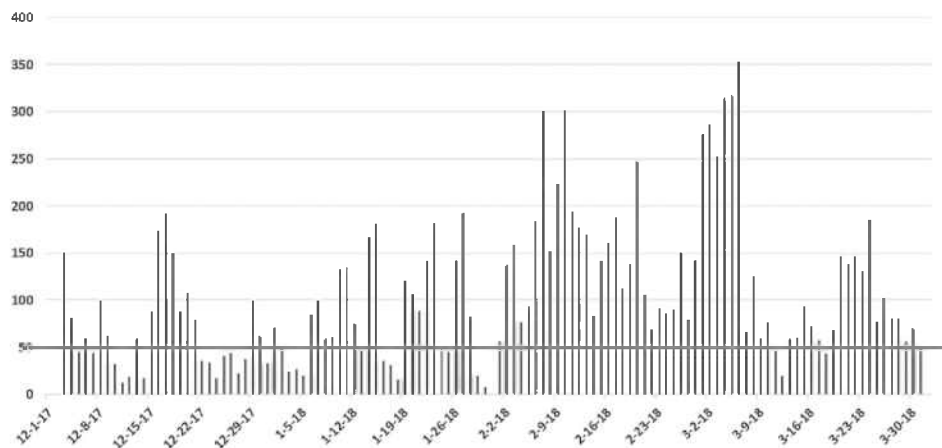
PM10 - średnia dzienna – Bystra, ul. Jasna 1.12.2017 - 31.03.2018
