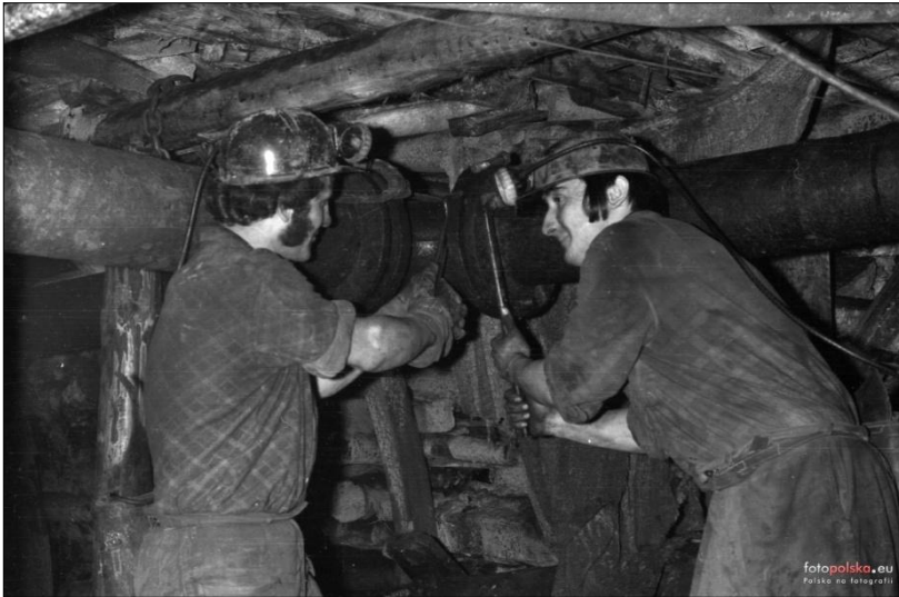
Montaż rurociągu doprowadzającego powietrze, tzw. lutfociągu. .zdj. ilustracyjne z Kopalni Węgla Kamiennego Matylda, źródło: Fotopolska-Eu, autor: Eugen+
