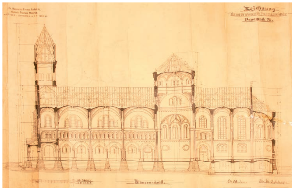
Przekrój podłużny założenia kościoła panewnickiego projektu Mansuetusa Fromma
