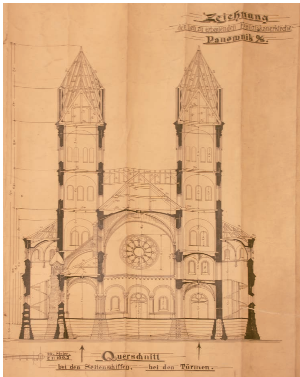
Przekrój poprzeczny założenia kościoła panewnickiego projektu Mansuetusa Fromma
