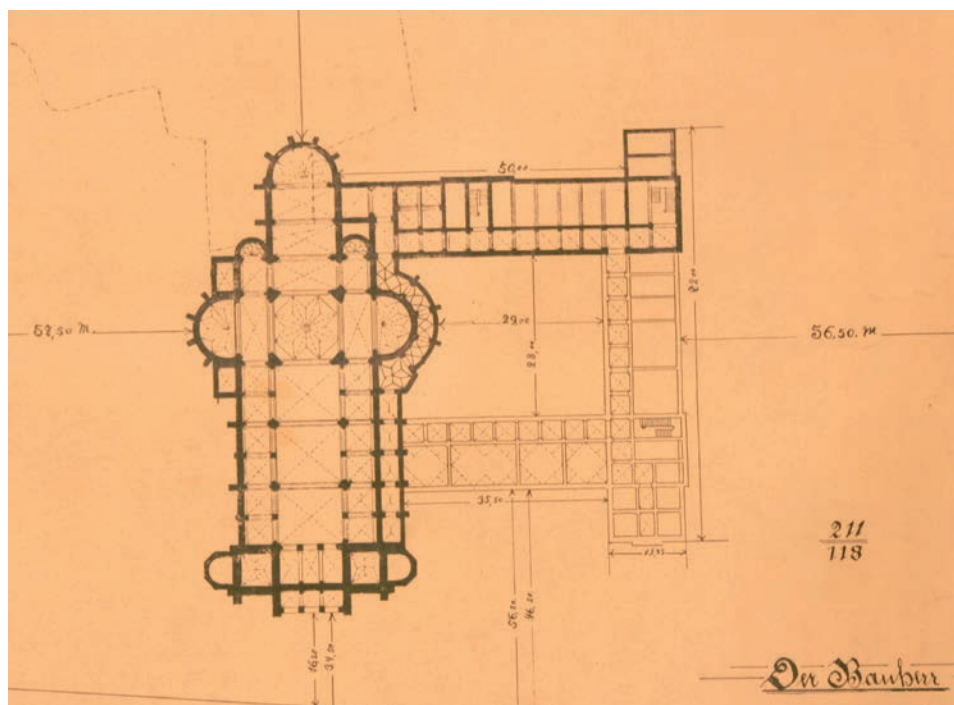
Rzut założenia kościoła i klasztoru panewnickiego projektu Mansuetusa Fromma
