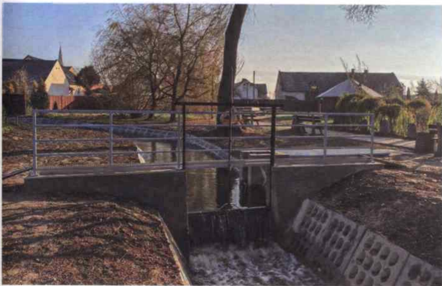
Prace na cieku „Obrowiecki” polegały m.in. na wykonaniu mnicha piętrząco – zrzutowego
