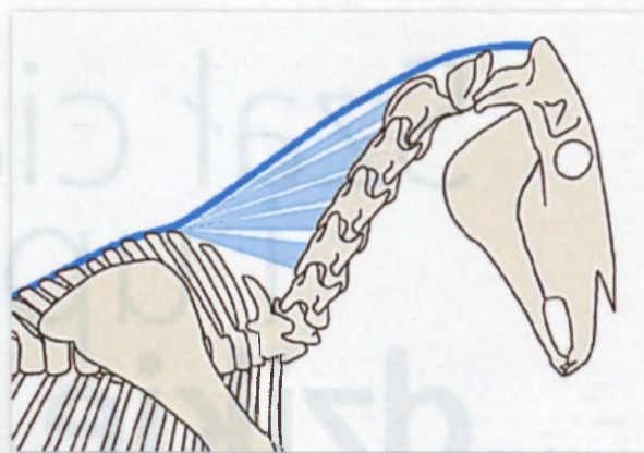
Rys. 2. Więzadło karkowe
