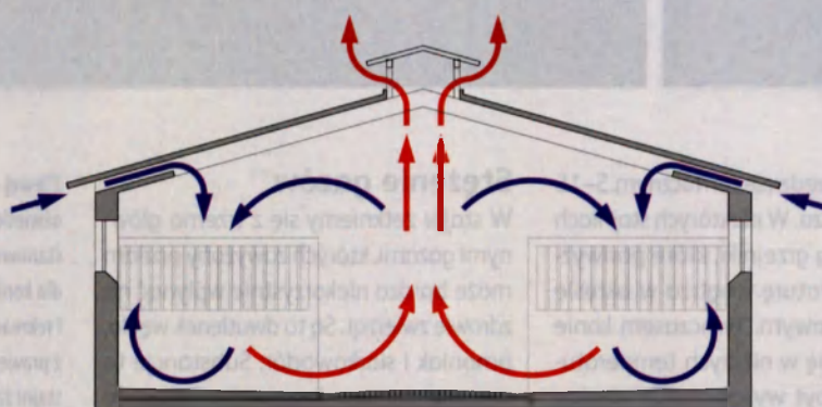
WENTYLACJA GRAWITACYJNA PRZEZ KALENICĘ
