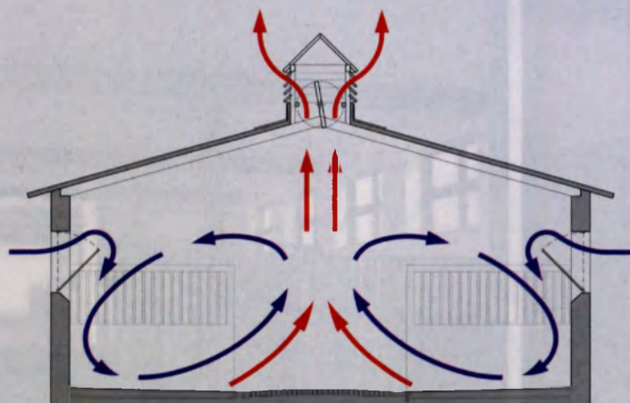
WENTYLACJA KOMINOWA
