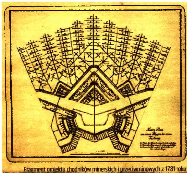
Poza obrębem murów obronnych budowano dziesiątki, różnej wielkości, podziemnych chodników minerskich
