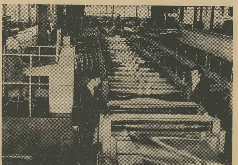
Tu produkowane są osłony. Roboty te wykonuje brygada walcownicza: mistrz Franciszek GAJOWSKI, mechanik utrzymania ruchu Jan MATEJCZYK, obsługa pulpitu sterowniczego Krystyna KRASON, oraz Urszula KURJANOWICZ i Janina ZAK.
