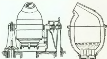
Konverter
