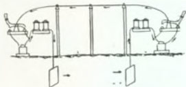
Telegraphie, Stromlauf zwischen zwei Morse- stationen
