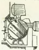
Tenbrinkfeuerung mit schrägem Rost
