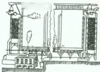
Bleikammern u. Glovertürme
