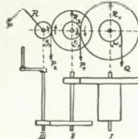
Räderwerk
