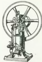
Viertakt-Gasmotor
