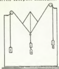
Kraftparallelogramm
