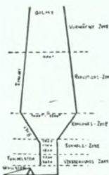
Hochofen-Anlage
