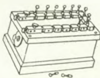
Stöpsel-Rheostat
