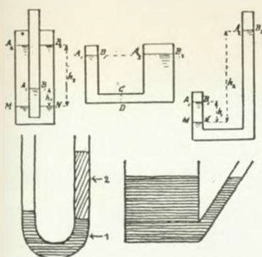
kommunizierende Röhren
