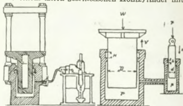
Hydraulische Pressen
