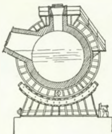
Rohreisenmischer
