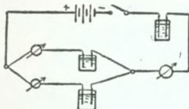
Faradismus
