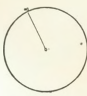
Halbmesser
