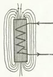
Kraftlinien im Magnetfeld
