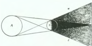
Kern- u. Halbschatten
