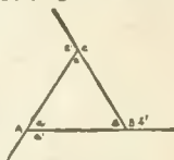
Außenwinkel
