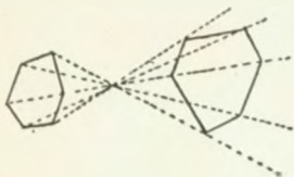
Ähnlichkeit (Math.)
