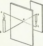
Entstehung eines Bildes durch ein kleines Loch
