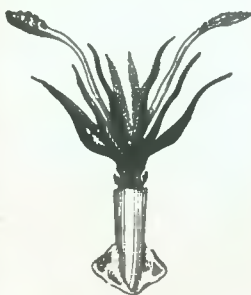
Zehnnarmer Tintenfisch
