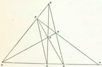
Harmonische Teilung
