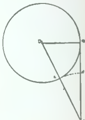
Goldener Schnitt
