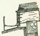
Holzzementdach
