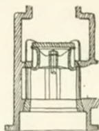
Doppelstz-Ventil
