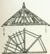
Zeltdach
