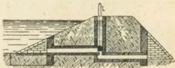
Abblaktationsvorrichtung für einen Teich
