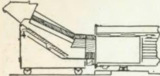
Treppenrost-Vorfeuerung
