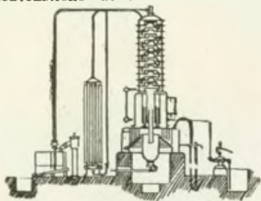
Ammoniak-Darstellung
