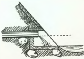
Ausmündung eines Sammeldrains
