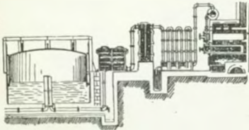
Steinkohlen-Destillation
