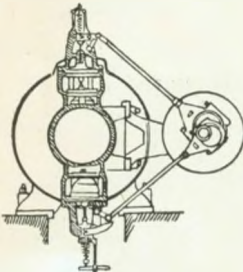
Dampfzylinder mit Ventilsteuerung
