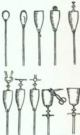
Herstellung eines Kelchglases
