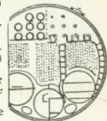
Zylinderkessel (Querschnitt)
