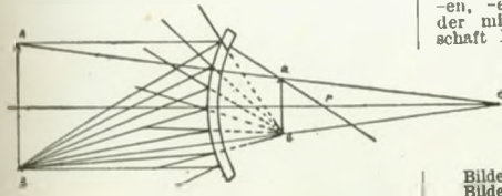
Entstehung eines Bildes bei einem Konvexspiegel
