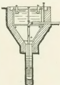
Klärbrunnen
