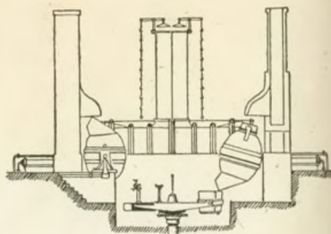
Bessemer-Anlage
