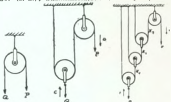
Einfache u. zusammengesetzte Rollen
