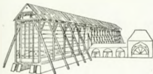
Gradierverk
