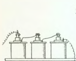
Bunsen'sche Elemente
