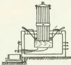
Aluminium: Heroult-Apparat
