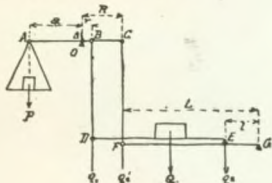
Brücken-Wage (Schema)
