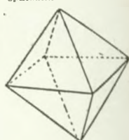
Oktaeder
