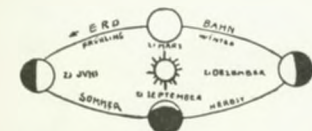
Sonnenjahr (Lauf der Erde um die Sonne)
