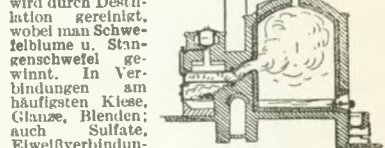
Schwefeldarstellung
