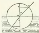
Brechungsgesetz
