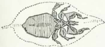
Wandelndes Blatt
