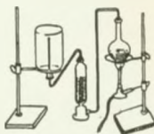
Ammoniak-Darstellung
