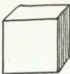
Hexaeder
