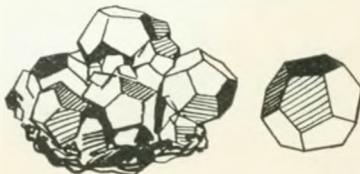
Eisenkies
