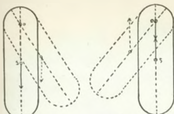
Labiles Gleichgewicht
