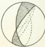
Sphärisches Zweieck u. Dreieck
