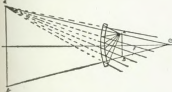
Entstehung eines Bildes bei einem Hohlspiegel
