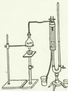
Avogadros Gesetz
