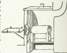
Kalium-Darstellung
