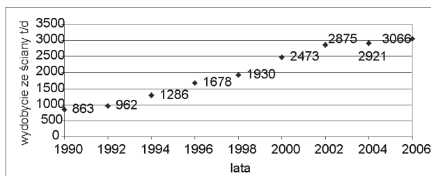
Rys. 2. Wzrost wydobywania ze ścian
