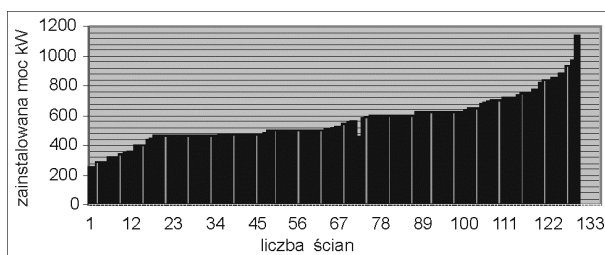
Rys.4. Rozkład zainstalowanej mocy w kombajnach
