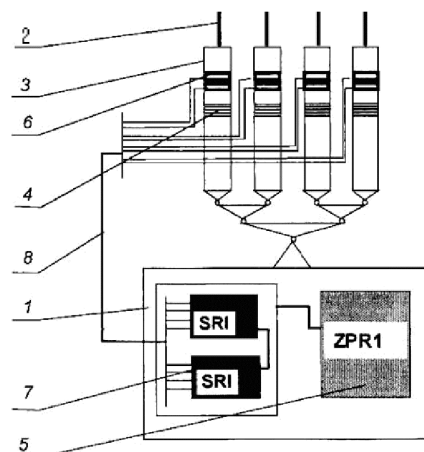
Rys.6. Schemat toru pomiarowego i rozmieszczenia czujników siły
