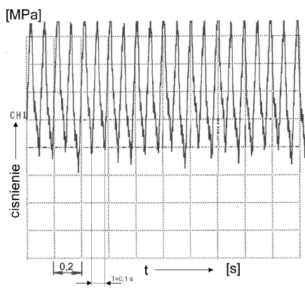
Rys.8. Przebieg pulsacji ciśnienia w układzie hydraulicznym. Częstotliwość wymuszeń pulsacji ciśnienia wzбудnikiem impulsu f_w = 10 Hz. Ciśnienie tłoczenia p_t = 16 , CH1 – układ bez tłumika, CH2 – układ z tłumikiem
