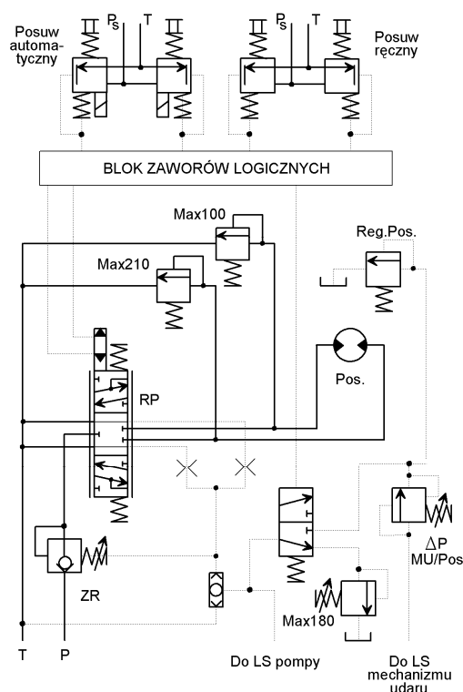
Rys.8. Funkcjonowanie układu zasilania i sterowania mechanizmu obrotów hydraulicznej wiertarki obrotowo-udarowej [11]
