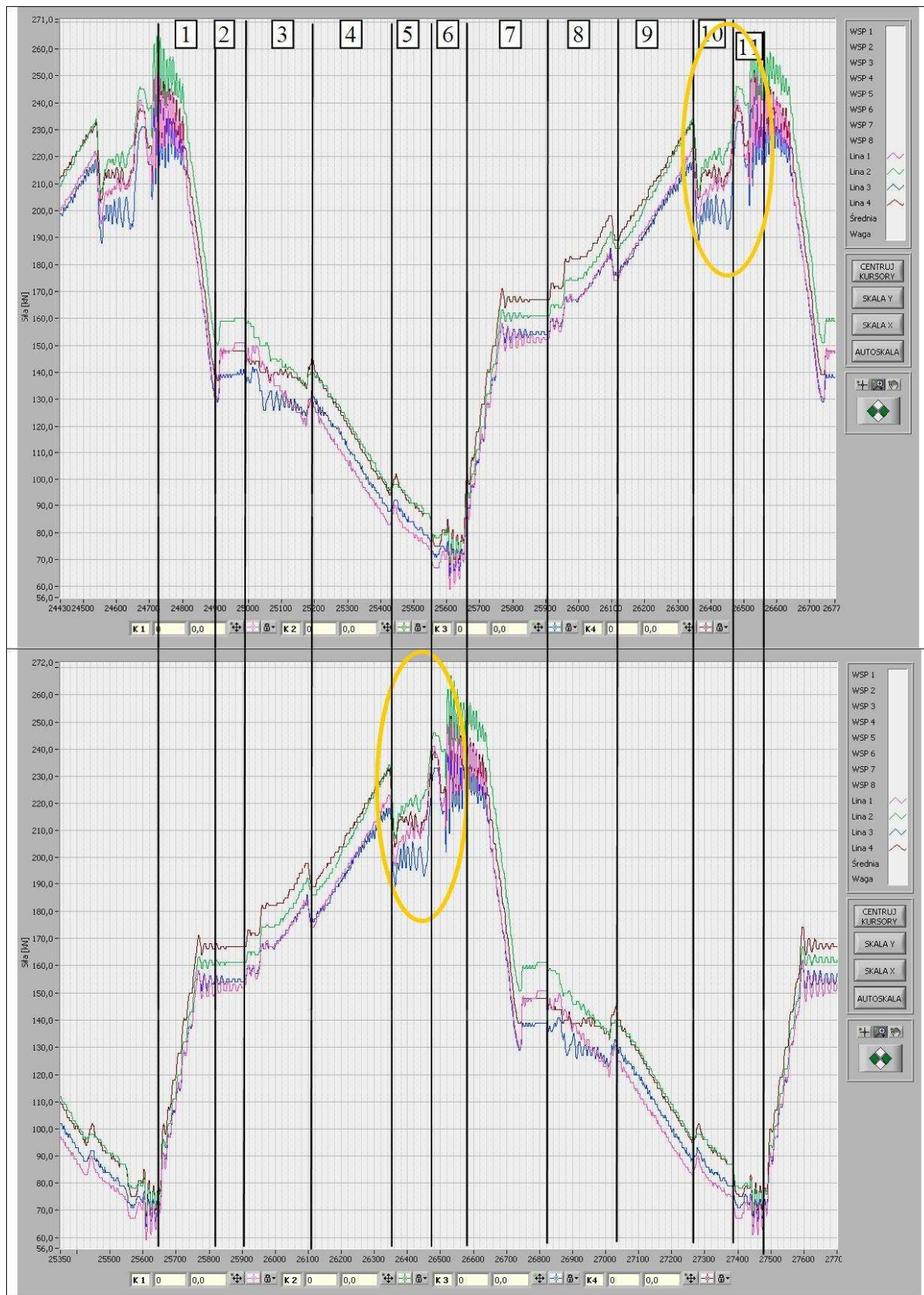
Rys.6. Zarejestrowane rozkłady obciążeń w linach czterolinowego wyciągu szybowego, mierzone w łącznikach zmiennej długości obydwóch zawiesz naczyn wyciągowych
