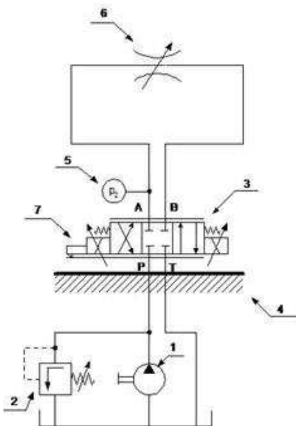
Rys.4. Schemat układu hydraulicznego badanego zaworu 1 – pompa wyporowa, 2 – zawór bezpieczeństwa, 3 – rozdzielacz proporcjonalny, 4 – drgający stół symulatora, 5 – pomiar ciśnienia, 6 – nastawny zawór dławiący jako obciążenie bezinercyjne, 7 – czujnik przemieszczenia suwaka
