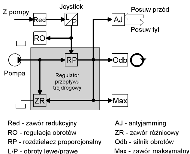
Rys.8. Funkcjonowanie układu zasilania i sterowania mechanizmu obrotów hydraulicznej wiertarki obrotowo-udarowej [11]
