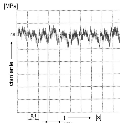
Rys.8. Przebieg pulsacji ciśnienia w układzie hydraulicznym. Częstotliwość wymuszeń pulsacji ciśnienia wzбудnikiem impulsu f_w = 10 Hz. Ciśnienie tłoczenia p_t = 16 , CH1 – układ bez tłumika, CH2 – układ z tłumikiem
