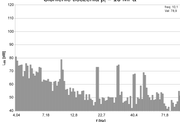
Rys.10. Analiza wąskopasmowa pulsacji ciśnienia w układzie hydraulicznym z tłumikiem czynnym. Częstotliwość wymuszeń pulsacji ciśnienia wzбудnikiem impulsów f_w = 10 Hz. Ciśnienia tłoczenia p_t = 16 MPa
