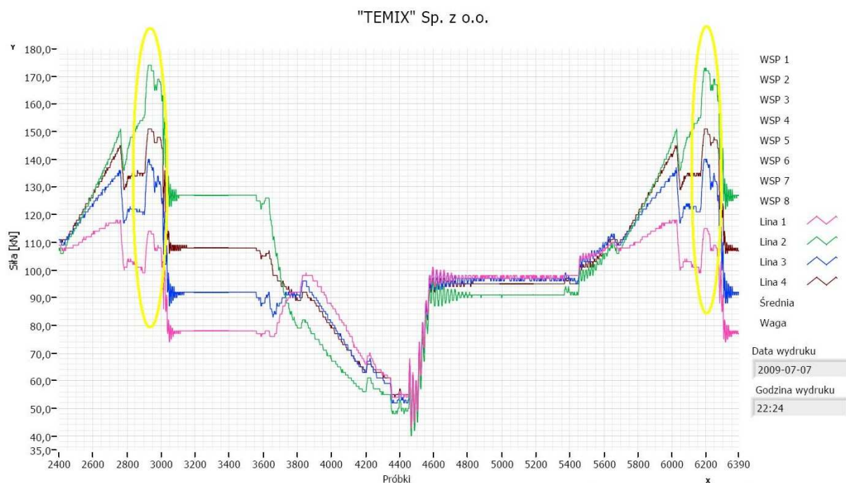
Rys.7. Zarejestrowany rozkład obciążeń w linach czterolinowego wyciągu szybowego z maszyną wyciągową umieszczoną na wieży w czasie dwóch cyklu pracy (próbki od około 3400 do 6390)
