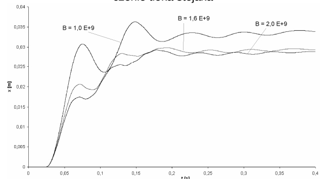
Rys.12. Wpływ modułu sprężystości na przemieszczenie tłoka stojaka
