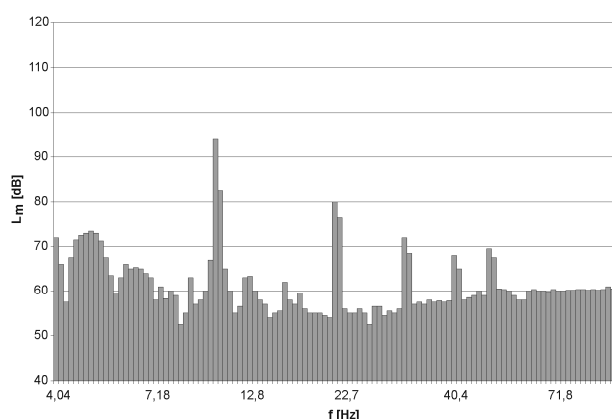
Rys.9. Analiza wąskopasmowa pulsacji ciśnienia w układzie hydraulicznym bez tłumika czynnego. Częstotliwość wymuszeń pulsacji ciśnienia wzбудnikiem impulsów f_w = 10 Hz. Ciśnienie tłoczenia p_t = 16 MPa
