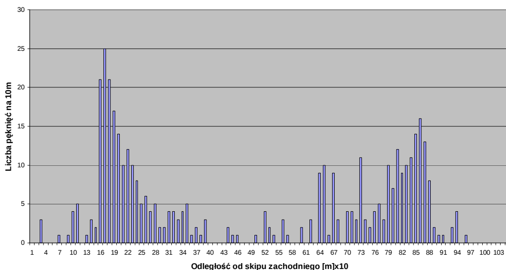
Rys. 3. Rozkład liczby pękniętych drutów wzdłuż długości liny nośnej trójkątnosplotkowej ( d = 65 \text{ mm} , l = 1050 \text{ m} ), maszyna usytuowana na zrębie [3]
