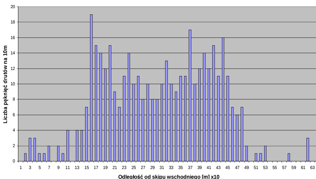
Rys.4. Rozkład liczby pękniętych drutów wzdłuż długości liny nośnej trójkątnosplotkowej ( d = 65 \text{ mm} , l = 640 \text{ m} ), maszyna usytuowana na zrębie [3]
