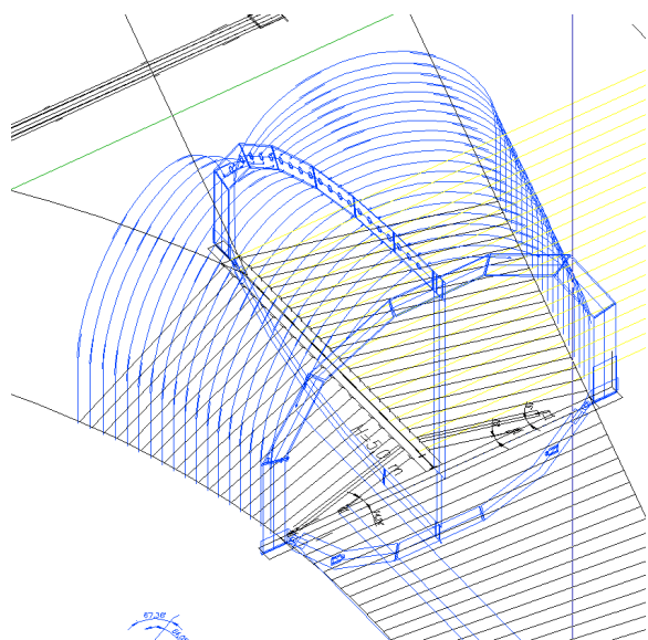
Rys.5. Modelowanie skrzyżowania dróg transportowych [2]
