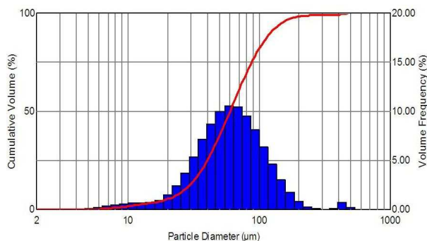
Rys.7. Przykładowy rozkład wielkości średnic cząsteczek badanej strugi powietrzno-wodnej [źródło: Sprawozdanie z badań Nr 231/BT/2009]
