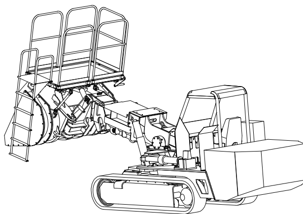
Rys.13. Uniwersalny podest roboczy [1]
