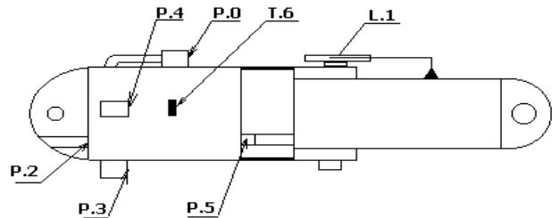
Rys.11. Schemat rozmieszczenia punktów pomiarowych na stojaku hydraulicznym [12]
