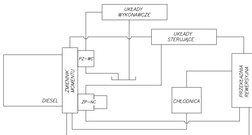
Rys.2. Hydrauliczny schemat blokowy lokomotywy typu Lds: PZ-WC – pompa zębata obwodu wysokiego ciśnienia, ZP-NC – zespół pompowy obwodu niskiego ciśnienia [13]
