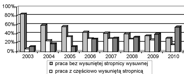
Rys.11. Rodzaj pracy sekcji skrajnych w rejonie napędu zwrotnego i wysypowego [3]
