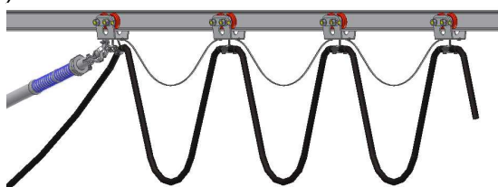
Rys.15. Urządzenie do podwieszania przewodu zasilającego: a) linowe, b) szynowe [1]
