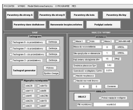
Rys.14. Oprogramowanie do wyznaczania obciążeń linopędni z uwzględnieniem zjawisk dynamicznych
