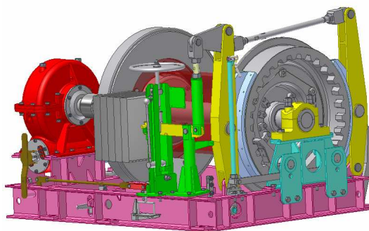
Rys.5. Model wciągarki KUBA-5
