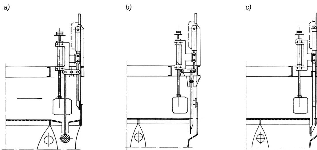
Rys.3. Przepusty produktów w osadzarkach miałowych typu KOMAG [7, 9]: a) rurowy, b) zasuwowy dźwigniowy, c) zasuwowy prostoliniowy
