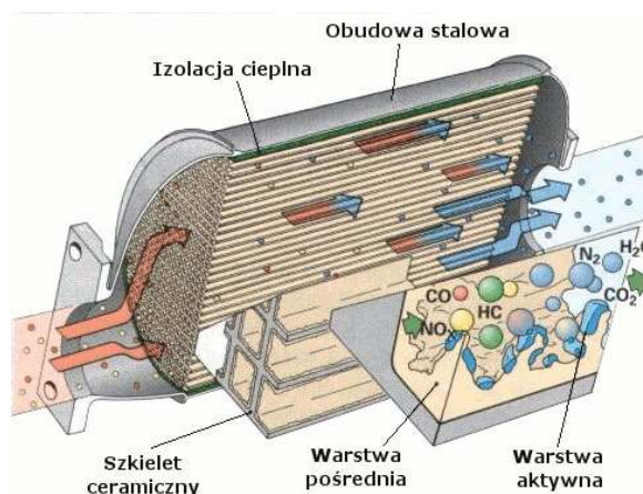
Rys.2. Budowa katalizatora oraz zachodzące w nim reakcje [1]
