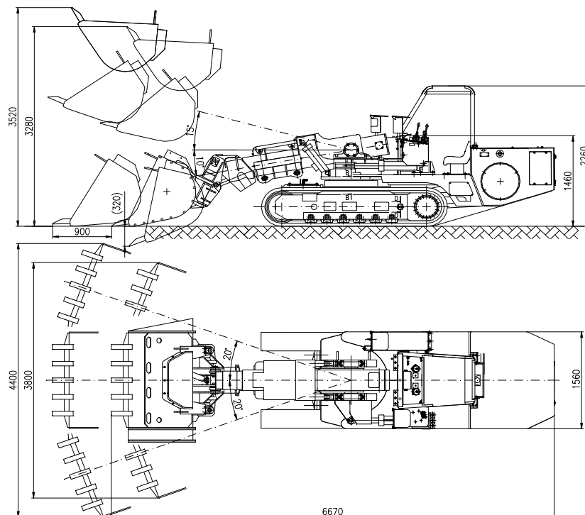
Rys.7. Ładowarka ŁBT-1200M – wymiary [1]
