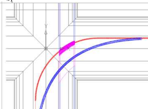
Rys.8. Model 3D trasy kolejki podwieszanej – transport obudowy zmechanizowanej [2]
