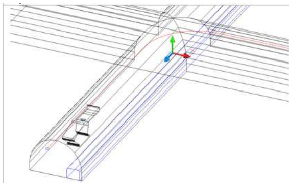
Rys.8. Model 3D trasy kolejki podwieszanej – transport obudowy zmechanizowanej [2]
