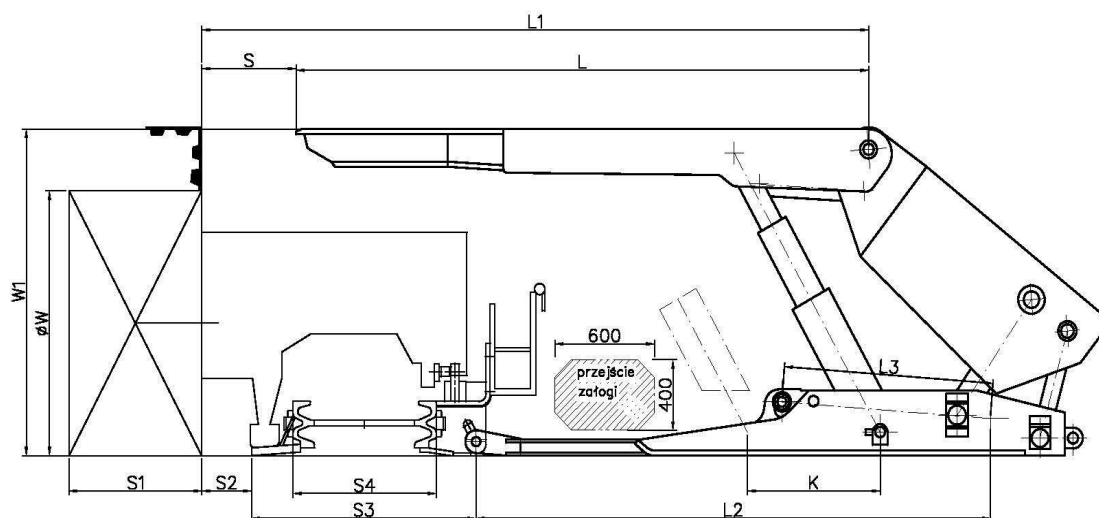
Rys.1. Przykładowy przekrój przez ścianę niezbędny do wydania „Opinii rzeczoznawcy”
