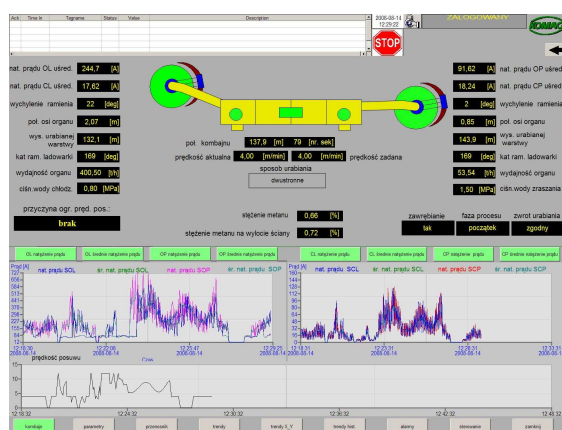
Rys.1. Interfejs Zintegrowanego systemu sterowania i oceny stanu technicznego ścianowego systemu mechanizacyjnego [2]
