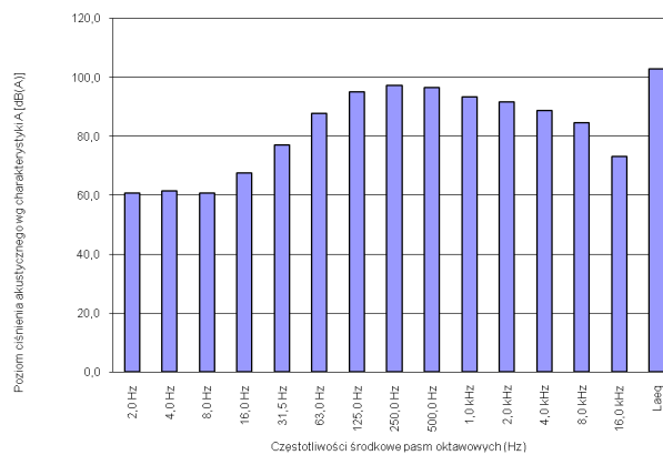
Rys.7. Uśrednione widmo emisji dźwięku wentylatora promieniowego [8]: a) przed zabudowaniem tłumika, b) po zabudowie tłumika
