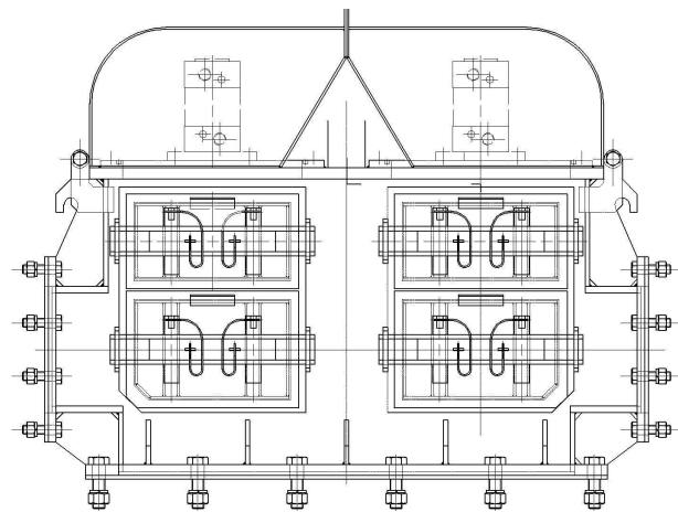
Rys.1. Zawór pulsacyjny dwutalerzowy typu KOMAG [8, 10]
