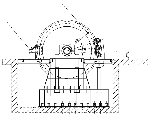
Rys.8. Maszyna wyciągowa 2L-4000/DC-6m/s
