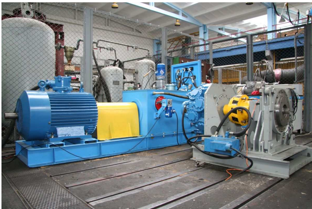
Rys.4. Stanowisko do badań elementów hydrauliki górniczej [źródło: fot. KOMAG]
