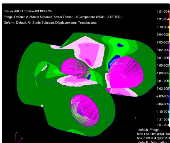
Rys.9. Symulacja MES obciążenia wału Cardana [1]
