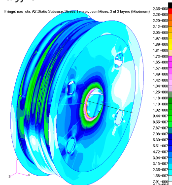
Rys.8. Mapy naprężeń w linopędni w odniesieniu do warunków ruchowych i awaryjnych
