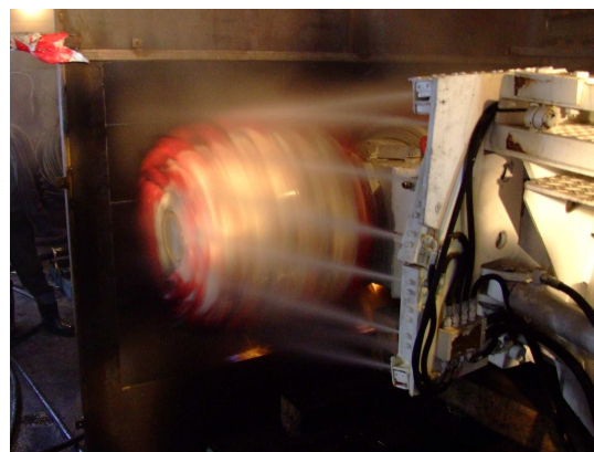
Rys.10. Badania skuteczności kurtyny w gaszeniu i niedopuszczaniu do zapłonu gazu [7]
