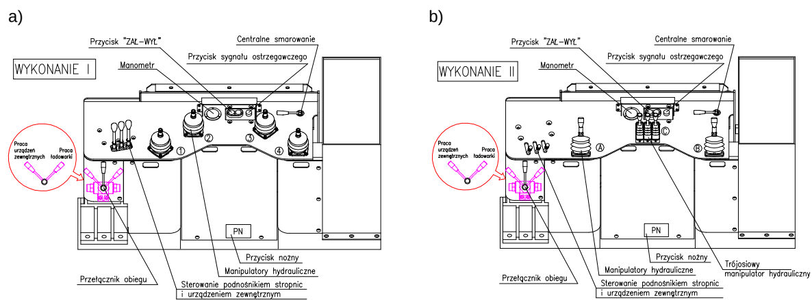
Rys.8. Pulpit operatora ładowarki ŁBT-1200M: a) - wykonanie I, b) - wykonanie II [1]
