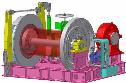
Rys.5. Model wciągarki KUBA-5
