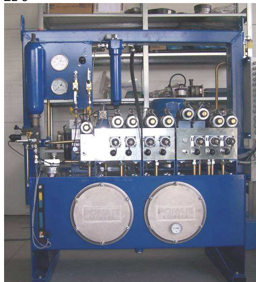
Rys.3. Agregaty hydrauliczne zespołu sterowania EL
