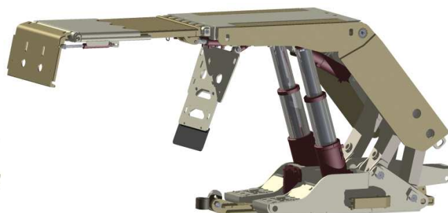
Rys.5. Sekcja obudowy zmechanizowanej KHW-12/28-POz/BSN [2]
