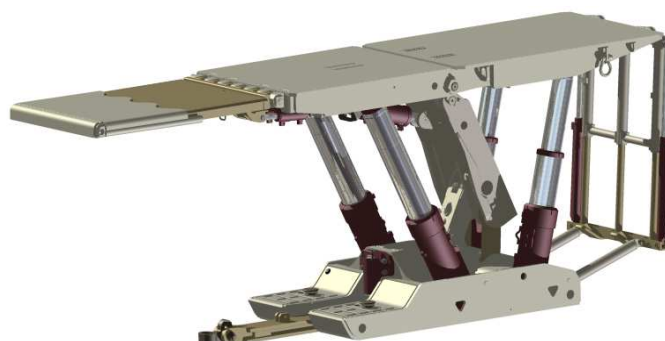
Rys.3. Sekcja obudowy zmechanizowanej KHW-14/24-Pp/BSN [1]
