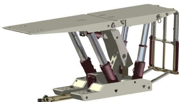
Rys.2. Sekcja obudowy zmechanizowanej KHW-14/24-Pp [1]
