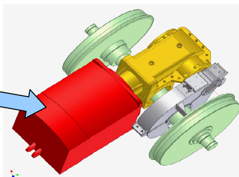
↑ Rys.13. Zespół napędowy z silnikiem z magnesami trwałymi Popg-250L lokomotywy Ld-31EM
