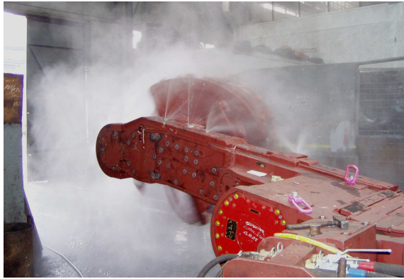
Rys.1. Kombajn ścianowy KSW-460NE wyposażony w nowe rozwiązanie instalacji zraszającej powietrzno-wodnej [2]
