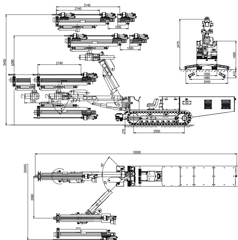
Rys.2. Wymiary wozu MWW-1 [4]
