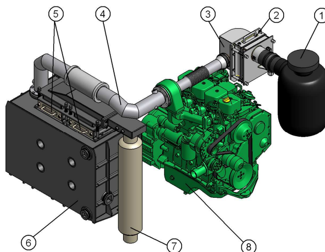
Rys.4. Górniczy napęd spalinowy [3]
