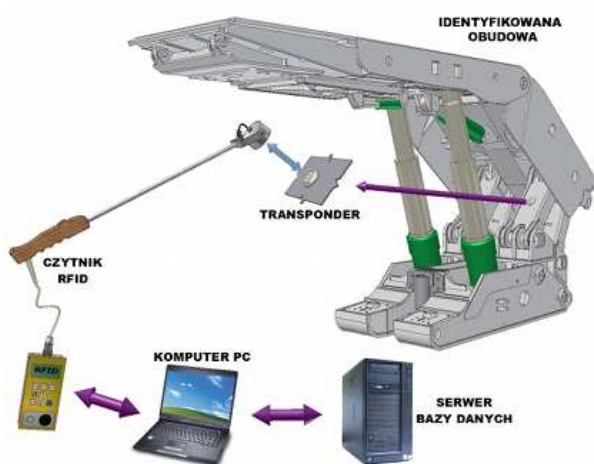
Rys.3. Elementy Elektronicznego Systemu Ewidencji Elementów Sekcji Ścianowej Obudowy Zmechanizowanej [3]
