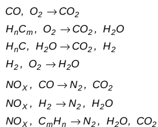
Rys.2. Budowa katalizatora oraz zachodzące w nim reakcje [1]
