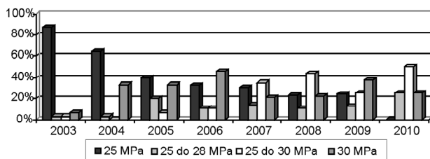
Rys.8. Rozkład ciśnienia zasilania ścian wydobywczych [3]
