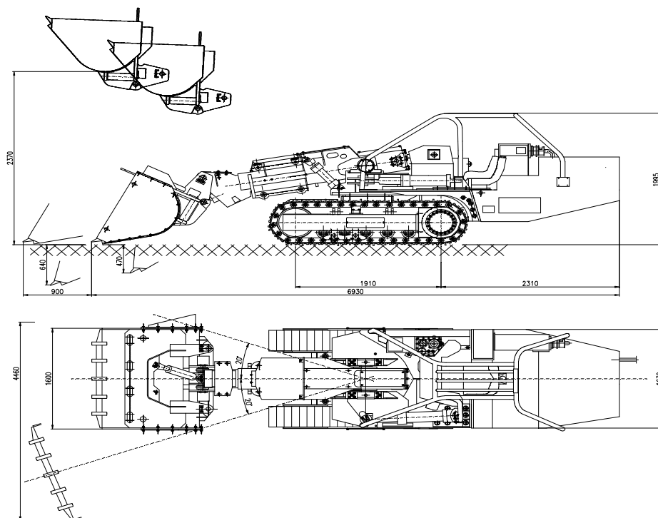
Rys.10. Ładowarka ŁJK-1200 – gabaryty [15]
