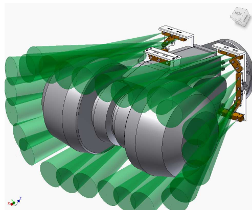
Rys.8. Modele rozkładu strumieni zraszających na ramionach kombajnów chodnikowych [6]
