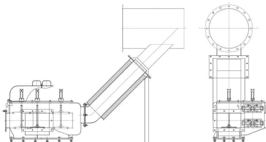
Rys.2. Zawór pulsacyjny dwuciśnieniowy z napędem hydraulicznym typu KOMAG [8, 10]
