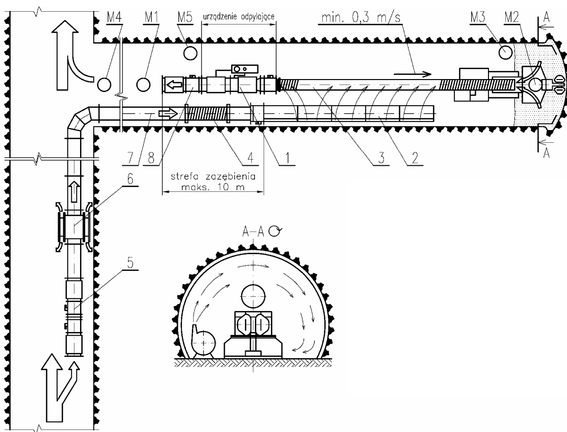
Rys.1. Schemat układu wentylacji kombinowanej [5, 11]
