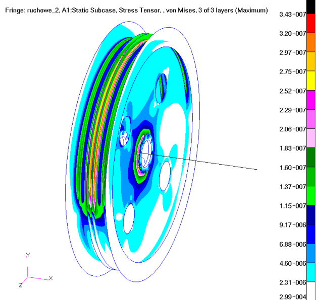
Rys.13. Wyniki analiz numerycznych MES – mapy naprężeń zredukowanych w linopędniach
