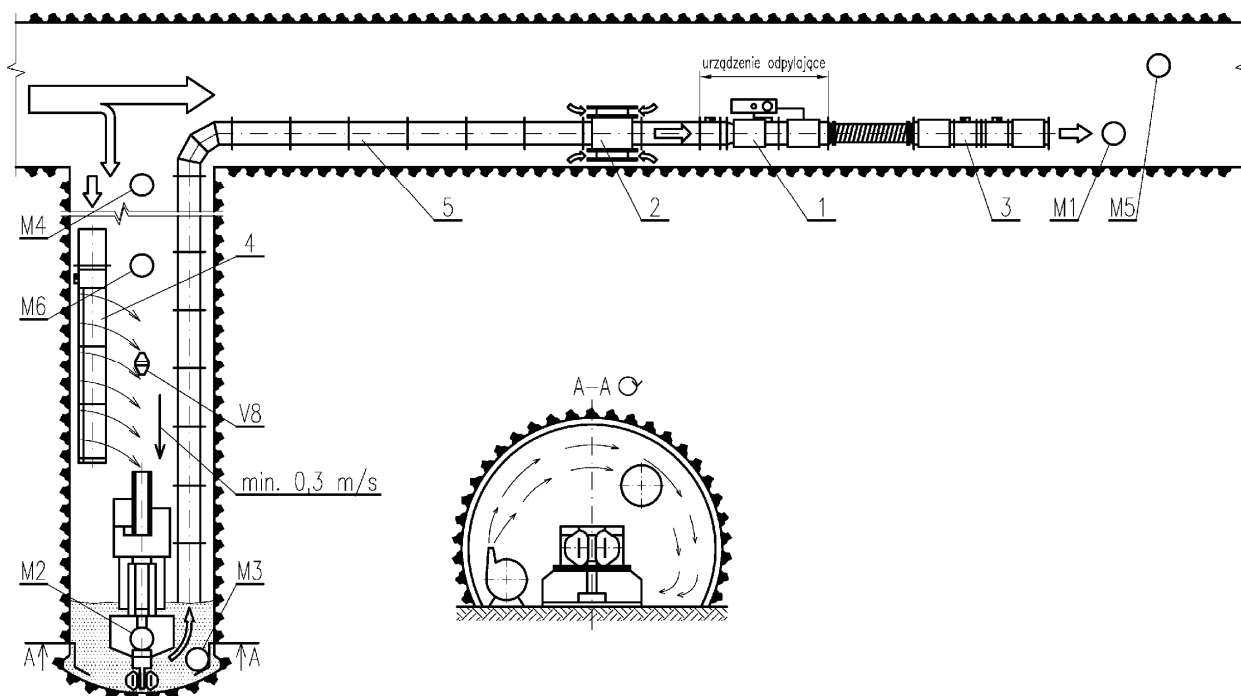
Rys.2. Schemat układu wentylacji ssącej [5, 11]
