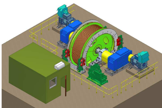
Rys.11. Model 3D maszyny wyciągowej B-4300/DC-8m/s
