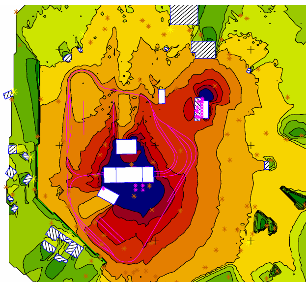
Rys.1. Model rzeźby terenu w rejonie projektowanego szybu górniczego [5]
