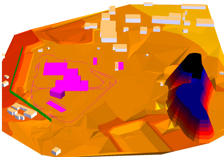
Rys.1. Model rzeźby terenu w rejonie projektowanego szybu górniczego [5]
