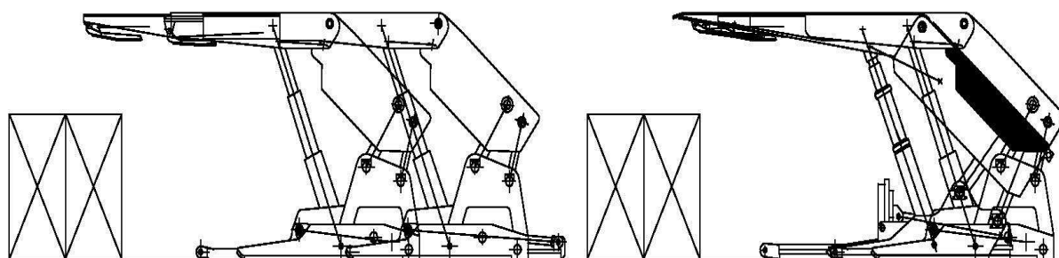
Rys.14. Przykładowa analiza „wysprzęglania się” osłon bocznych osłon odzawałowych
