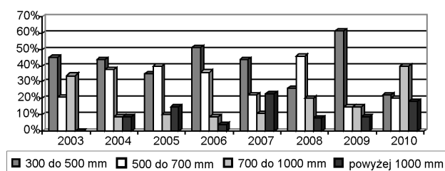
Rys.12. Wielkość ścieżki przystopowej dla sekcji skrajnych w rejonie napędu zwrotnego [3]
