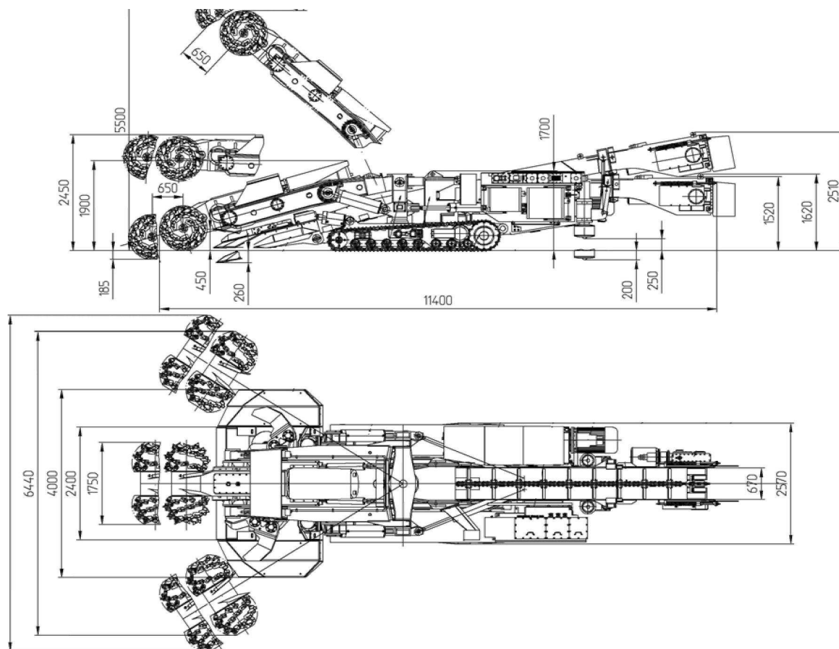
Rys.3. Kombajn chodnikowy P110-01M [6]
