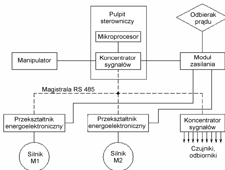
Rys.9. Schemat blokowy sterowania z nowoczesnym pulpitem
