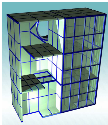
↓ Rys.6. Tłumik hałasu do współpracy z wentylatorami dużej mocy [8, 10]
