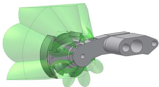
Rys.3. Modele rozkładu strumieni zraszających na ramieniu kombajnu ścianowego [4]
