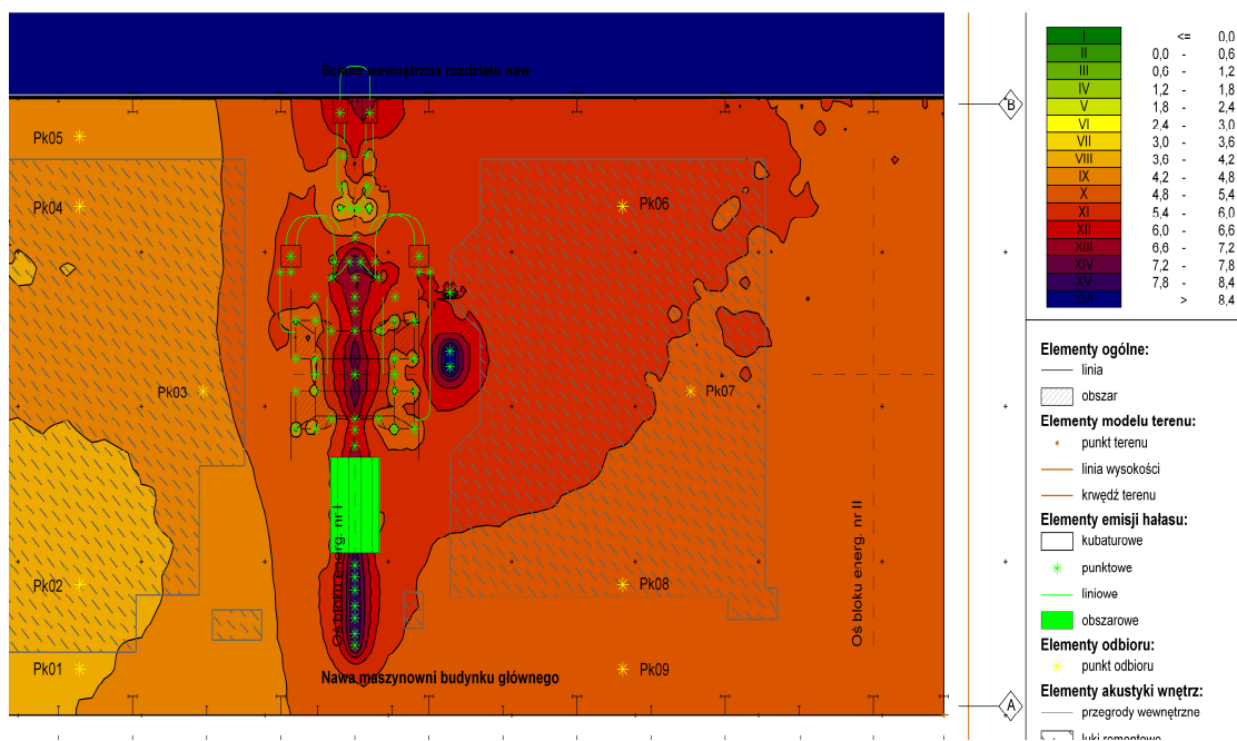
Rys. 7. Rozkład pola akustycznego bez osłony rejonu wzbudzenia dla złożonych źródeł emisji dźwięku [4]
