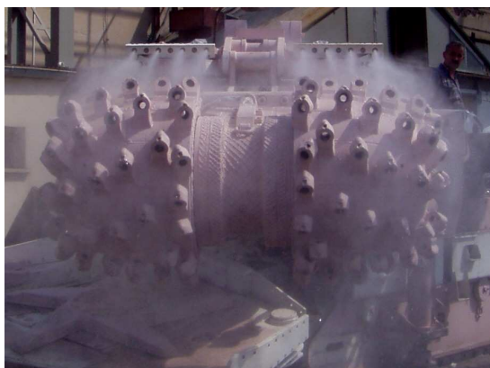
Rys.9. Działanie kurtyny powietrzno-wodnej na kombajnie chodnikowym [6]
