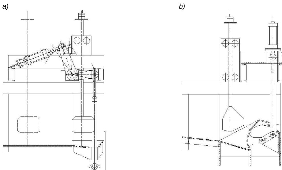
Rys.5. Koncepcje przepustu produktów dla osadzarek miałowych (a) i średnioziarnowych (b) typu KOMAG [7, 10]
