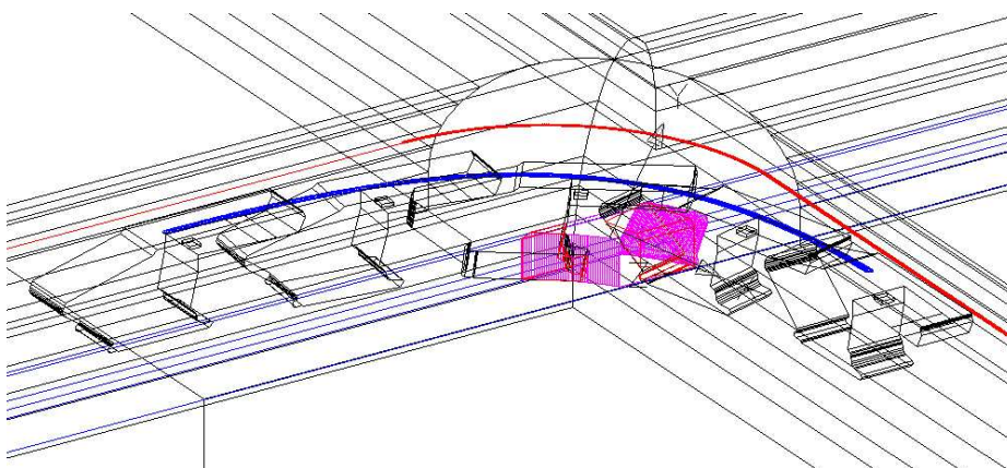
Rys.9. Symulacja transportu obudowy zmechanizowanej modułowym zestawem nośnym [2]
