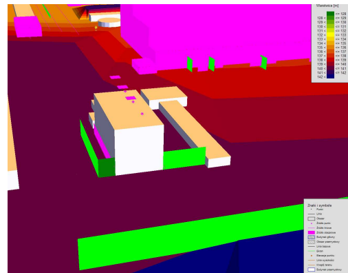
Rys.1. Ekran akustyczny w rejonie chłodni wyparnej turbiny: a) model geometryczny, b) model akustyczny [6]
