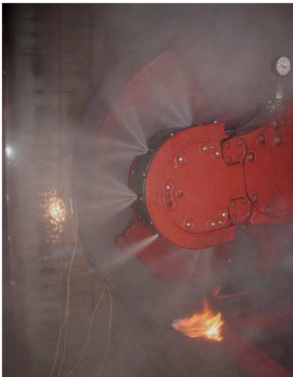
Rys.6. Badania powietrzno-wodnej instalacji zraszającej [źródło: fot. KOMAG]
