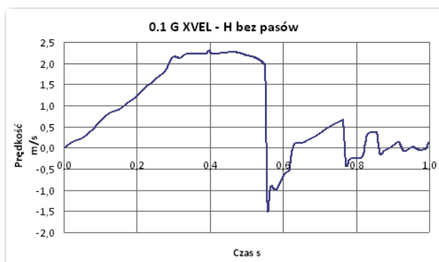
Rys.12. Przebieg prędkości dla głowy operatora [1]
