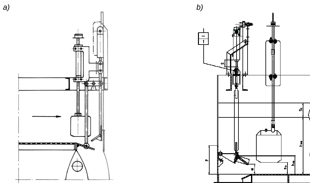
Rys.4. Przepusty klawiszowe produktów w osadzarkach ziarnowych (a) i średnioziarnowych (b) typu KOMAG [7, 9]
