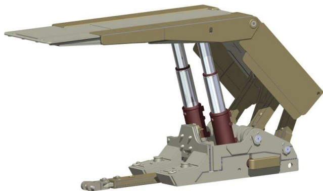
Rys.10. Sekcja obudowy zmechanizowanej KHW-13/26-POz [5]
