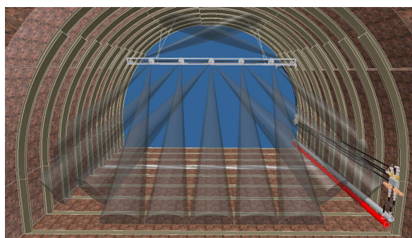
Rys.11. Kurtyna powietrzno-wodna kombajnu R-130, zaprezentowana na Międzynarodowych Targach Górnictwa, Przemysłu Energetycznego i Hutniczego KATOWICE 2009 [8]
