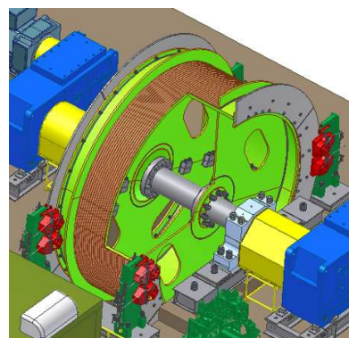
Rys.11. Model 3D maszyny wyciągowej B-4300/DC-8m/s
