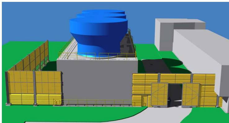
Rys.1. Ekran akustyczny w rejonie chłodni wyparnej turbiny: a) model geometryczny, b) model akustyczny [6]
