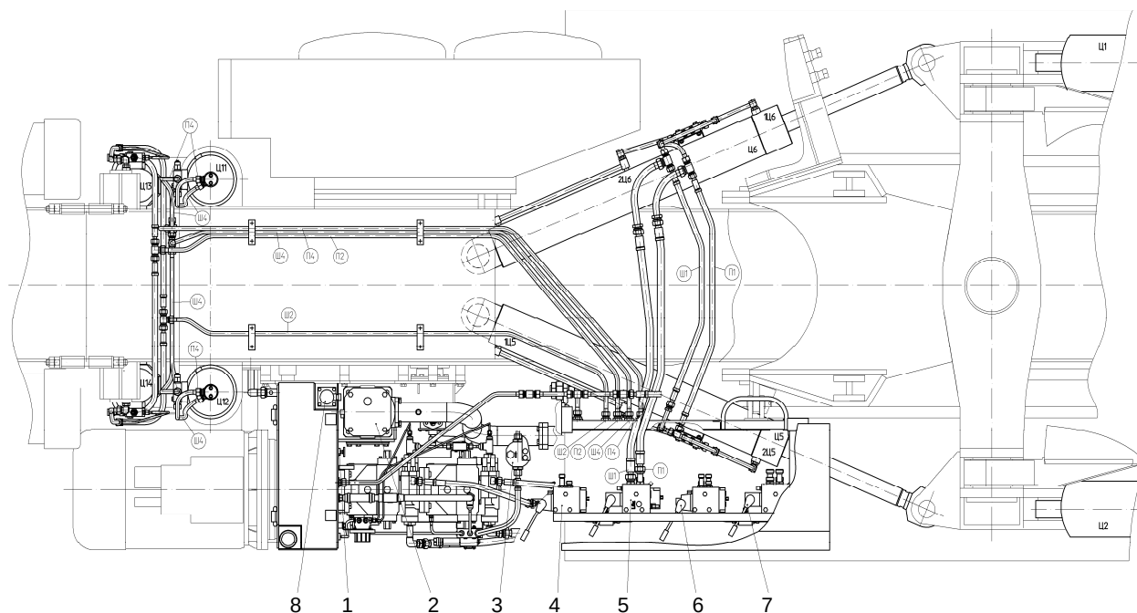
Rys.4. Rozmieszczenie niektórych podzespołów układu hydraulicznego kombajnu chodnikowego P110-01M – widok z góry
