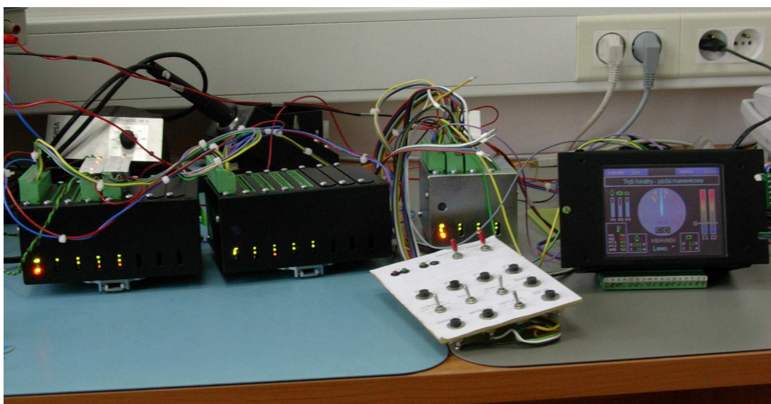
Rys.5. Model pulpitu sterowniczego wraz z koncentratorami sygnałów na stanowisku badawczym (fot. KOMAG)
