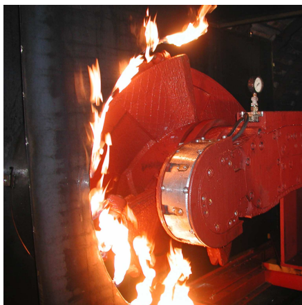
Rys.6. Badania skuteczności instalacji w gaszeniu i nie-dopuszczaniu do zapłonu gazu w KD BARBARA [5]
