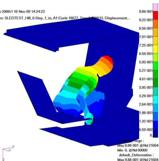
Rys.11. Model ciała operatora ograniczony powierzchnią kabiny kolejki w środowisku programu MSC.Dytran [1]
