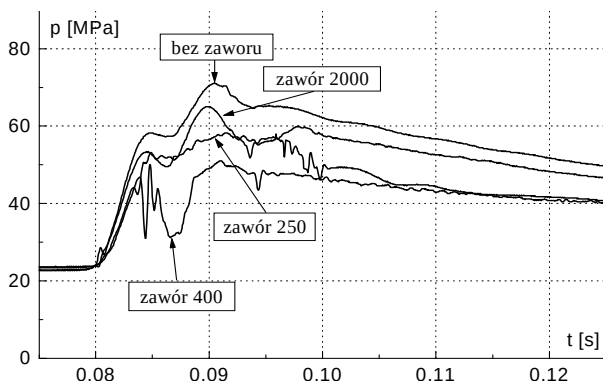
Rys.8. Przebiegi ciśnienia w funkcji czasu w stojaku \Phi 210 podczas obciążenia dynamicznego z użyciem MW, upodatkowanego za pomocą zaworów upustowych o różnej przepustowości [10]
