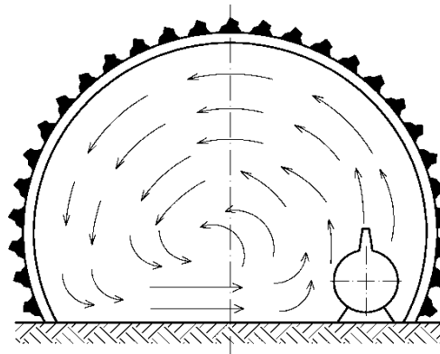
Rys.4. Schemat przewietrzania wyrobiska za pomocą lutni wirowej [9]
