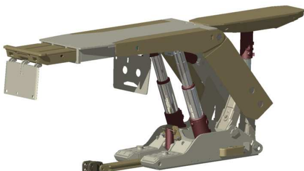
Rys.8. Sekcja obudowy zmechanizowanej KHW-12/28-POz/Pp [3]
