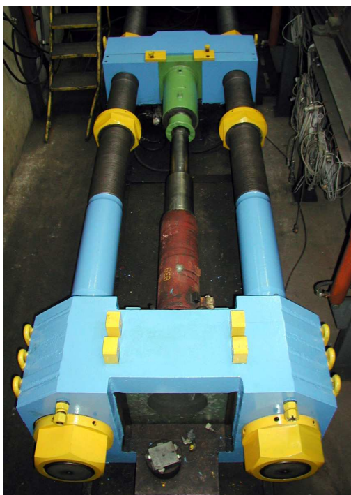
Rys.3. Stanowisko do badań stojaków oraz elementów hydrauliki wysokociśnieniowej
