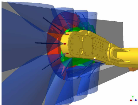
Rys.3. Modele rozkładu strumieni zraszających na ramieniu kombajnu ścianowego [4]
