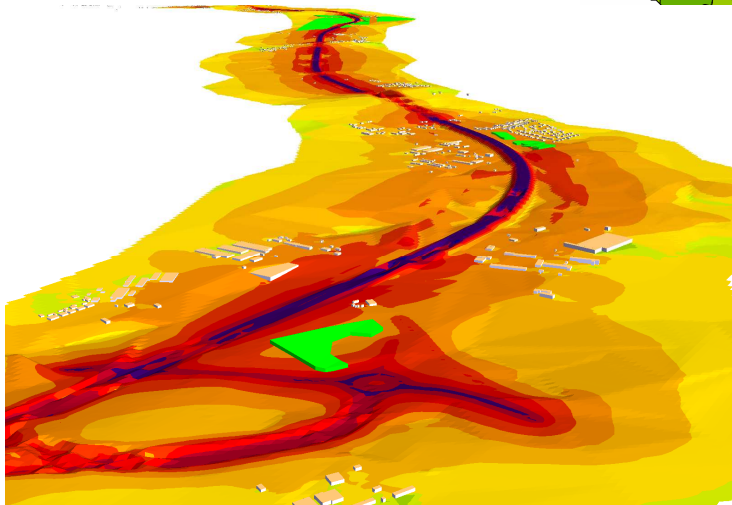
Rys.2. Rozkład pola akustycznego wyznaczony w rejonie projektowanego szybu górniczego z uwzględnieniem hałasu drogowego i kolejowego [5]
