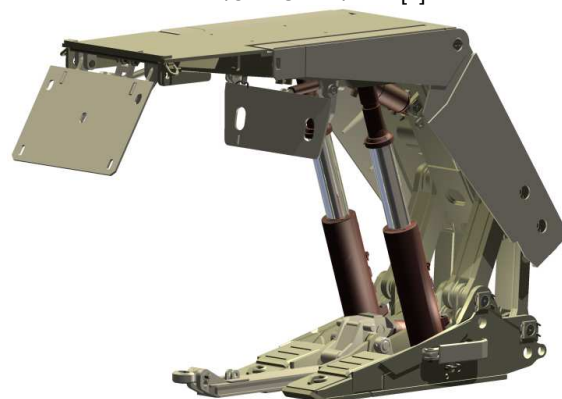
Rys.15. Sekcja obudowy zmechanizowanej KW-12/31-POzW2/ZRP [8]
