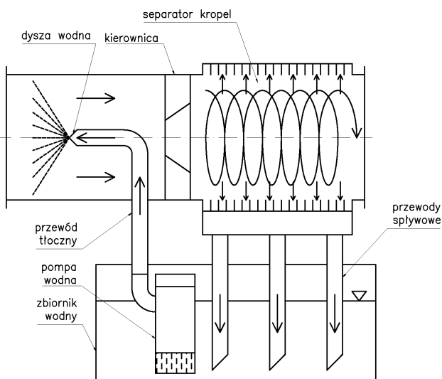
Rys.3. Obieg wody i powietrza w mokrym urządzeniu odpylającym
