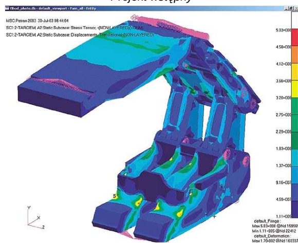
Obliczenia MES
