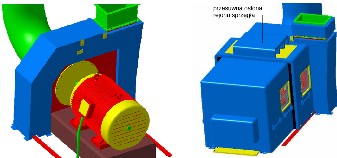
Rys.10. System tłumienia wentylatora [7]
