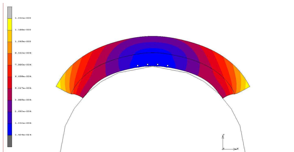
Rys.15. Mapa odkształceń segmentu tarczy hamulcowej w wyniku jej nagrzewania
