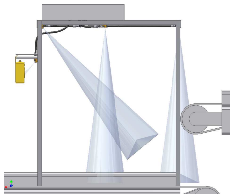
Rys.10. Badania skuteczności kurtyny w gaszeniu i niedopuszczaniu do zapłonu gazu [7]
