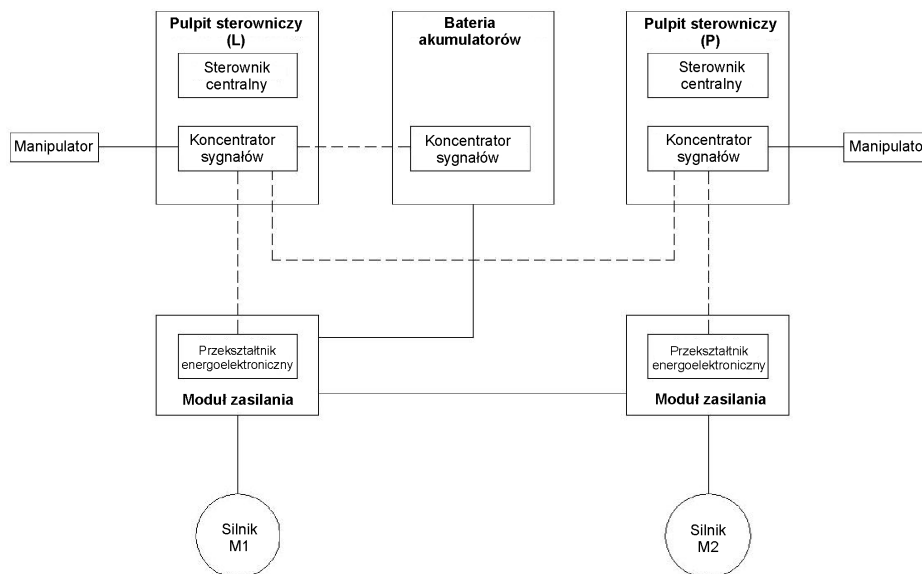
Rys.13. Schemat blokowy sterowania lokomotywy akumulatorowej
