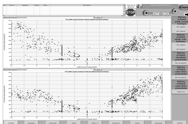
Rys.1. Interfejs Zintegrowanego systemu sterowania i oceny stanu technicznego ścianowego systemu mechanizacyjnego [2]
