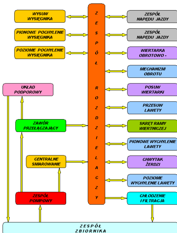
Rys.6. Schemat blokowy układu hydraulicznego małowabarytowego wozu wiertniczego MWW-1
