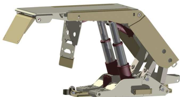
Rys.4. Sekcja obudowy zmechanizowanej KHW-12/28-POz [2]
