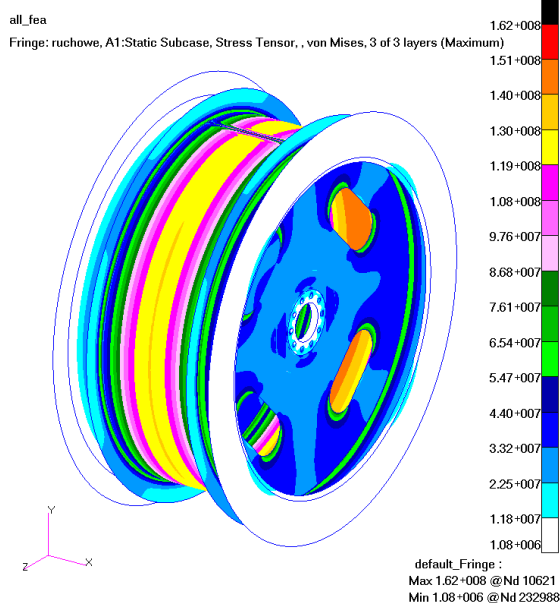
Rys.13. Wyniki analiz numerycznych MES – mapy naprężeń zredukowanych w linopędniach
