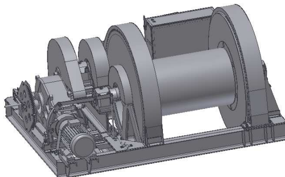
Rys.6. Model wciągarki KUBA-10
