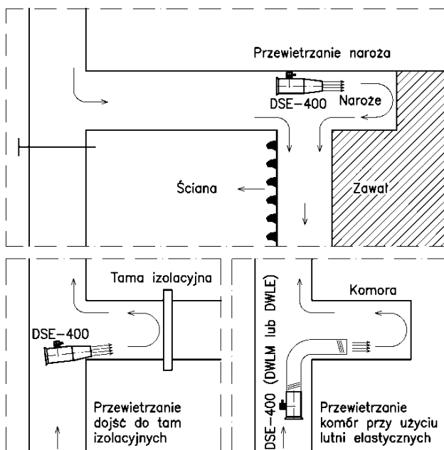
Rys.10. Przykłady zastosowania dmuchawy DSE-400 [10]
