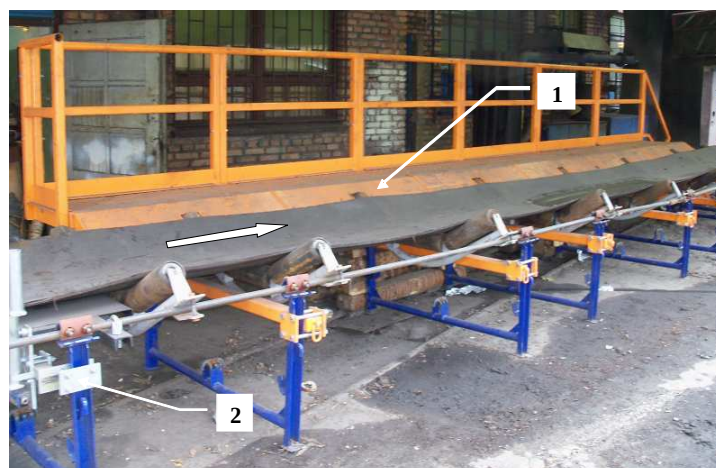
Rys.8. Pomost do wysiadania poz. 1 z czujnikiem schodzenia taśmy poz. 2
