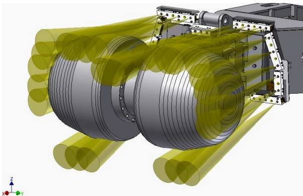
Rys.8. Modele rozkładu strumieni zraszających na ramionach kombajnów chodnikowych [6]
