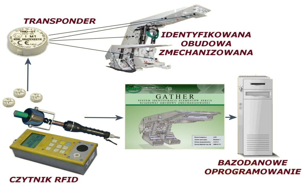
↓ Rys.16. System elektronicznej identyfikacji elementów sekcji ścianowej obudowy zmechanizowanej
