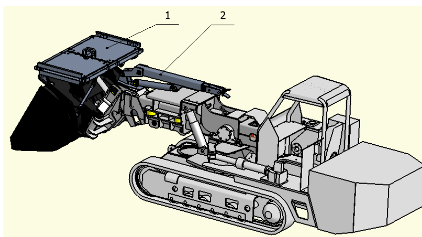
Rys.12. Urządzenie do wznoszenia obudowy chodnikowej WOCh-1 [2]
