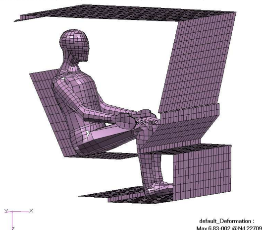
Rys.11. Model ciała operatora ograniczony powierzchnią kabiny kolejki w środowisku programu MSC.Dytran [1]
