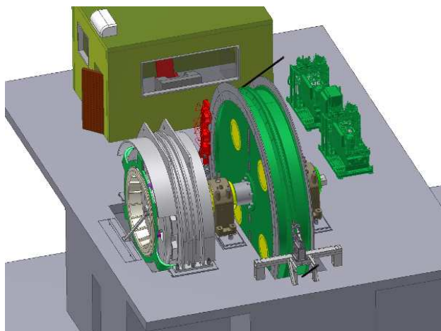
Rys.12. Model 3D maszyny wyciągowej K-6000/DC-16m/s
