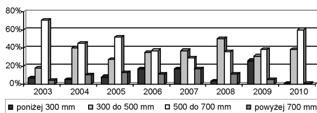
Rys.10. Wielkość ścieżki przystopowej dla sekcji liniowych [3]
