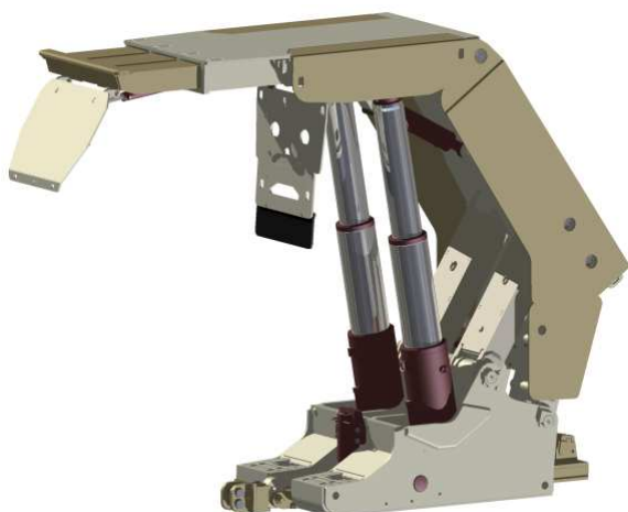
Rys.6. Sekcja obudowy zmechanizowanej KHW-24/46-POz [4]
