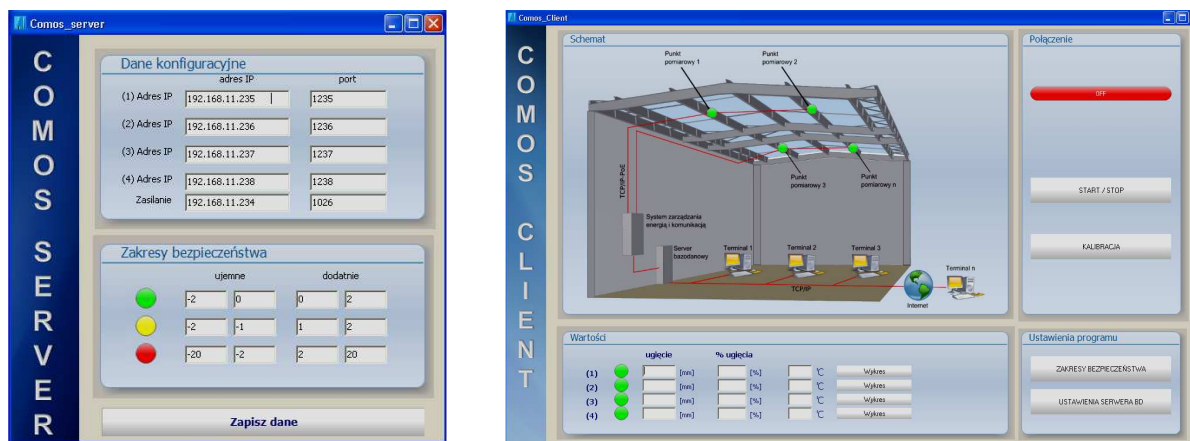
Rys. 7. System monitoringu konstrukcji [5]
