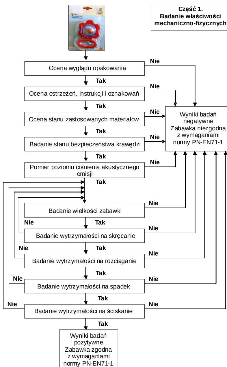
Rys.4. Algorytm badań właściwości mechaniczno-fizycznych zabawki-grzechotki [1]
