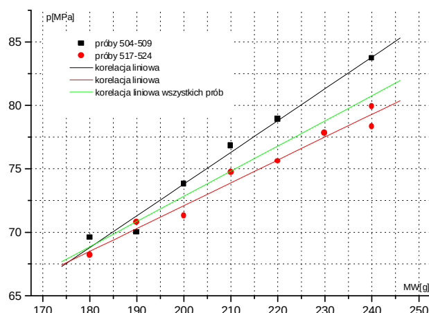
Rys.9. Stojak \Phi 250 mm. Wykresy korelacji liniowych dla prób dynamicznych z materiałem wybuchowym typu BAZALT [7]
