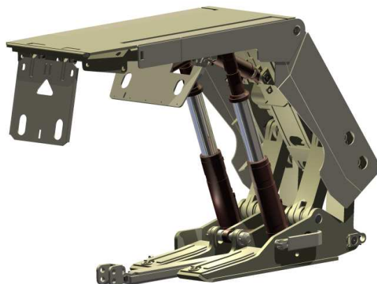
Rys.11. Sekcja obudowy zmechanizowanej KW-12/28-POz/ZRP [6]
