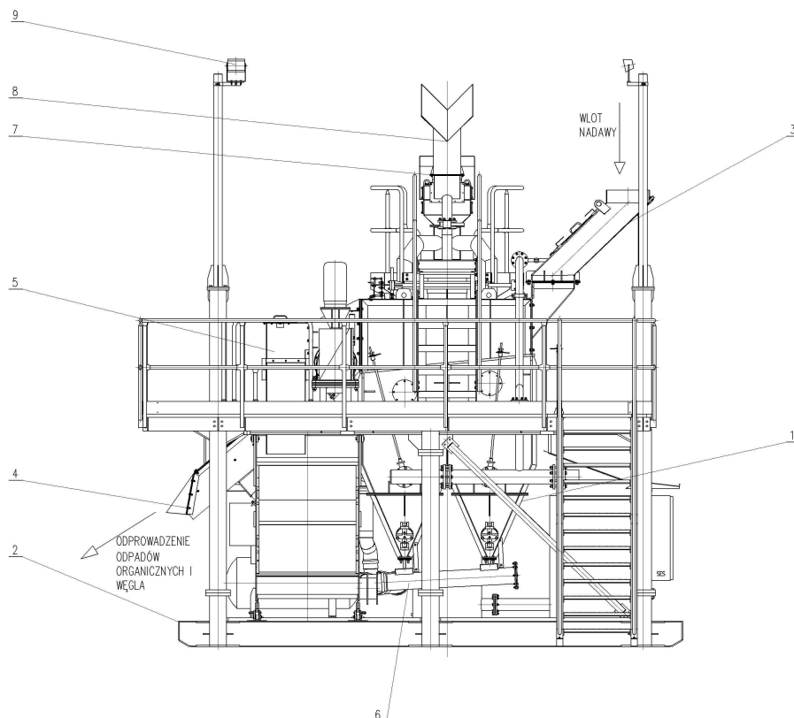
Rys.1 Klasyfikator pulsacyjny K101 [5]
