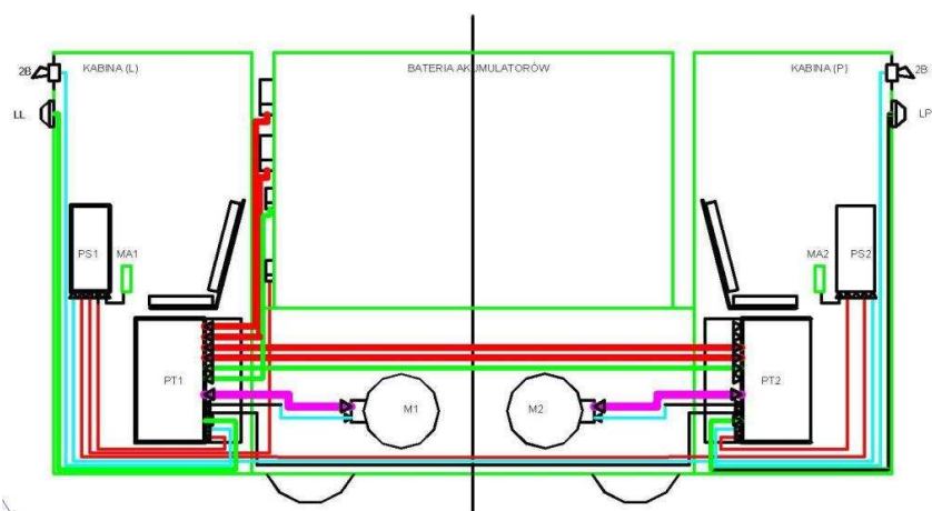
Rys.12. Koncepcja napędu i sterowania lokomotywy Lea BM-12
