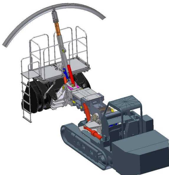
Rys.14. Urządzenie WOCh-1: a) podest złożony, b) podest rozłożony [1]
