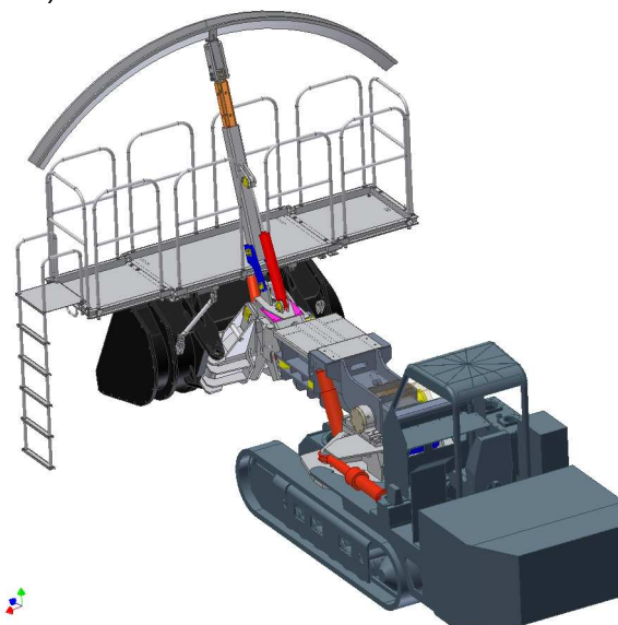
Rys.14. Urządzenie WOCh-1: a) podest złożony, b) podest rozłożony [1]
