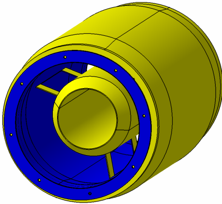
Rys.4. Tłumiki typu TG, do stosowania w atmosferze zagrożenia wybuchem metanu i pyłu węglowego [4, 5]: a) tłumik TG 630/2000, b) typoszereg tłumików TG z elementem rozpraszającym
