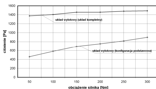
Rys.1. Zmiany wartości ciśnienia w układzie wylotowym w zależności od jego konfiguracji [3]
