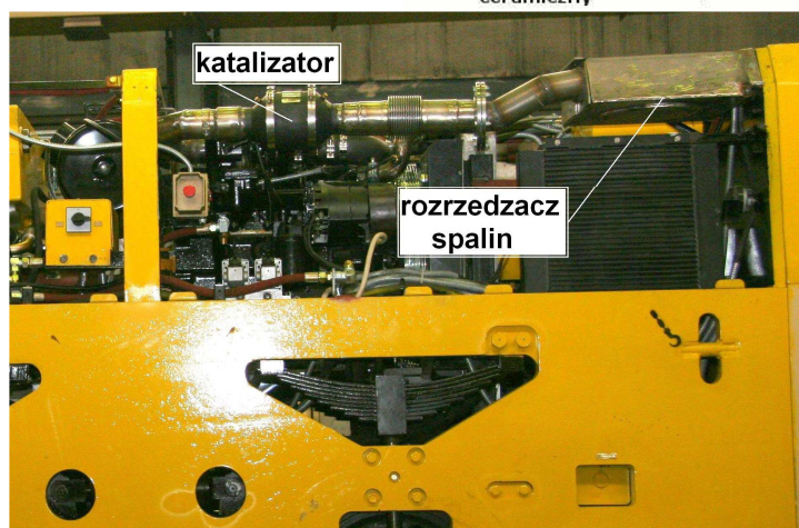
Rys.3. Lokomotywa Lds100K-EM z zabudowanym katalizatorem [1]
