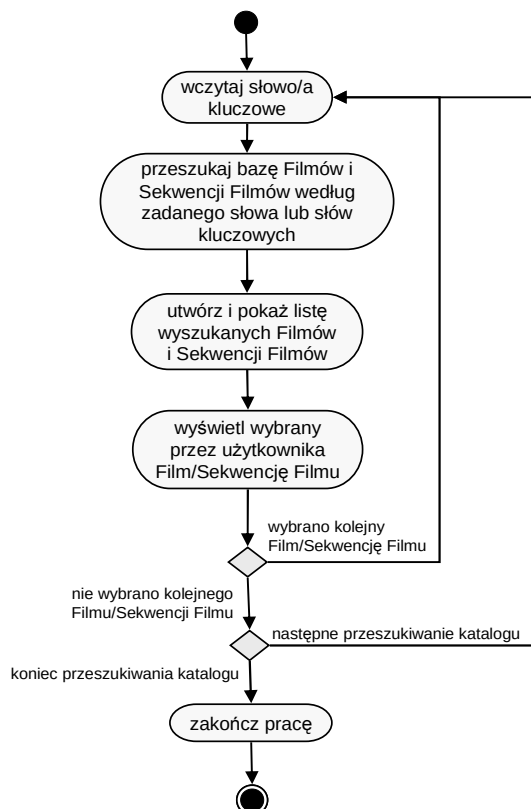
Rys.3. Sposób działania aplikacji IKFW [opracowanie własne]
