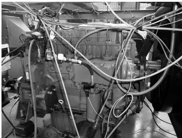
Rys.2. Silnik spalinowy Volvo Penta D5A T na stanowisku badawczym [1]
