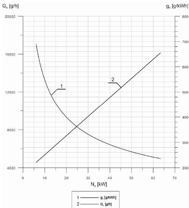
Rys.7. Godzinowe i jednostkowe zużycie paliwa
