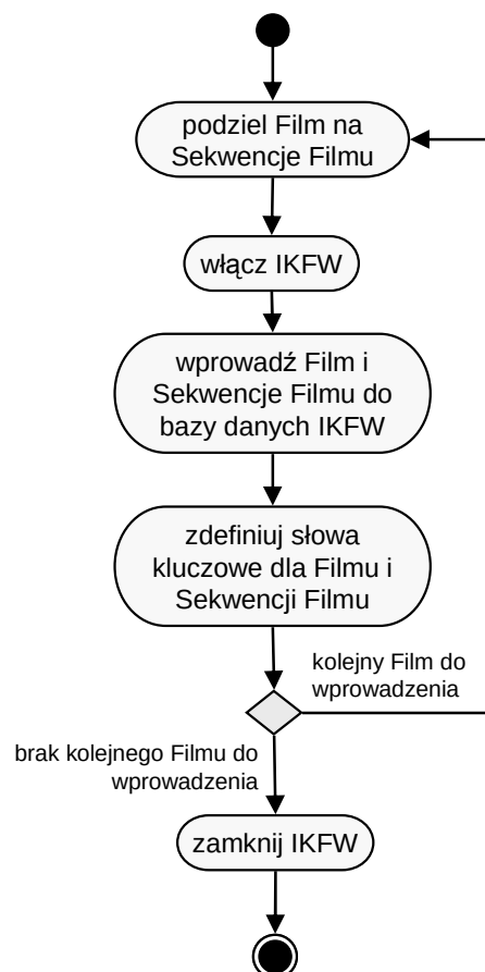
Rys.1. Przygotowanie zasobów aplikacji IKFW [opracowanie własne]
