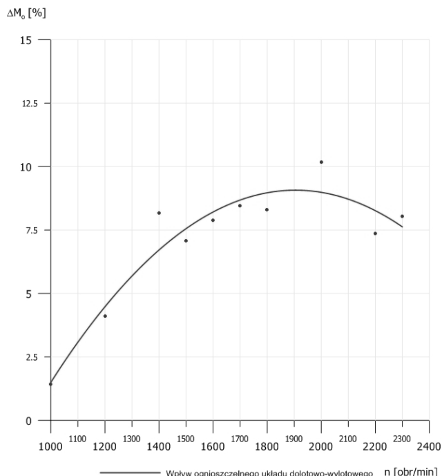
Rys.11. Wpływ ognioszczelnego układu dolotowo-wylotowego w wersji według rozwiązania KOMAG-u na parametry (moc, moment obrotowy) uzyskiwane przez silnik [1]
