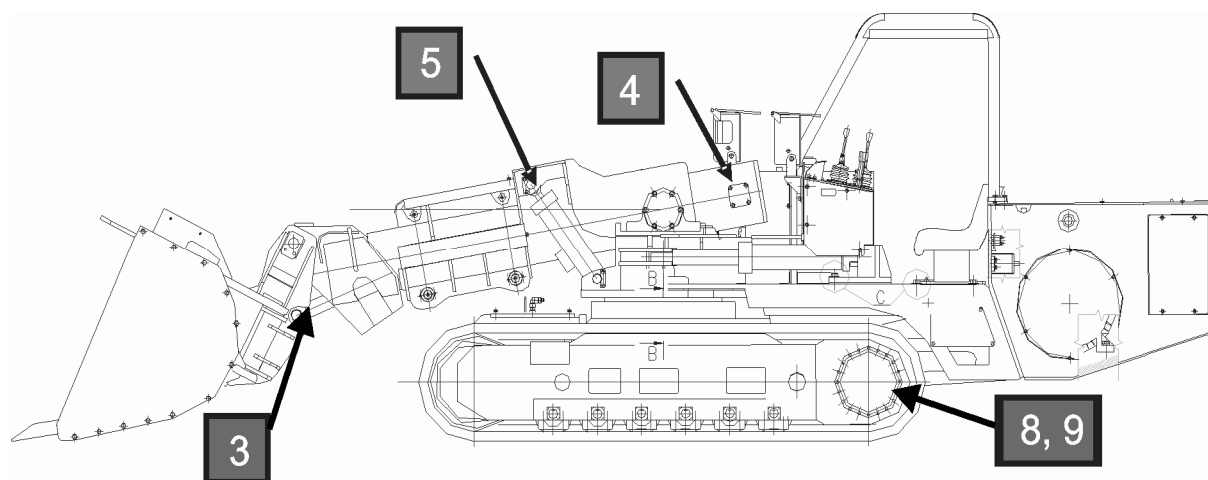
Rys.3b. Rozmieszczenie przetworników pomiarowych [opracowanie własne ITG KOMAG]
