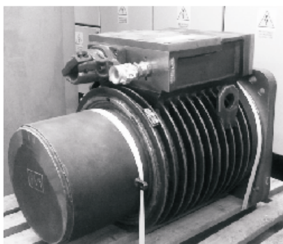
Rys.4. Silnik PMSM typu SMwsd 200 S-4, wraz z podstawowymi parametrami technicznymi [1]
