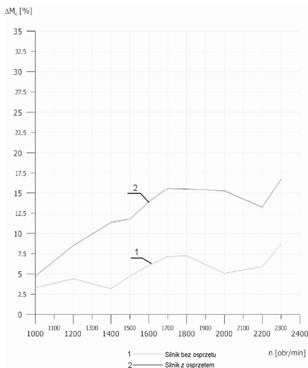
Rys.10. Procentowe zmiany wartości momentu obrotowego silnika D5A T w odniesieniu do wartości deklarowanych przez producenta [1, 12]
