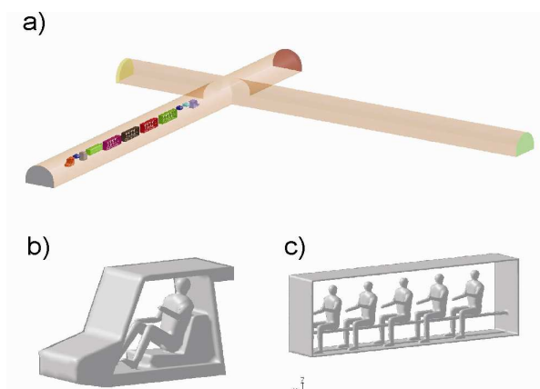
Rys.2 a) Model geometryczny analizowanego fragmentu wyrobiska, b) kabina operatora kolejki, c) ława do przewożenia ludzi [15]
