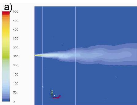
Rys.4. Wykres konturowy prędkości mieszaniny w płaszczyźnie przechodzącej przez oś wlotu poprzecznego i oś dyszy a) i izopowierzchnia dla udziału objętościowego wody równego \alpha = 1 b) dla zasilania powietrzem prostopadłe do osi dyszy. Te same wykresy dla zasilania powietrzem równoległe do osi dyszy odpowiednio rysunki c) i d). Prędkość wyrażono w m/s [16]
