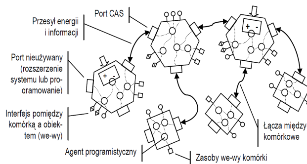
Rys.2. Model systemu roju z programowaniem agentowym [2]
