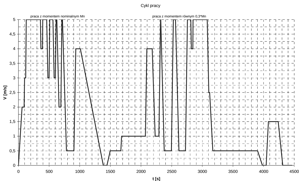
Rys. 7. Zamodelowany cykl pracy górniczej lokomotywy akumulatorowej [2]
