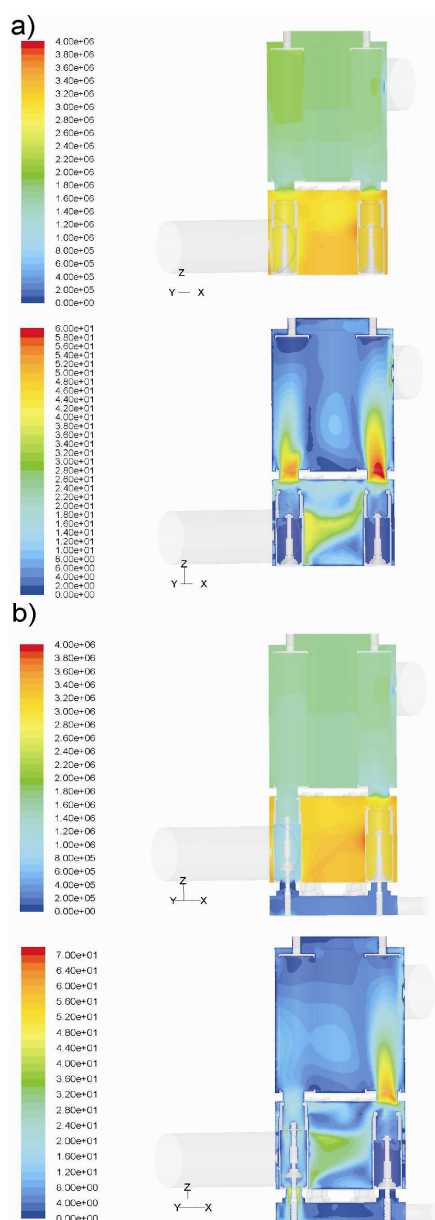
Rys.1. Wykres konturowy ciśnienia statycznego (u góry) i prędkości (u dołu) w płaszczyźnie pionowej przechodzącej przez osie wkładów filtracyjnych dla normalnej pracy filtra a) i dla stanu przepłykiwania jednego z filtrów b) p = 4 \text{ MPa}
