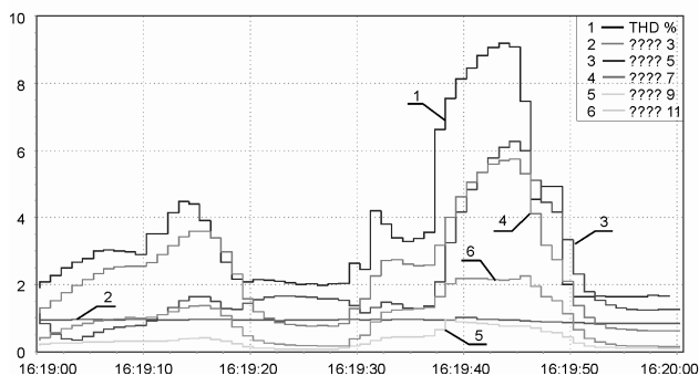
Rys.1. Wartości wyższych harmonicznych napięcia w ciągu cyklu transportu pionowego
