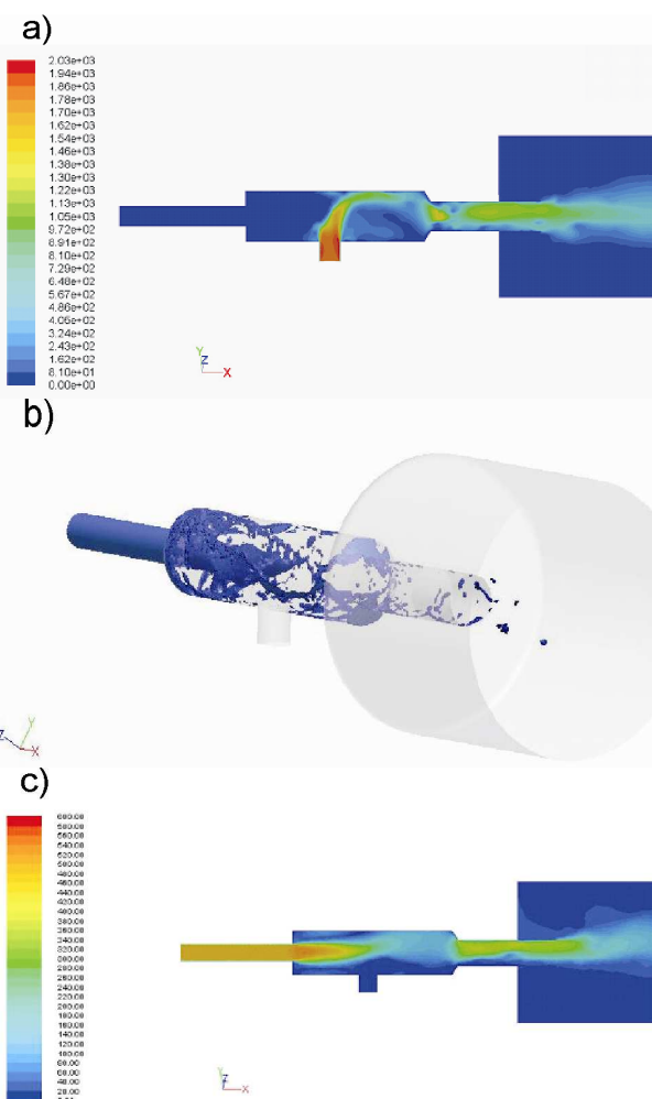
Rys.3. Rozkład udziału objętościowego tlenu węgla w przekroju wyrobiska a) na wysokości twarzy przewożonych ludzi w przykładowej fazie ruchu fazach ruchu tj. dla t = 135 \text{ s} , b) dla ławy znajdującej się bezpośrednio za jednostką napędową zestawu transportowego [15]
