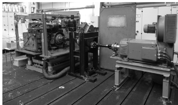
Rys.1. Stanowisko do badań górnich napędów spalinowych zbudowane w KOMAG-u. [1]
