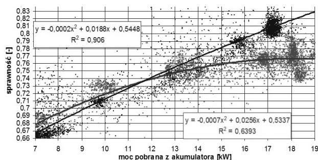
Rys. 9. Przebiegi sprawności układu napędowego z silnikiem synchronicznym z magnesami trwałymi typu SMwsd 200 S-4 (górny) oraz układu napędowego z silnikiem asynchronicznym typu dSkg 180L4-EP-f (dolny) w funkcji mocy pobieranej z akumulatora podczas cykli pomiarowych I – VI [3]
