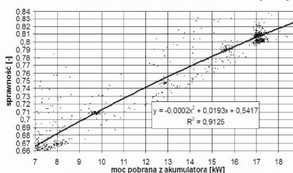
Rys.10. Zestawienie uzyskanych sprawności podczas wybranych cykli pomiarowych
