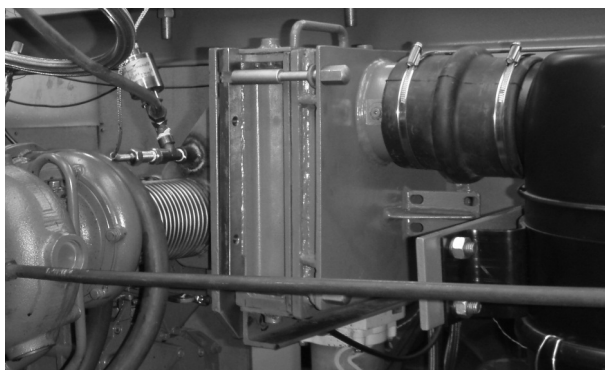
Rys.3. Układ dolotowy silnika [1]
