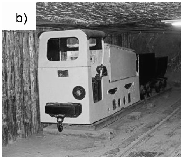
Rys.2. Górnicze lokomotywy akumulatorowe produkcji polskiej [3] a) Lea BM-12, b) Ldag 05M
