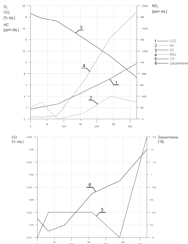
Rys.12. Ilość substancji szkodliwych w spalinach w funkcji obciążenia dla stałej prędkości obrotowej ( n = 1500 [obr/min]) – silnik bez ognioszczelnego układu dolotowo-wylotowego
