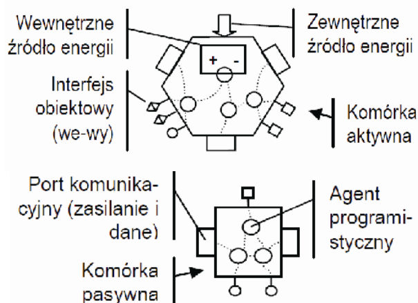
Rys.1. Przykładowe modele komórek roju programowane agentowo [2]
