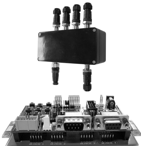
Rys.6. Moduł wejść analogowych [opracowanie własne ITG KOMAG]
