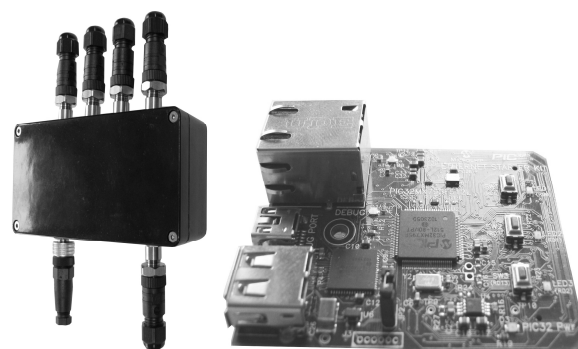
Rys.4. Rejestrator z magistralą CAN [opracowanie własne ITG KOMAG]
