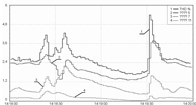
Rys.2. Wartości wyższych harmonicznych napięcia w ciągu cyklu transportu pionowego
