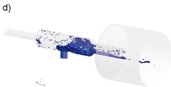
Rys.4. Wykres konturowy prędkości mieszaniny w płaszczyźnie przechodzącej przez oś wlotu poprzecznego i oś dyszy a) i izopowierzchnia dla udziału objętościowego wody równego \alpha = 1 b) dla zasilania powietrzem prostopadłe do osi dyszy. Te same wykresy dla zasilania powietrzem równoległe do osi dyszy odpowiednio rysunki c) i d). Prędkość wyrażono w m/s [16]
