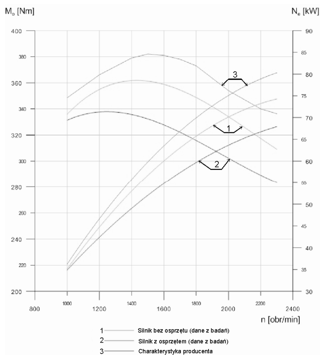
Rys.9. Charakterystyki zewnętrzne silnika D5A T [1, 12]
