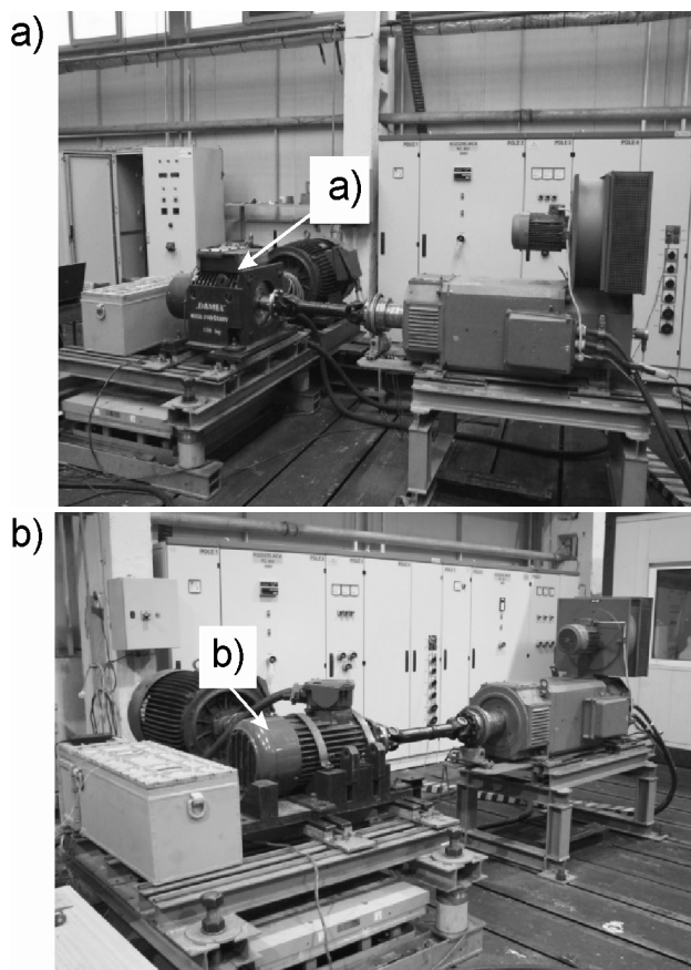
Rys. 8. Stanowisko badawcze [7] a – silnik synchroniczny z magnesami trwałymi typu SMwsd 200 S-4, b – silnik asynchroniczny typu dSkg 180L4-EP-f
