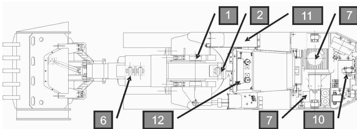
Rys.3a. Rozmieszczenie przetworników pomiarowych [opracowanie własne ITG KOMAG]
