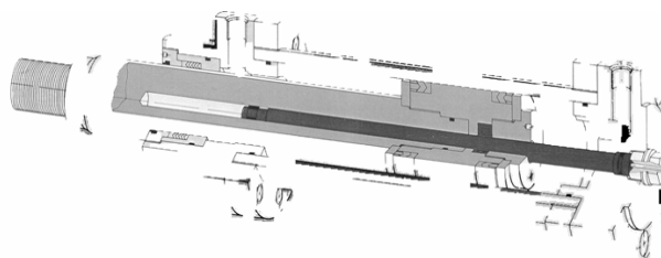
Rys.10. Przetwornik pomiaru długości wysuwu siłownika serii iKMA [2]
