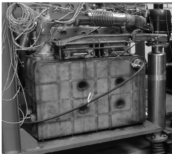
Rys.4. Układ wylotowy silnika [1]
