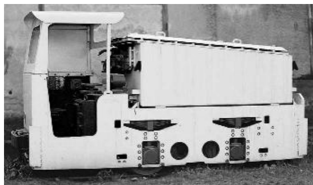
Rys.1. Górnicza lokomotywa akumulatorowa typu Lea BM-5 [7]
