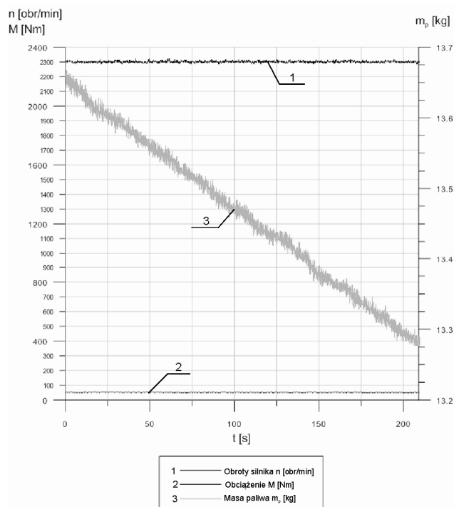
Rys.6. Zużycie paliwa podczas ustalonych parametrów pracy silnika [1]
