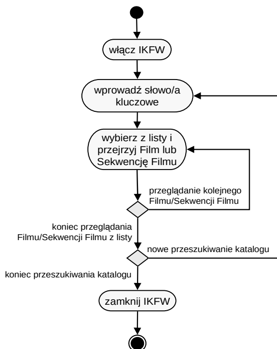
Rys.2. Użytkowanie aplikacji IKFW [opracowanie własne]
