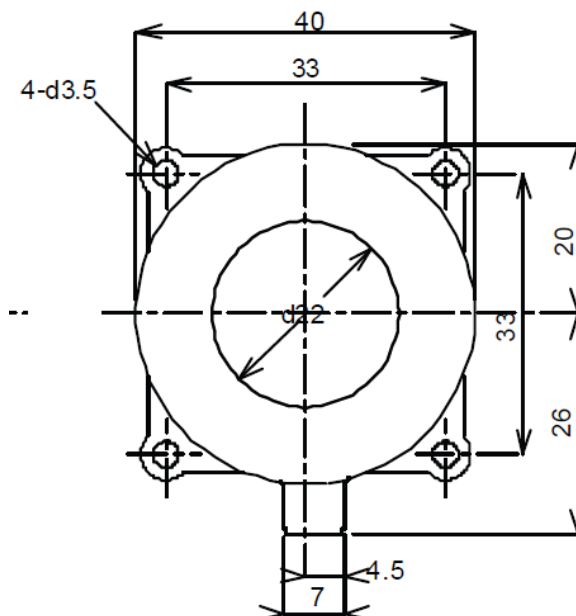
Rys.8. Przekładnik prądowy HTFS [1]
