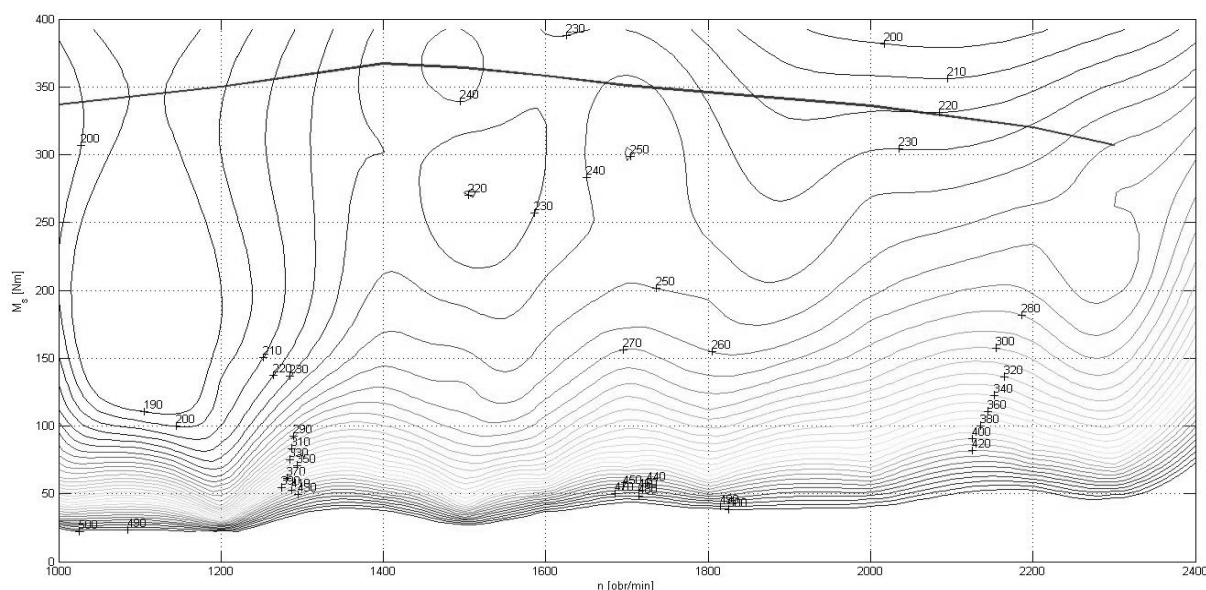
Rys.8. Charakterystyka uniwersalna silnika D5A T bez ognioszczelnego układu dolotowo-wylotowego
