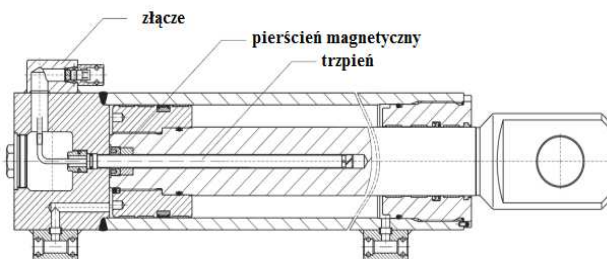
Rys.9. Przetwornik pomiaru długości wysuwu siłownika serii iKMA [2]
