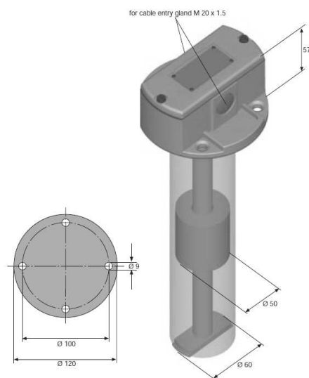
Rys.13. Wymiary przetwornika iTNA16 [2]
