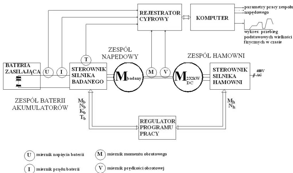
Rys.6. Schemat stanowiska badawczego [1]
