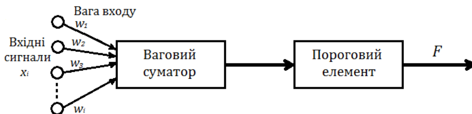
Рис. 1. Модель бінарного нейрона з n входами та одним виходом
