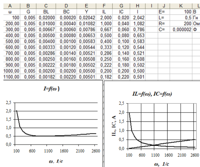
Рис. 12. Чисельні та графічні результати моделювання резонансних явищ у паралельному коливальному контурі за умови змінної частоти джерела напруги
