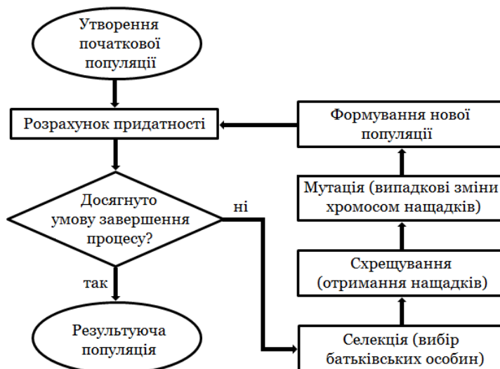
Рис. 2. Загальна схема класичного генетичного алгоритму
