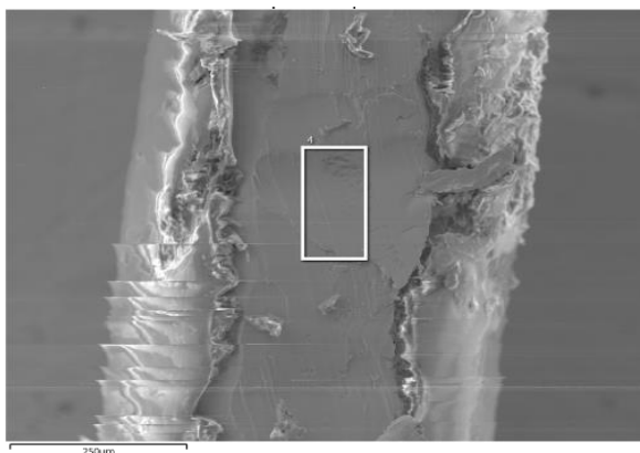
Рис. 17. Мікроструктура мідного дрота після 1 с відпалу
