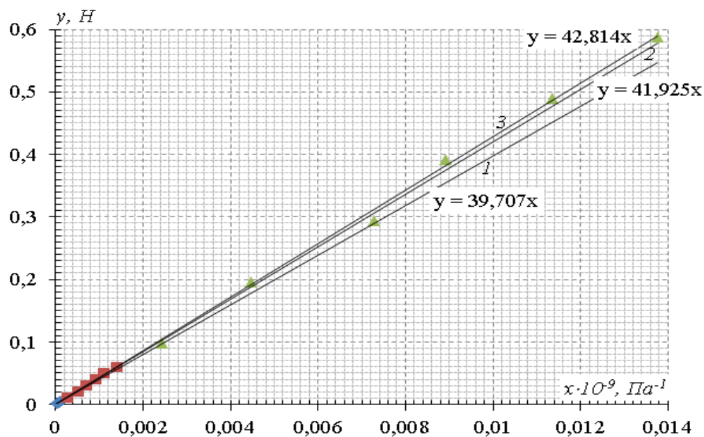
Рис. 3. Графік для визначення модуля зсуву необробленої пружини: d_1 – синій (1); d_2 – червоний (2); d_3 – зелений (3).
