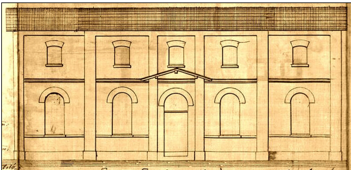
Ilustracja 25: Projekt rozbudowy dawnej olejarni w Małobądzu przez spółkę P. Strahl & Krins, budynek ekstraktora, 1886 (wydział ekstrakcji otwarto 1890)
