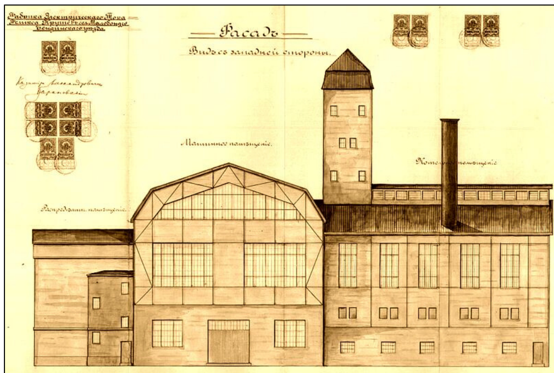
Ilustracja 5: Projekt elektrowni w Małobądzu, 1913
