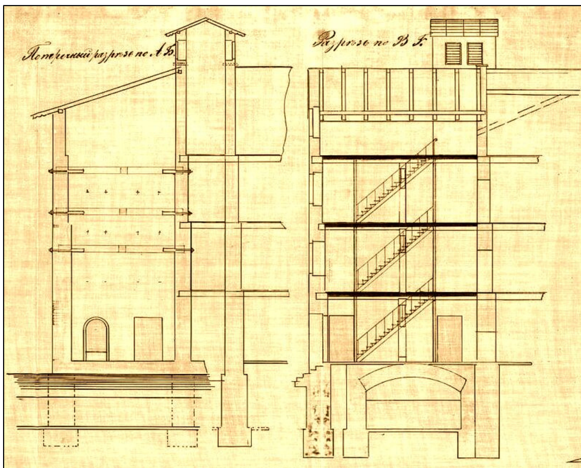
Ilustracja 20: Projekt rozbudowy dawnego młyna [I] w Małobądzu przez spółkę P. Strahl & Krins, 1889
