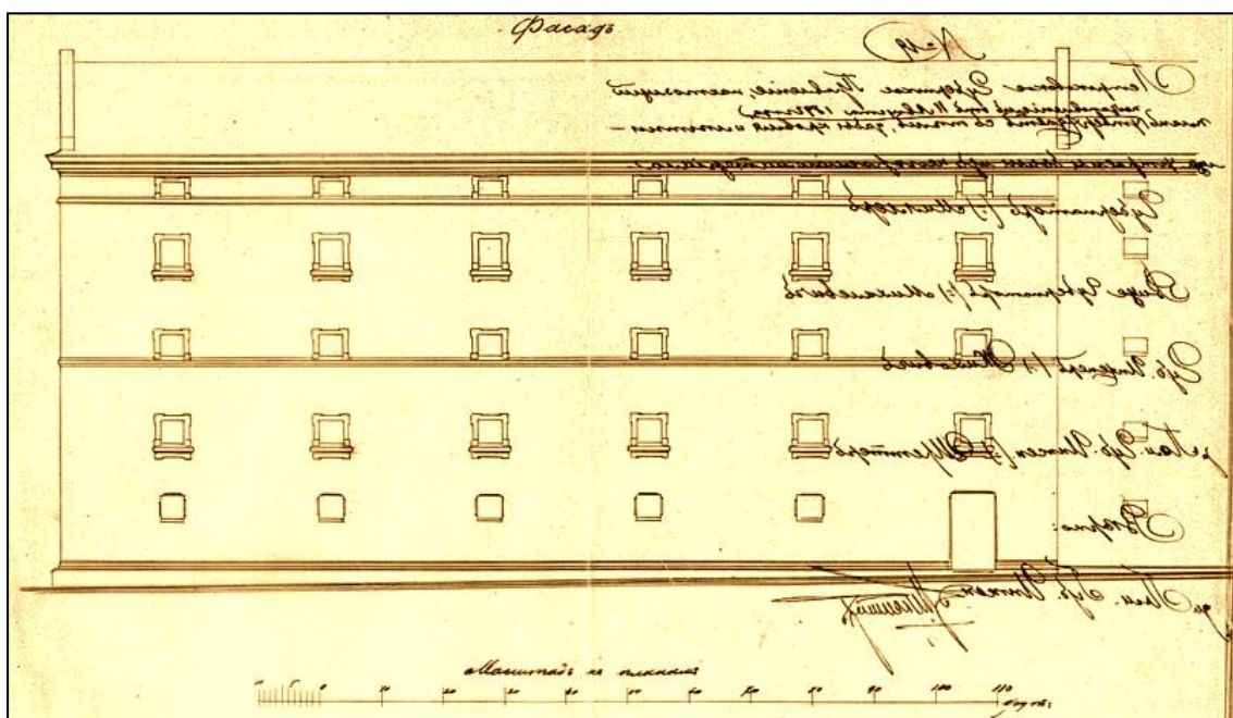
Ilustracja 21: Projekt rozbudowy dawnego młyna [I] w Małobądzu przez spółkę P. Strahl & Krins, spichrz, 1892
