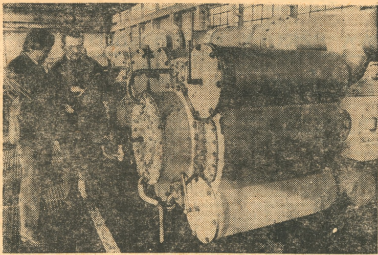
Kierownik tłoczni gazu w Świerklanach Ryszard Zieliński i maszynista tłoczni Alojzy Mika sprawdzają parametry gazu tłoczonego do naszych mieszkań. Zdj. Z. Keller
