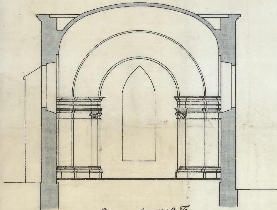
Querschnitt E.F.
