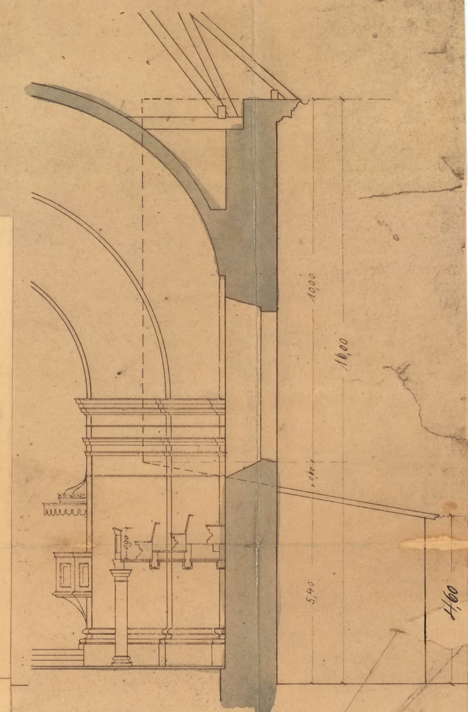
SCHNITT A-B.
