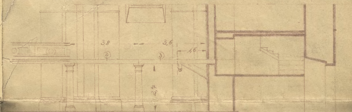
Schnitt cd.
