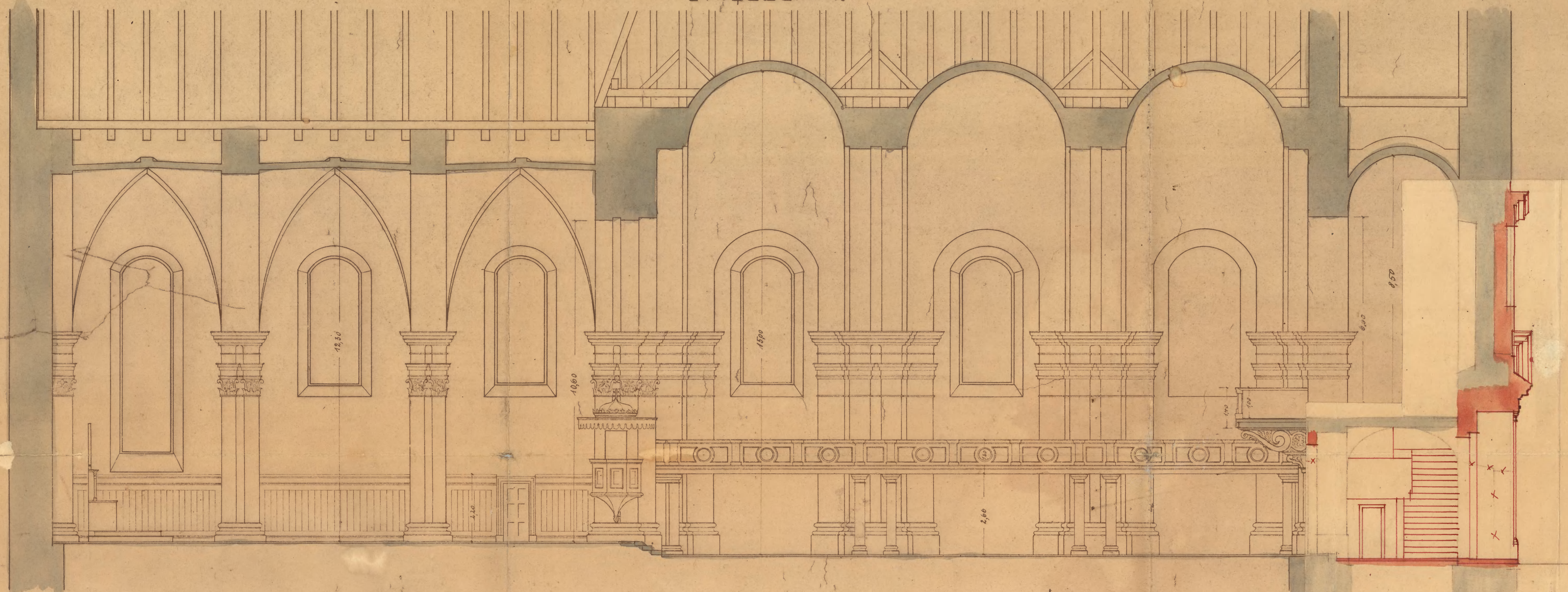
LÄNGSSCHNITT.
