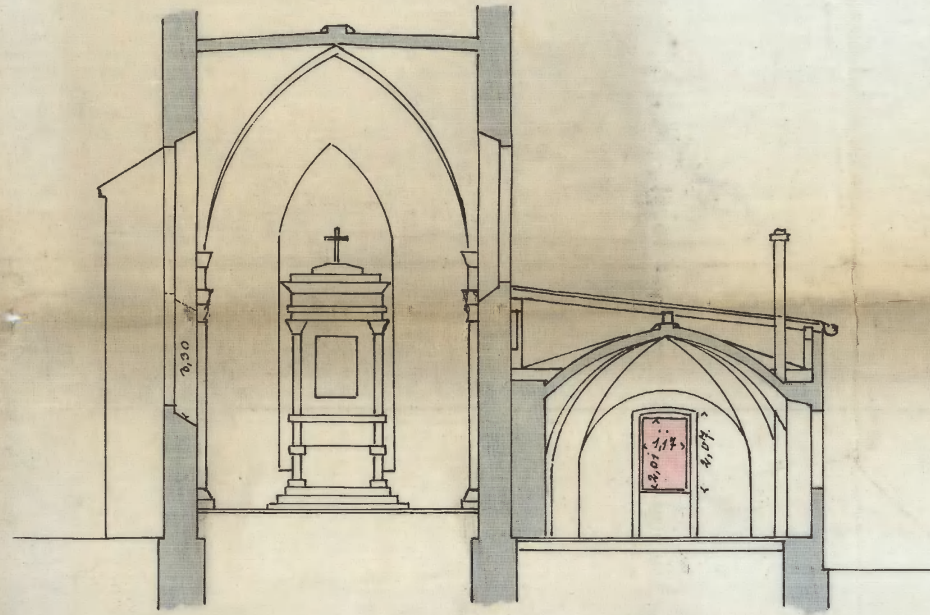
Querschnitt C.D.
