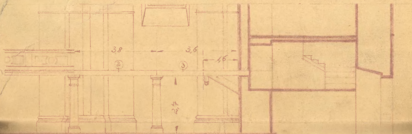
Schnitt cd.
