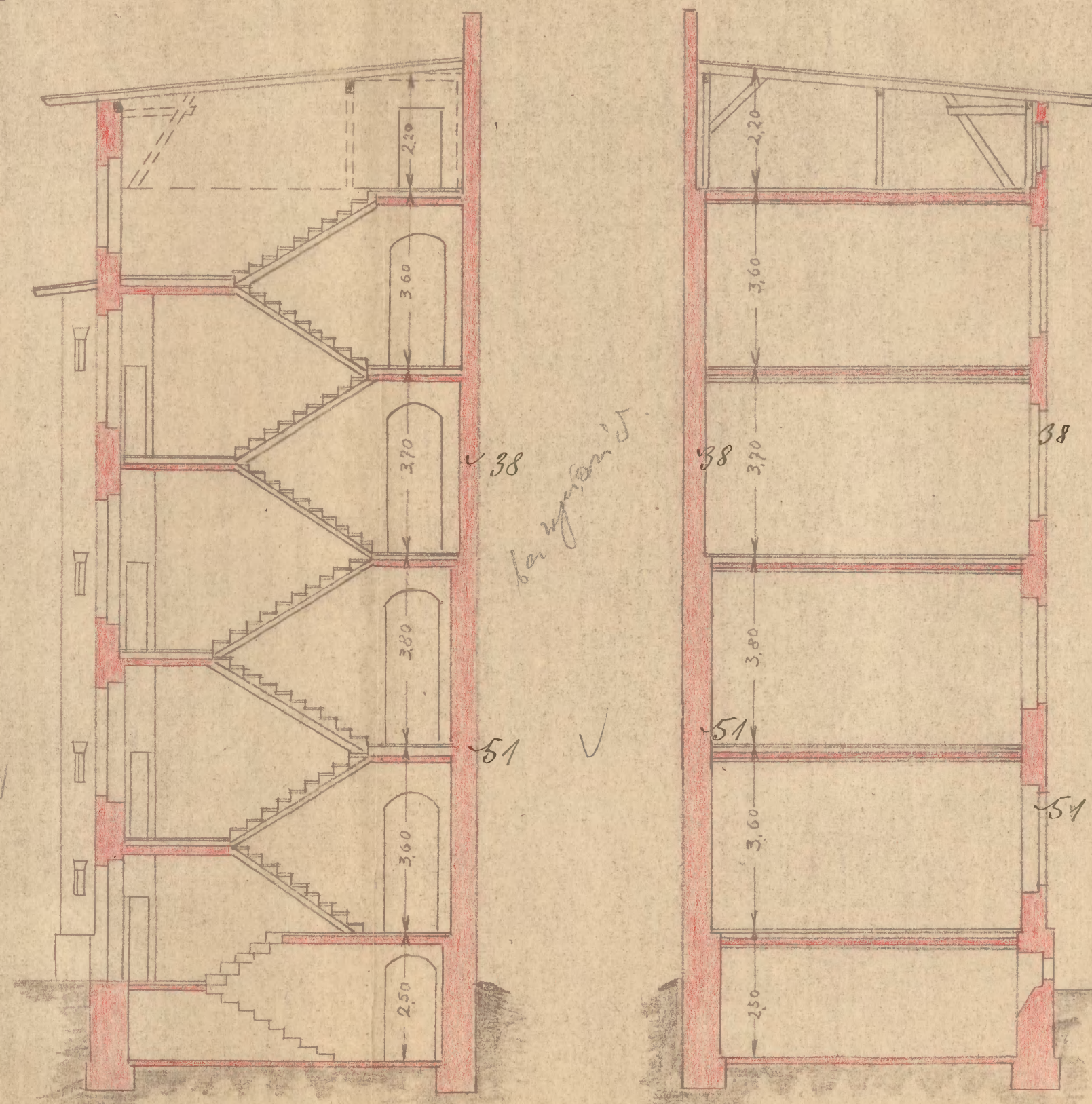
Schnitt C-D
