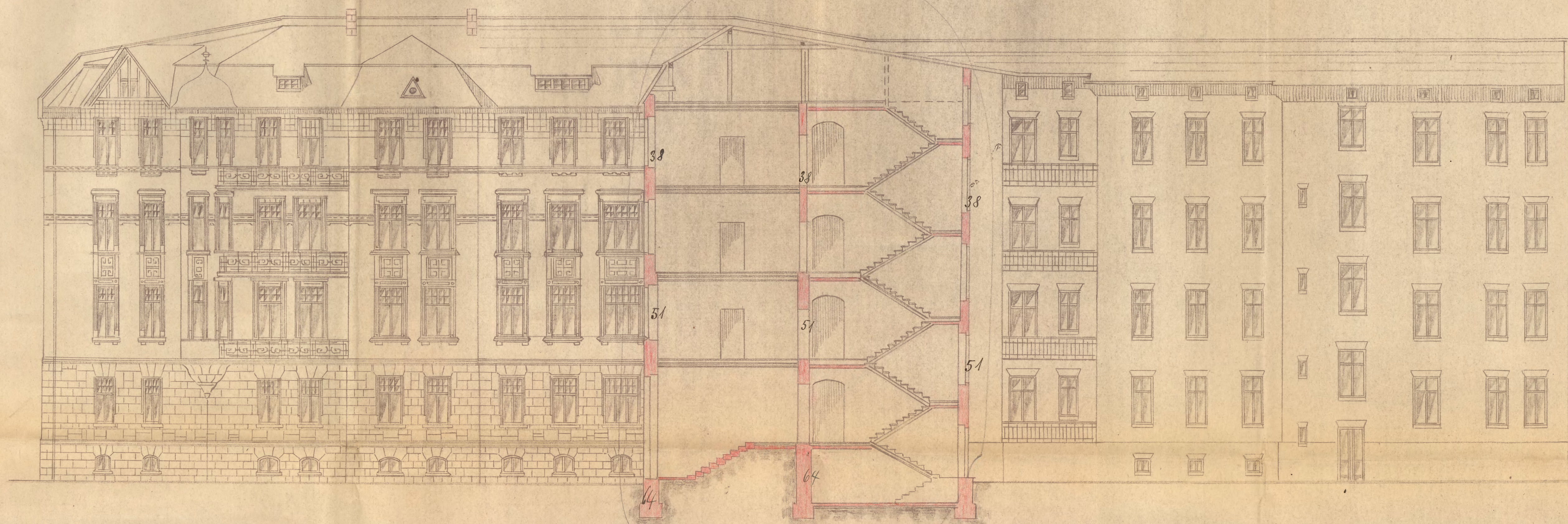
Schnitt A-B
