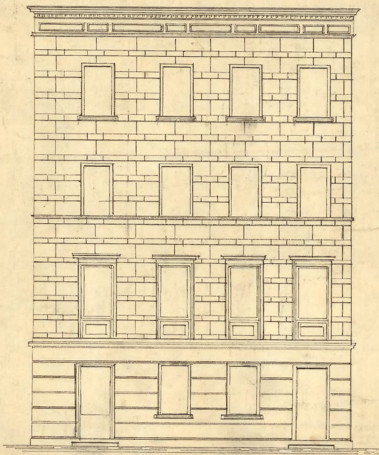
Ansicht von der Rittersstrasse.
