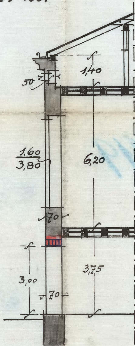
Schnitt.
