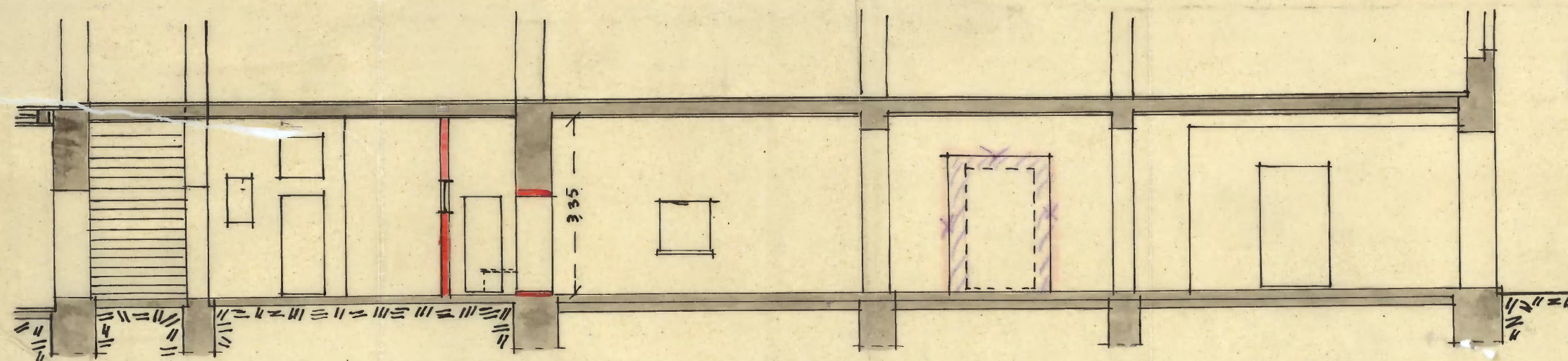
LÄNGENSCHNITT. 1:100.
