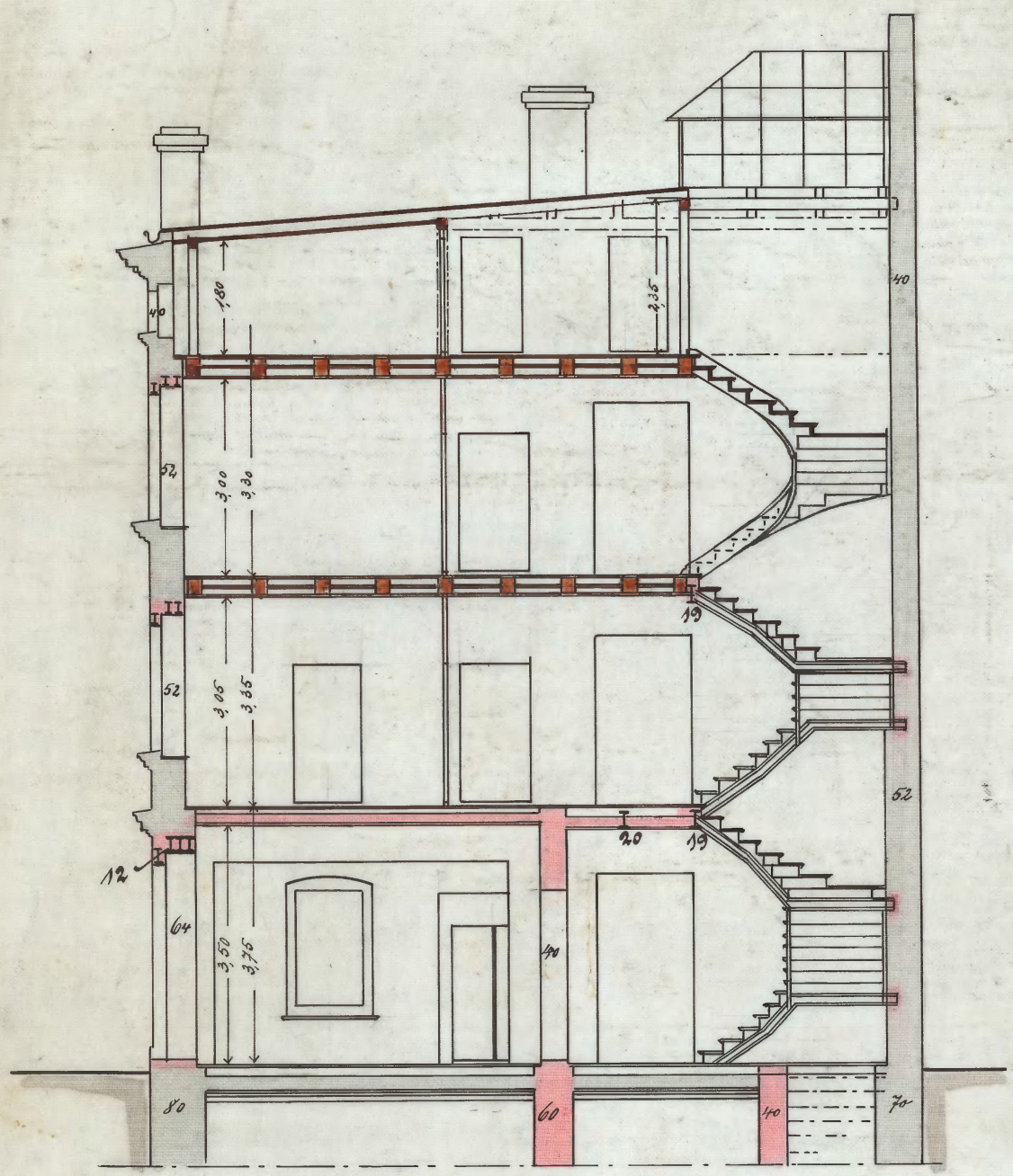
Schnitt c-d.
