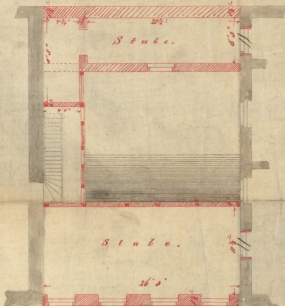
2. Stockwerk.
