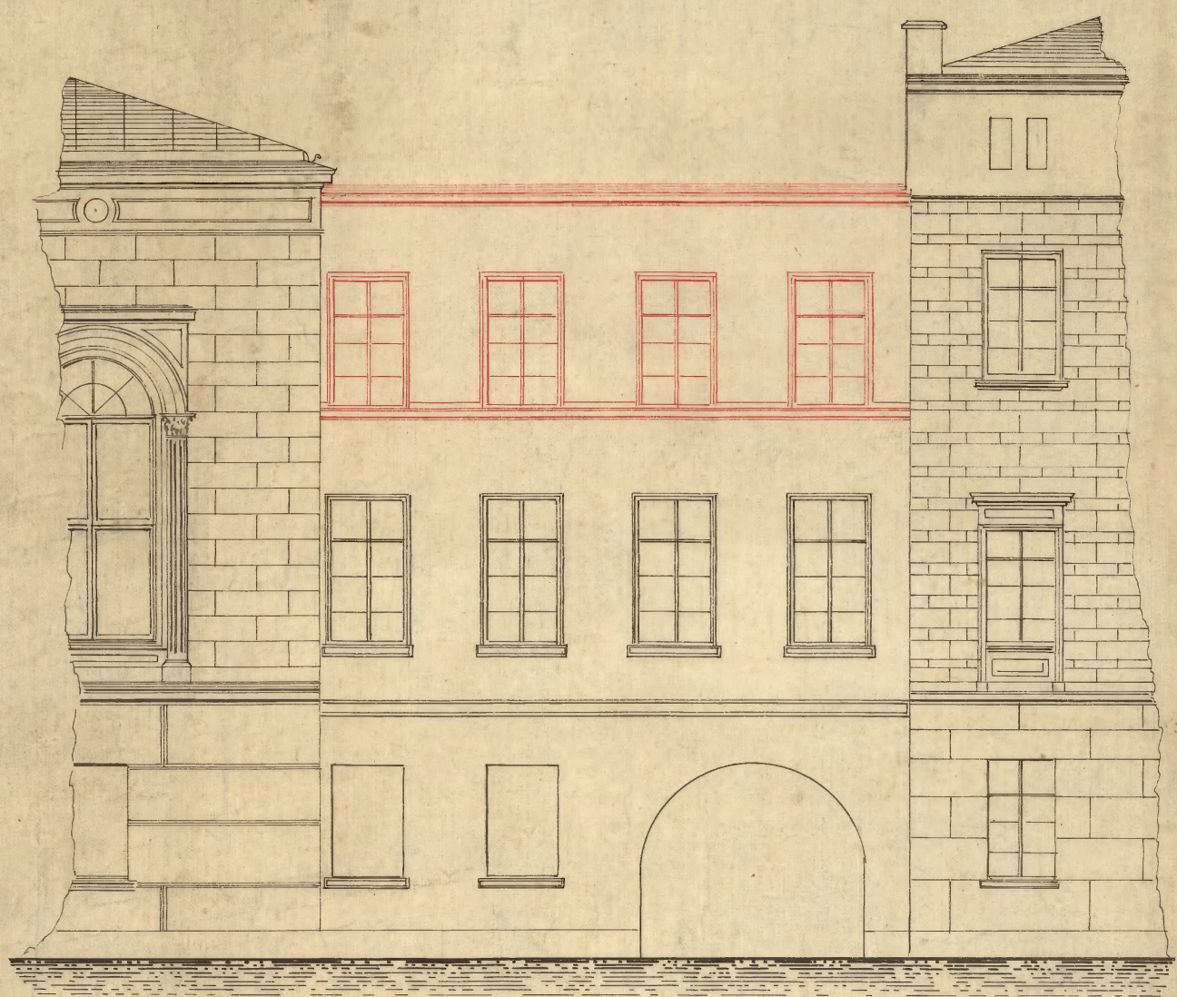
Ansicht.
