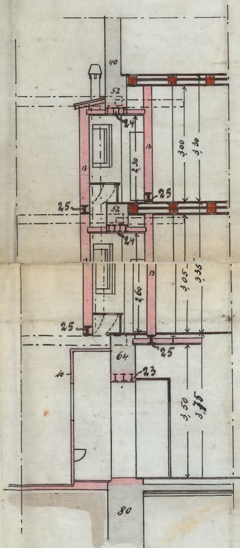
Schnitt l-m.
