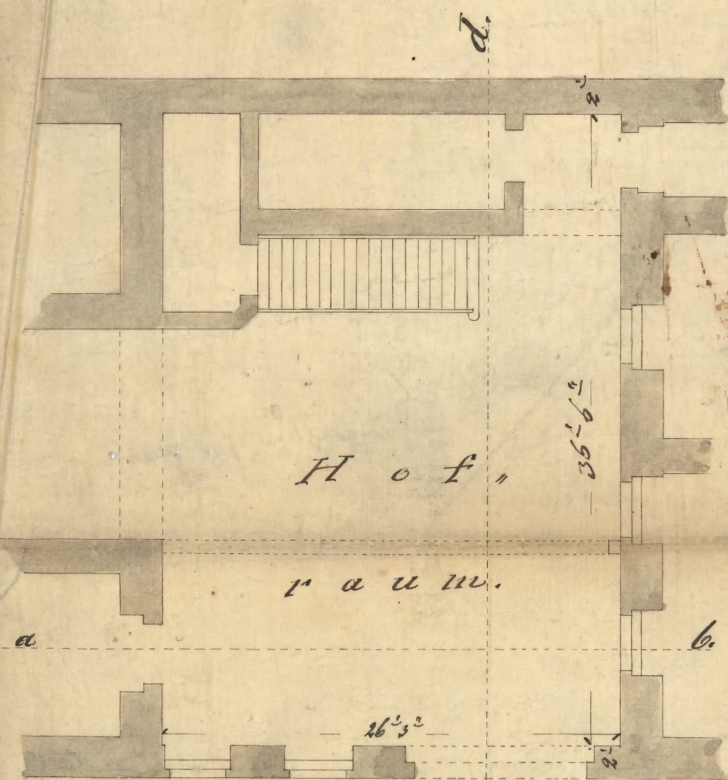
Erdegeschoss.
