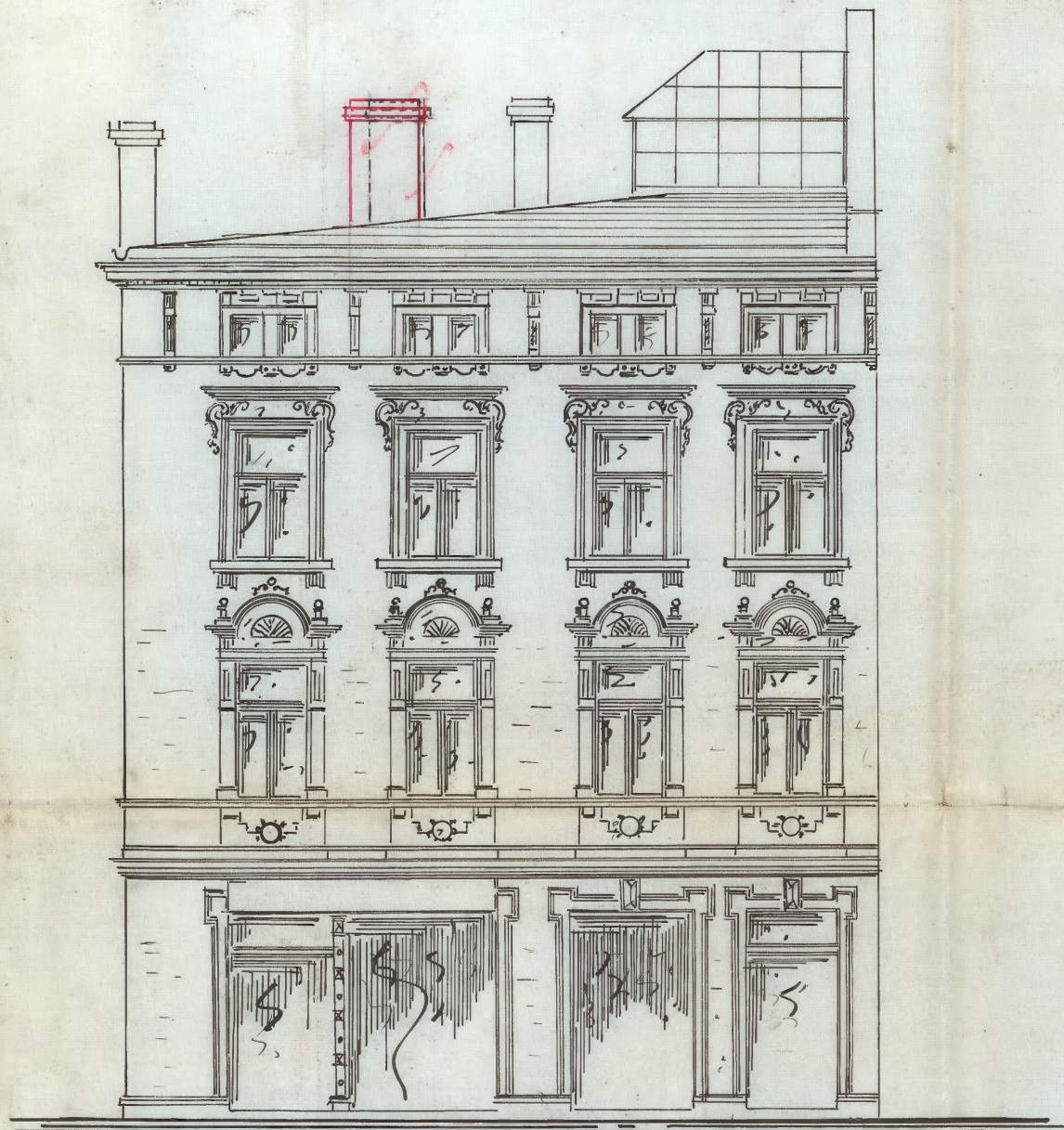
Ansicht von der Ritterstraße
