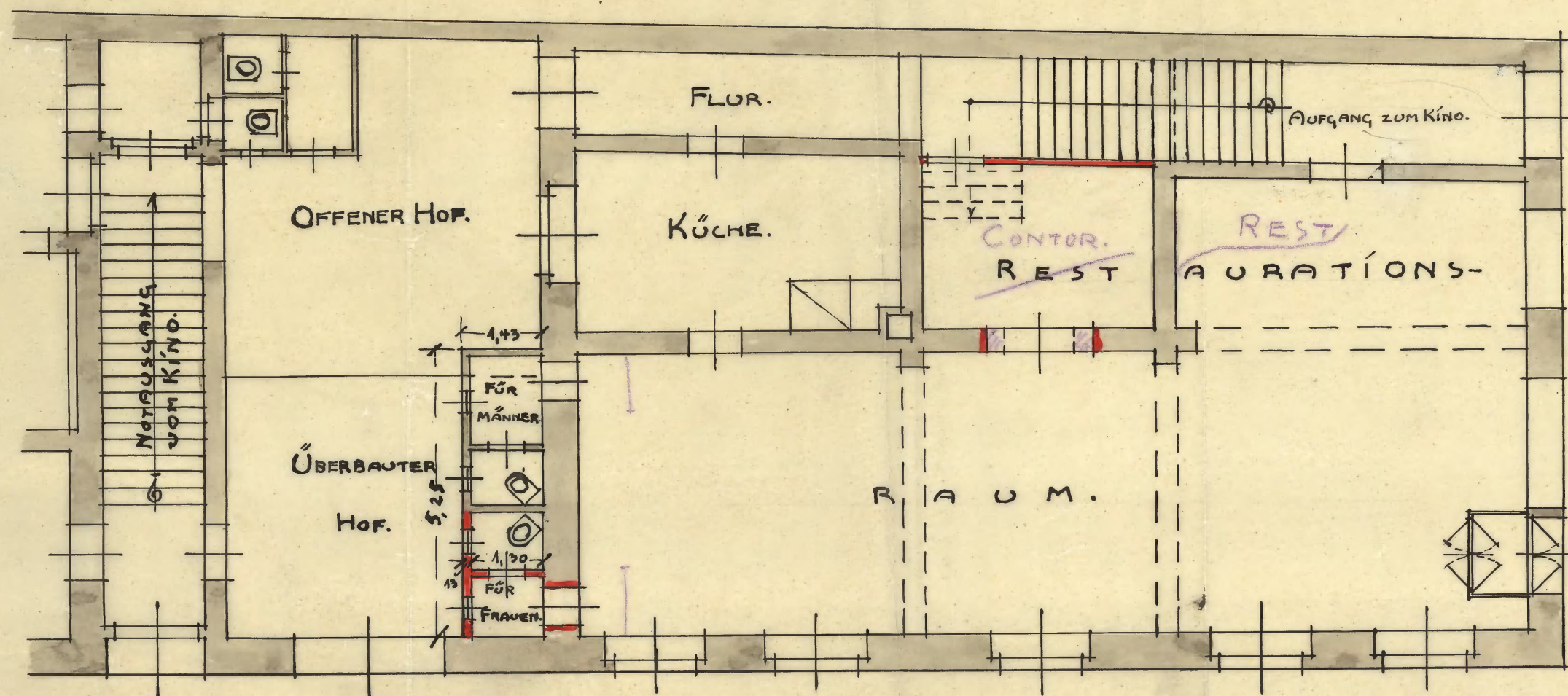
ERDGESCHOSS. 1:100.
