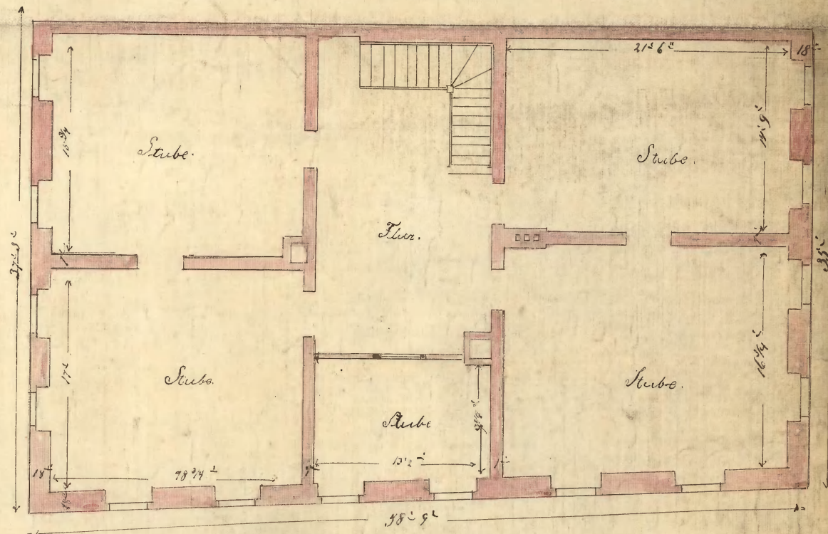
Grundriss der neuen 3 ten Etage.
