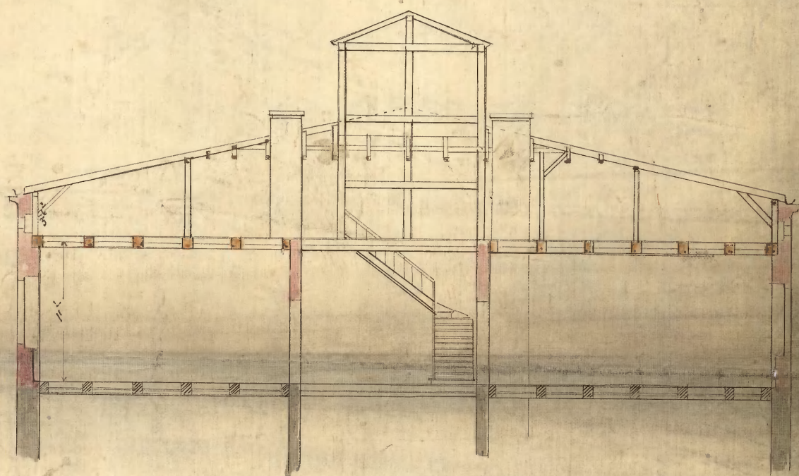
Längenprofil.
