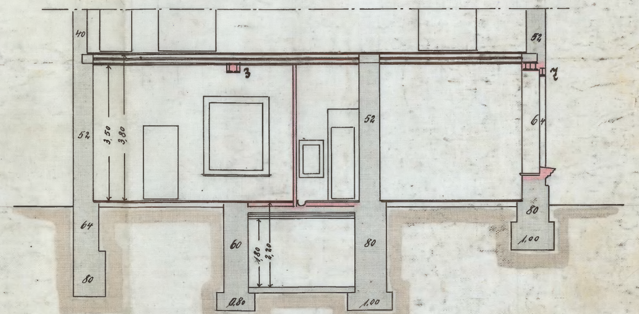
Schnitt g-h.
