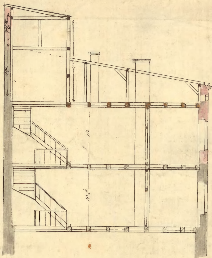
Querprofil.
