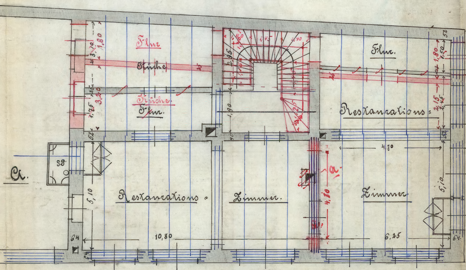
3. Geschoß.
