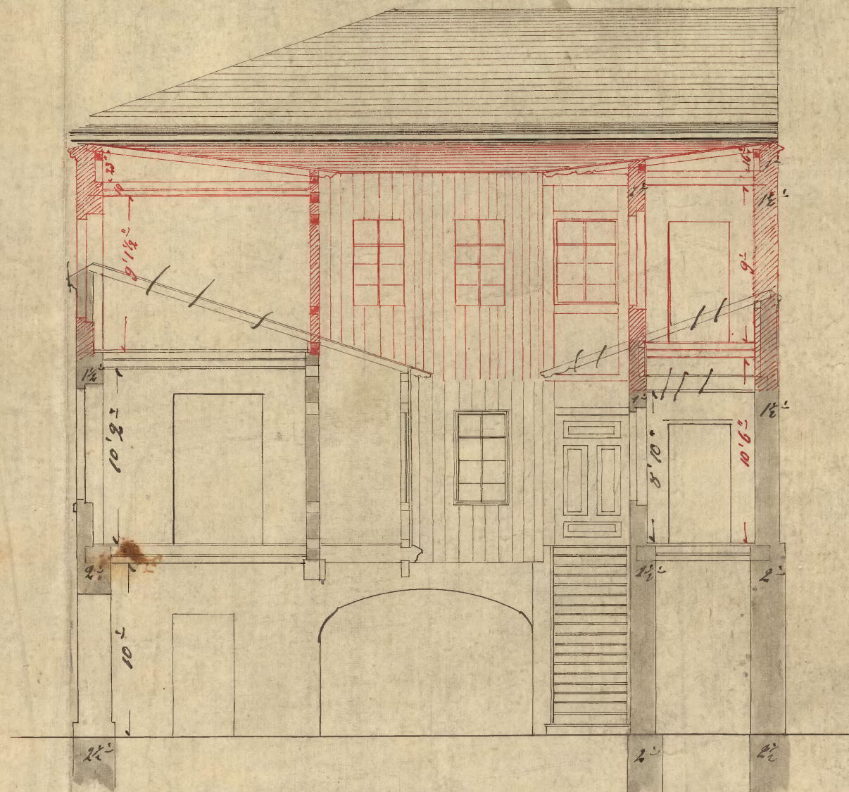
Querdurchschnitt c. d.
