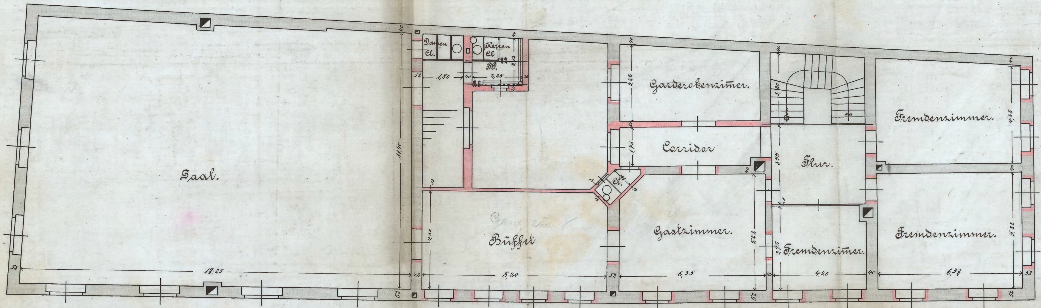
I. & II. Etage.
