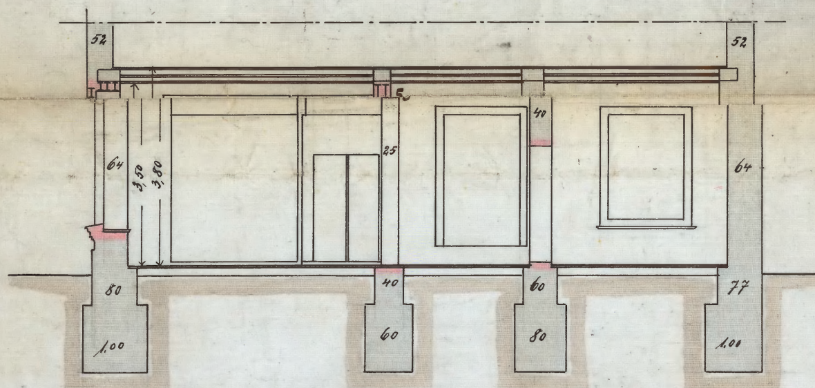
Schnitt i-k.
