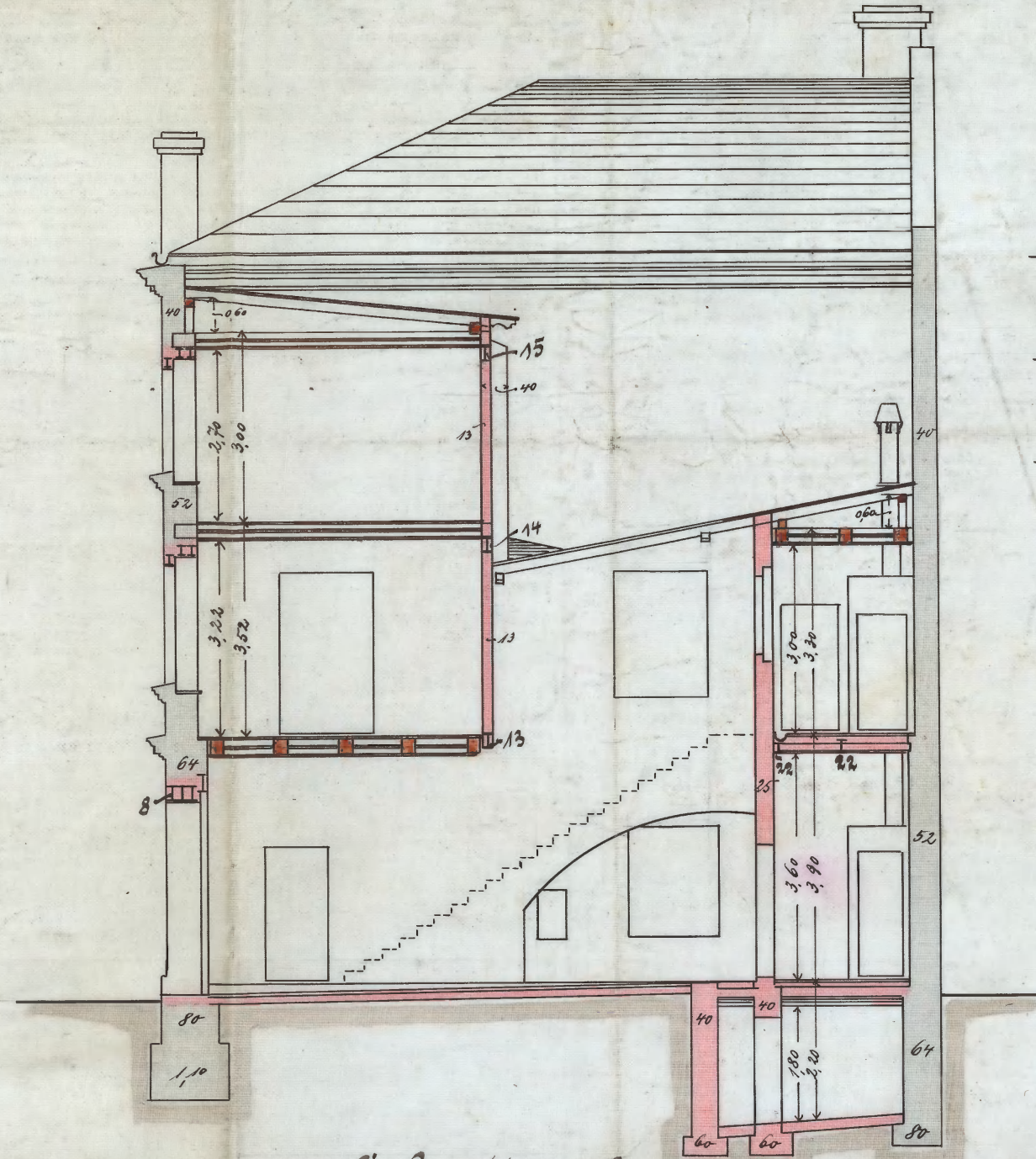
Schnitt e-f.
