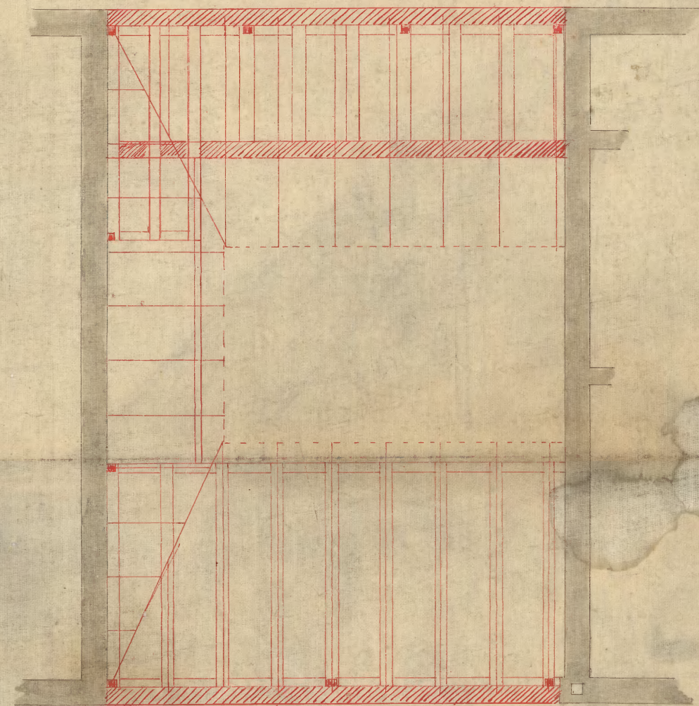
Dachbalkenlage.
