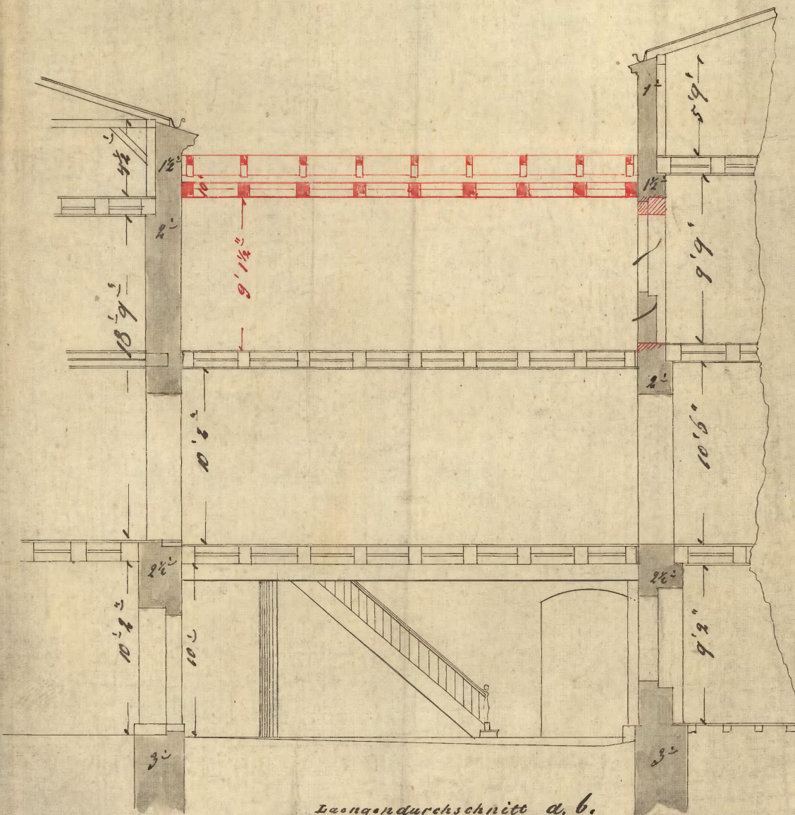
Längendurchschnitt a. b.
