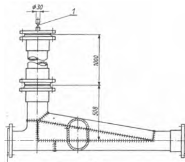
Doświadczalna konstrukcja „odpowietrzacza” i zamontowanego nad nim „separatora sprężonego powietrza” z rurociągów podsadzkowych; zainstalowana w kopalni „Chorzów”
