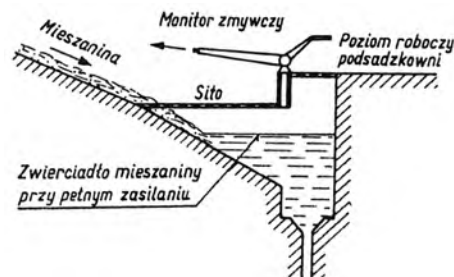
Rysunek opublikowany w maju 1959 roku w Wiadomościach Górniczych , ilustrujący występowanie lustra mieszaniny w leju podsadzkowym podczas pełnego zasilania rurociągu
