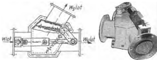
Przerzutnica klapowa PPK-2, kierująca mieszaninę podszkawką z rurociągu ścianowego na „wpust” skierowany za tamę
