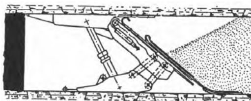
Schemat tamy ES-3. Przepona leży bezpośrednio na obudowie osłonowej
