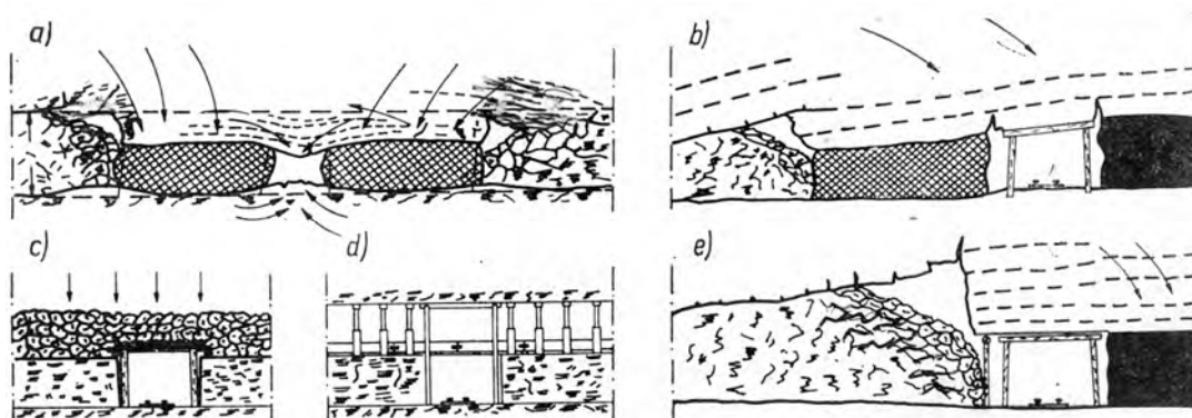
Szkice a) i b) ilustrują warunki utrzymania chodników chronionych pasami podsadzki. Szkice c) i d) przedstawiają chodnik wgłębny w strefie odprężonej oraz w fazie „przejściowej” przed zawaleniem stropu; e) chodnik na skraju calizny bez pasa podsadzki
