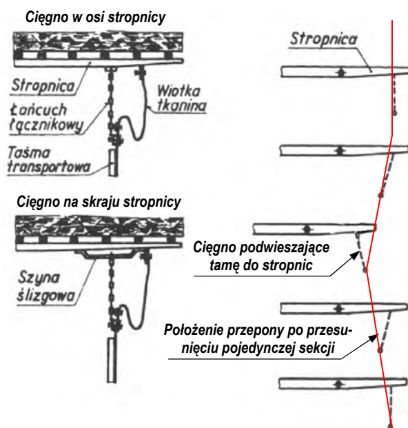
Schemat zawieszenia przepony tamy ES-5 na stropnicach obudowy zmechanizowanej
