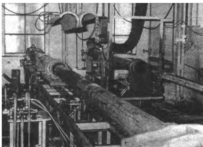
Specjalistyczna wylączarka realizująca zintegrowany proces formowania wykładziny gumowej i jej układania we wnętrzu czterometrowej rury podsadzkowej (RSG)
