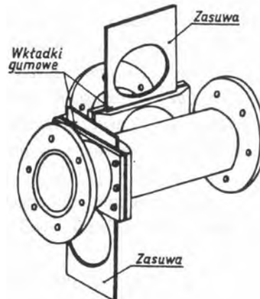
Przerzutnica trójkątowa (konstrukcja spawana) lansowana przez GIG w latach 1959–1962
