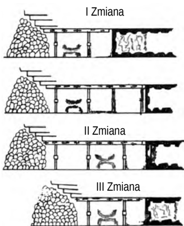
Schemat objaśniający trózmianowy, cykliczny sposób posuwania się przodka ścianowego, poprzez wybieranie kolejnych zabiorów
