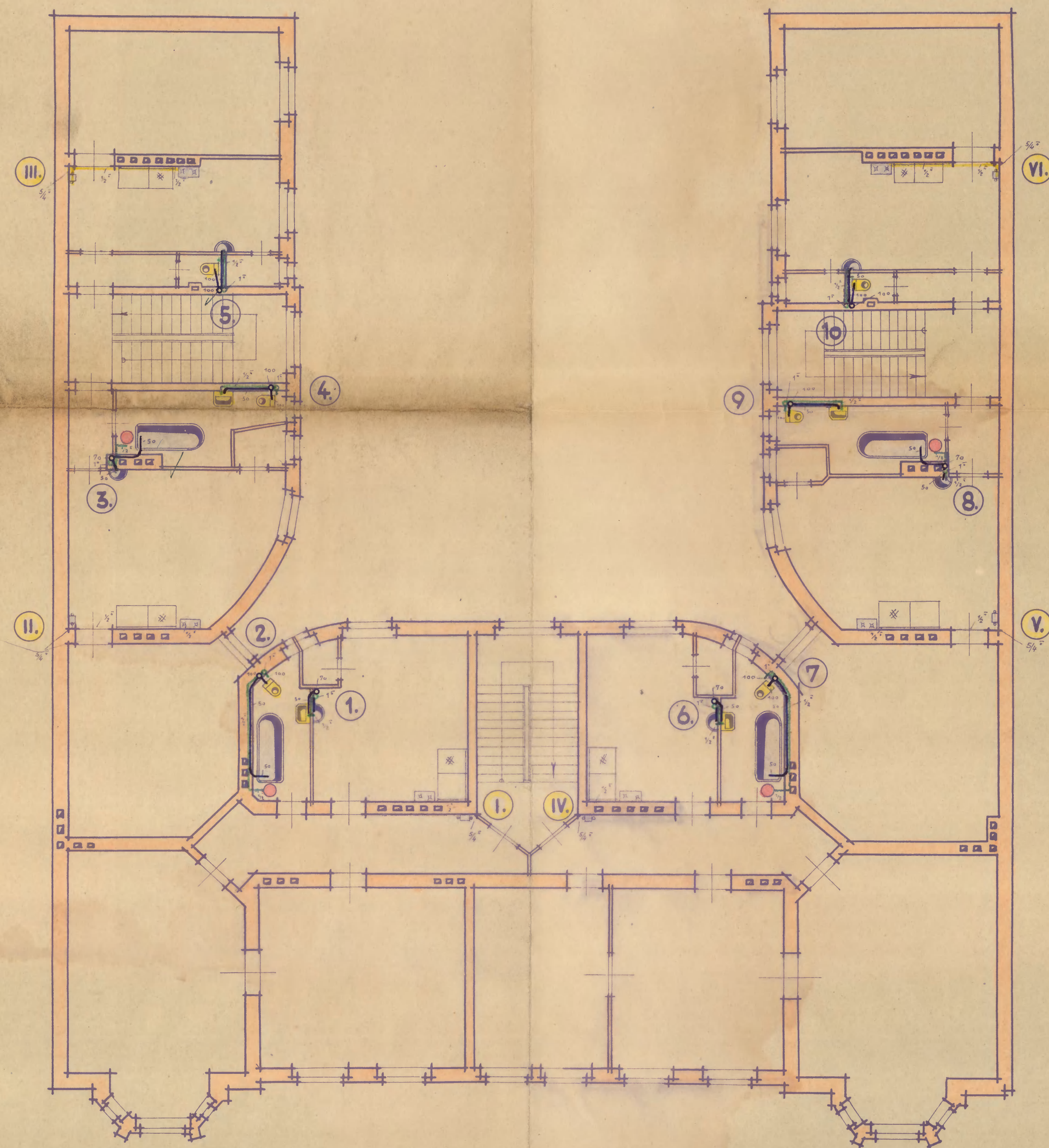
3. PIETRO 1:100
