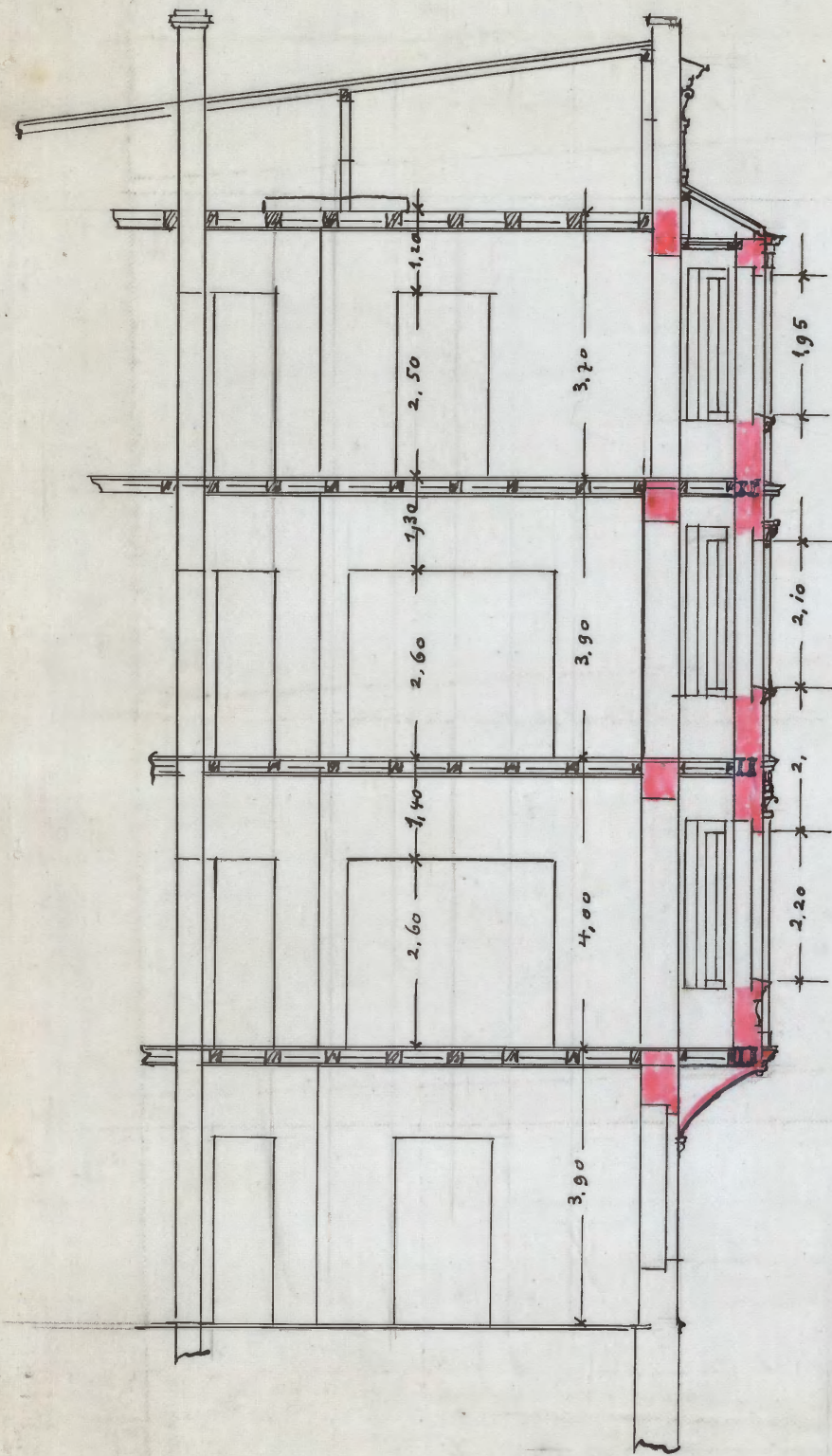
Schnitt
