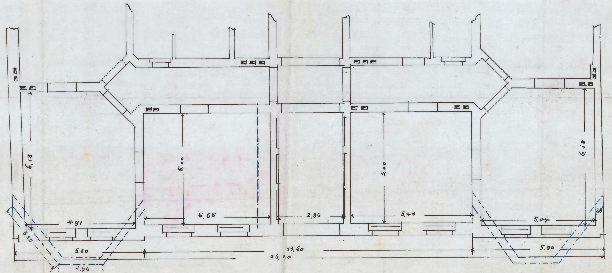
Erdgeschoss
