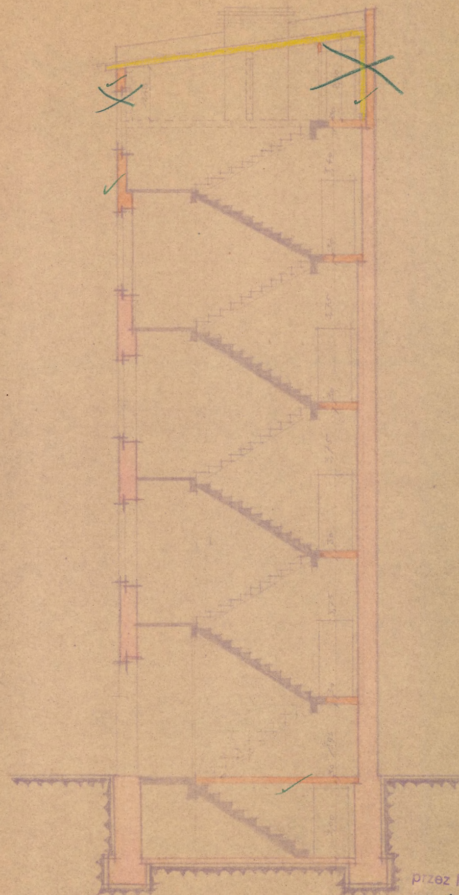
przekrój c-d
