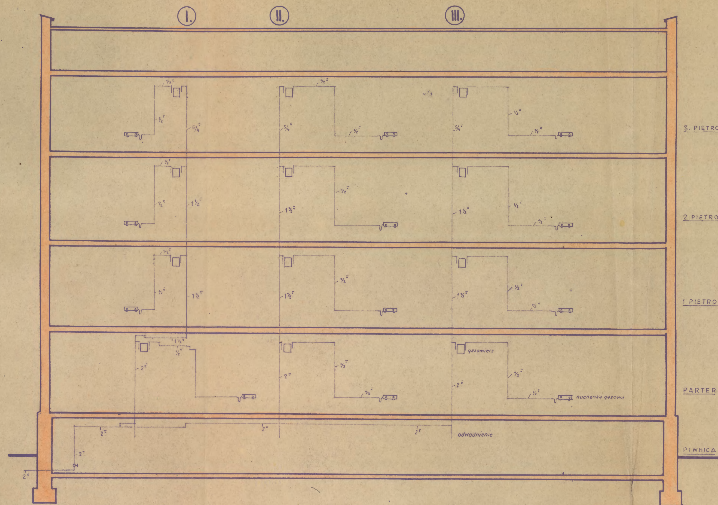
SCHEMAT PIONÓW GAZOWYCH I-III, PIONY IV-VI JEDYNYCZNIE
