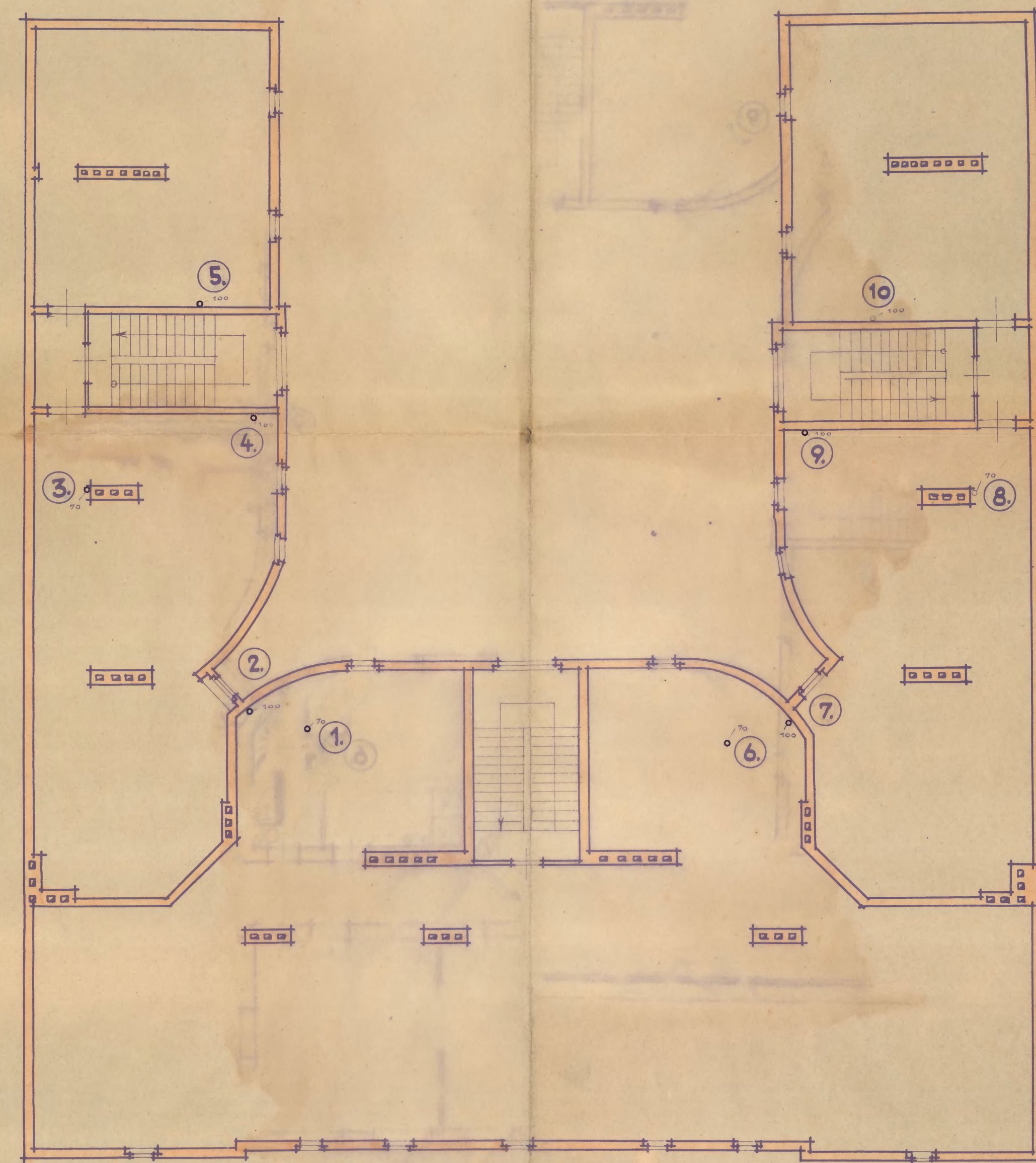
PODDASZE 1:100
