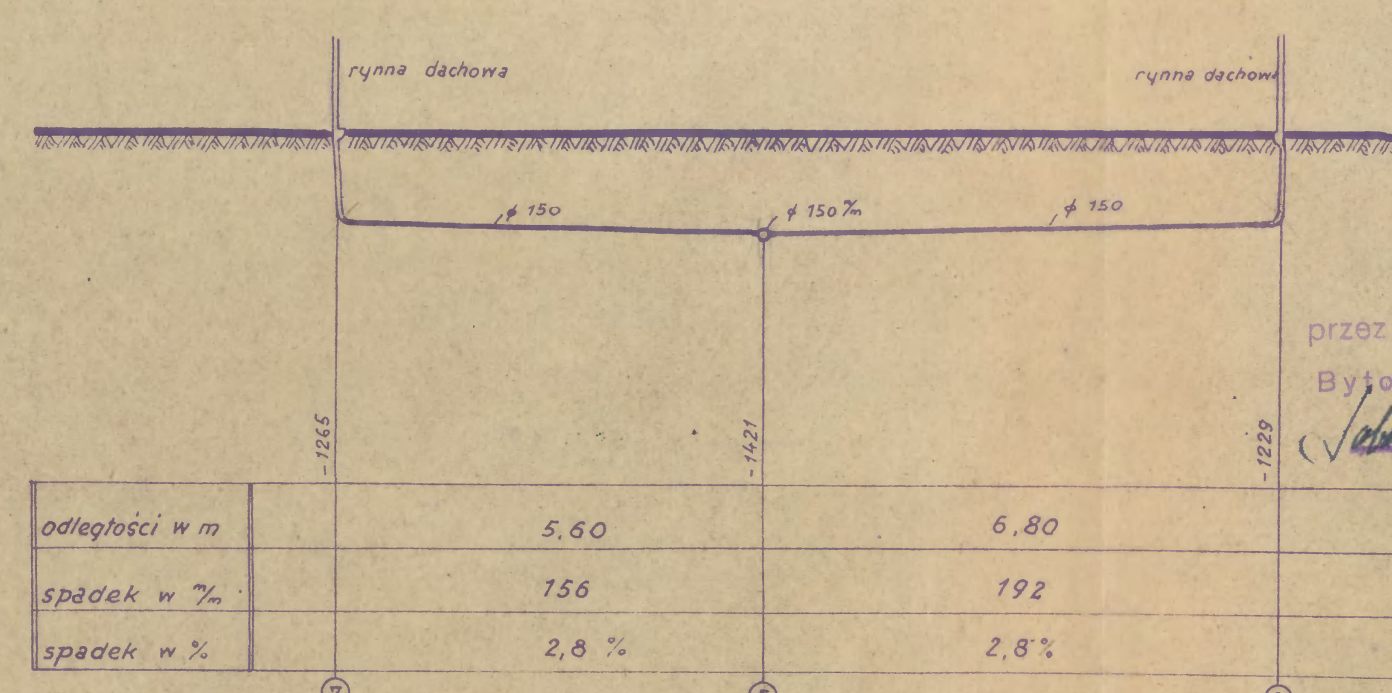
PRZĘKRÓJ POPRZECZNY KANAŁU DESZCZOWEGO 1:100
