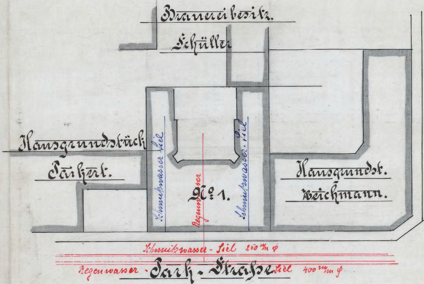
Lagerplan 1:500.
