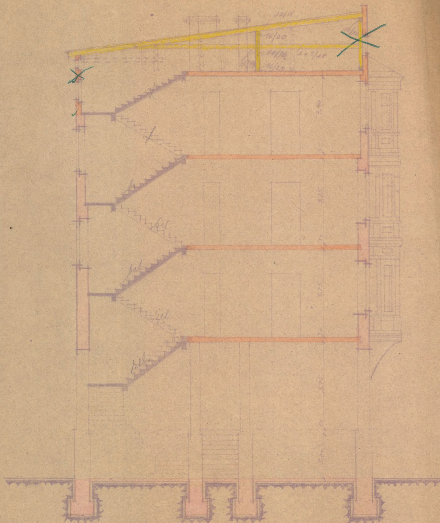
przekrój a-b
