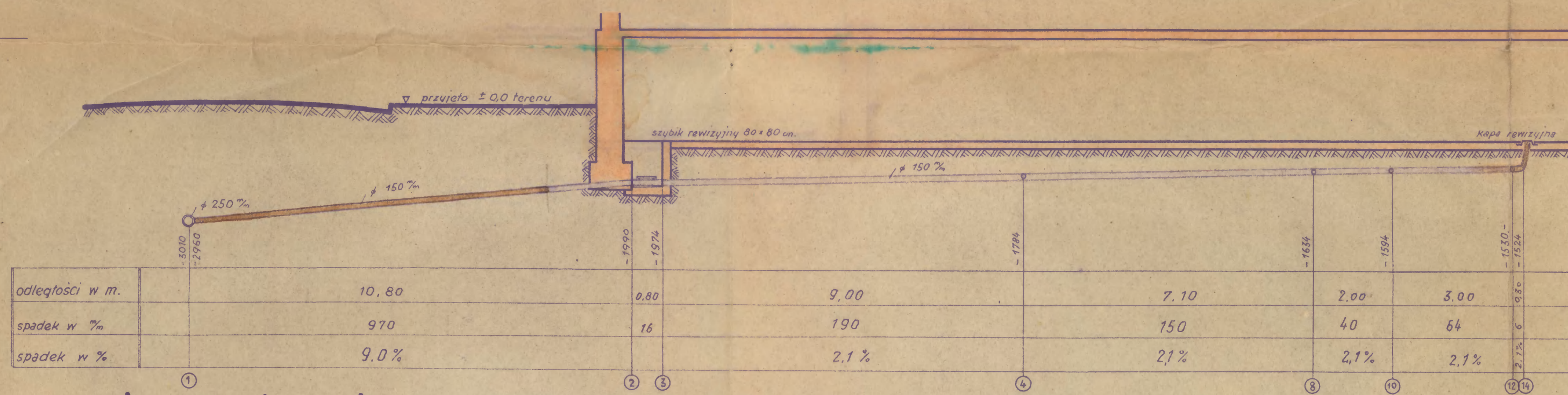
PRZĘKRÓJ PODŁUŻNY GŁÓWNEGO KANAŁU WEWNĘTRZNEGO WÓD BRUDNYCH 1:100
