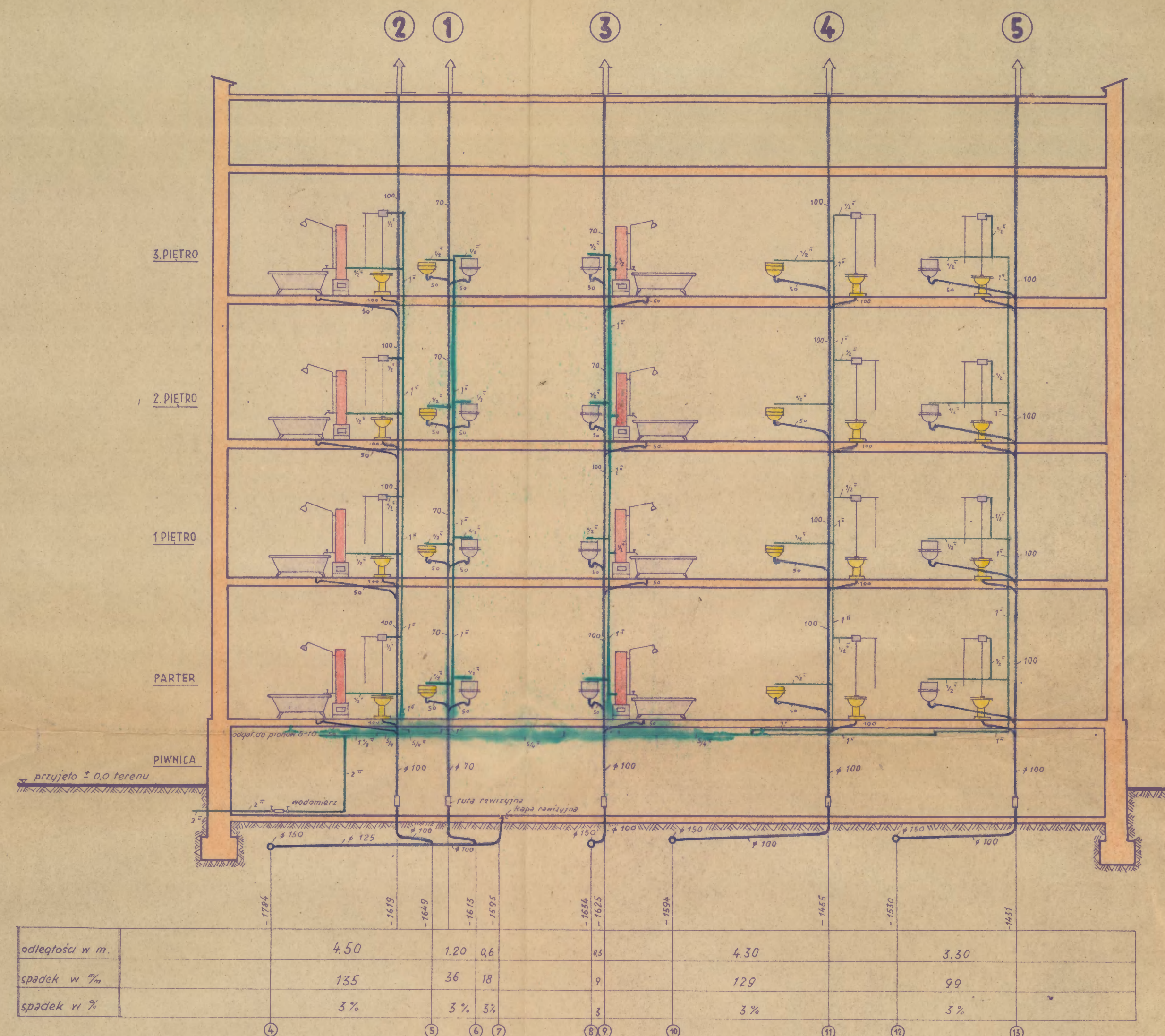
SCHEMAT PIONÓW KANALIZACYJNYCH I WODOCIĄGOWYCH 1-5 PIONY 6-10 JEDYNYCZNIE 1:100
