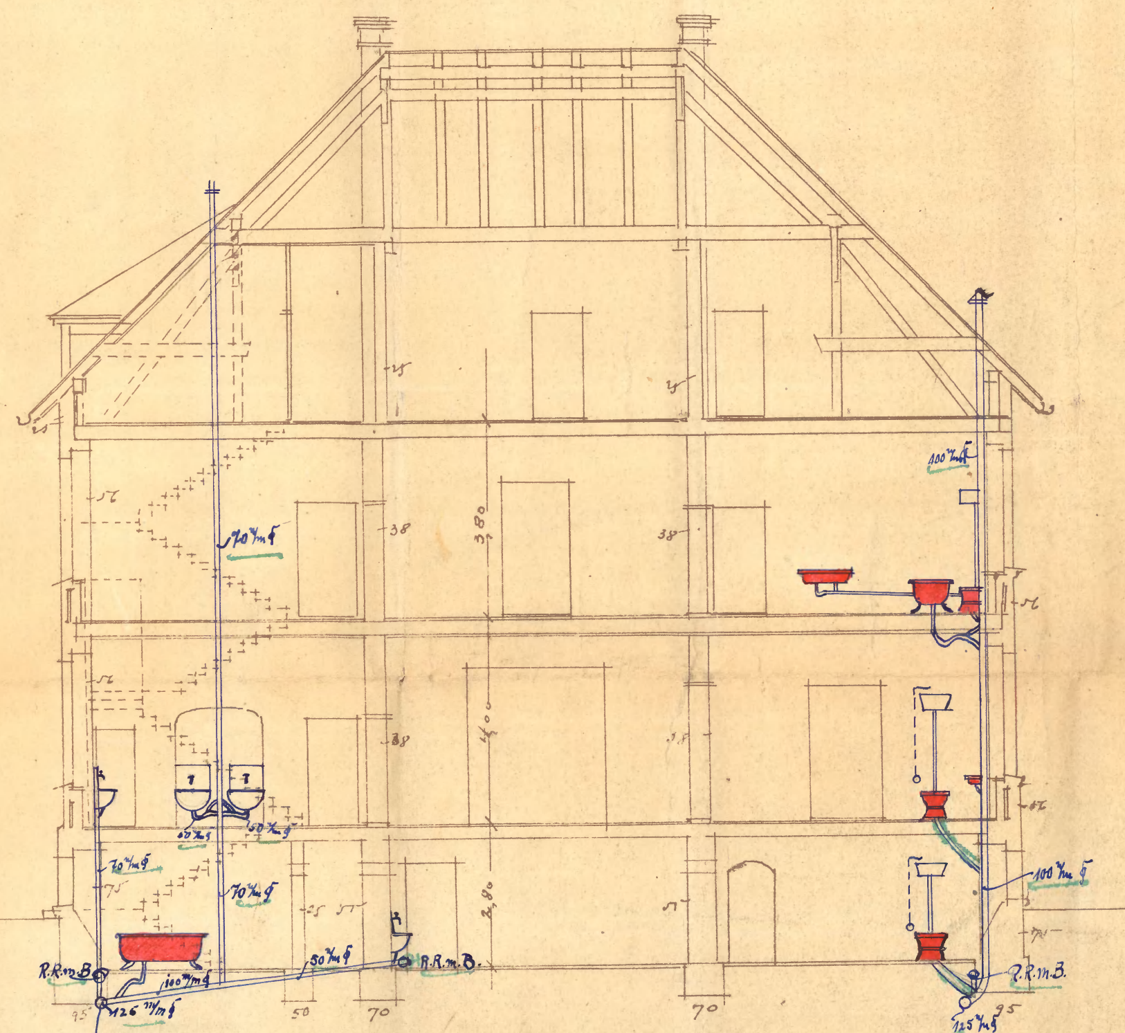
SCHEITTEL C-D.
