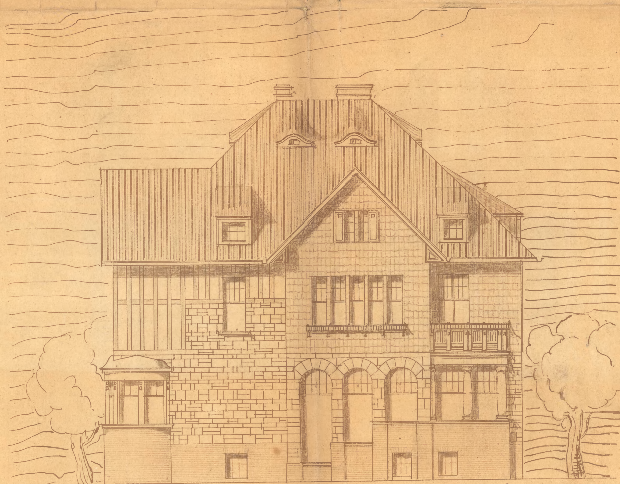
SEITENANSICHT.
