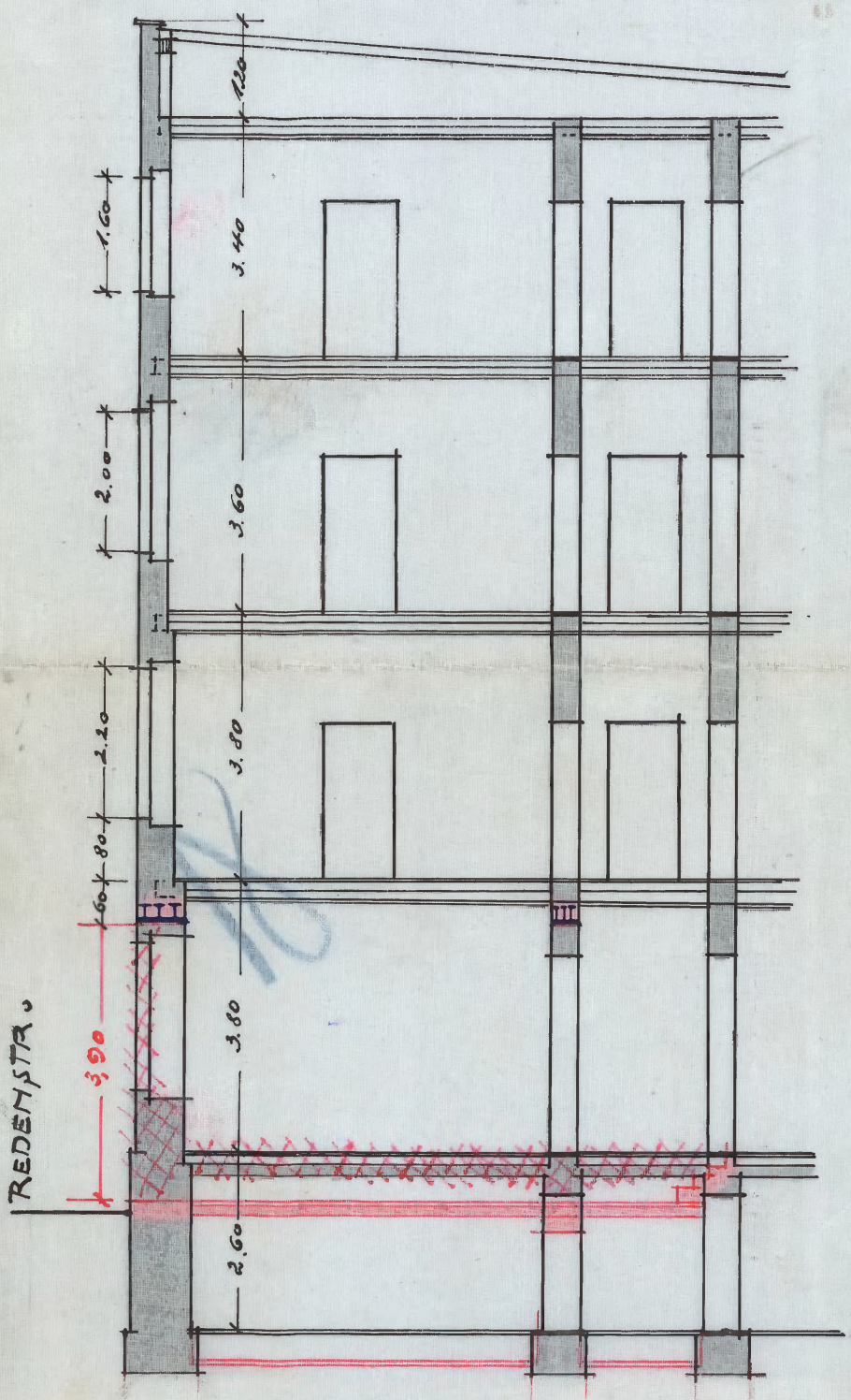
SCNITT.
