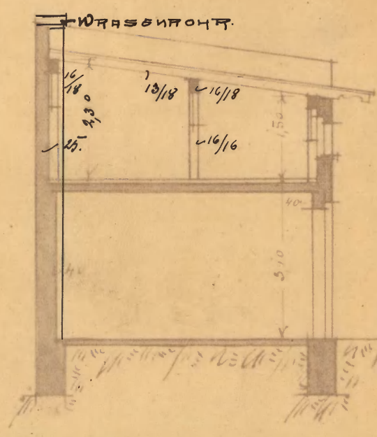
Schnitt C-D
