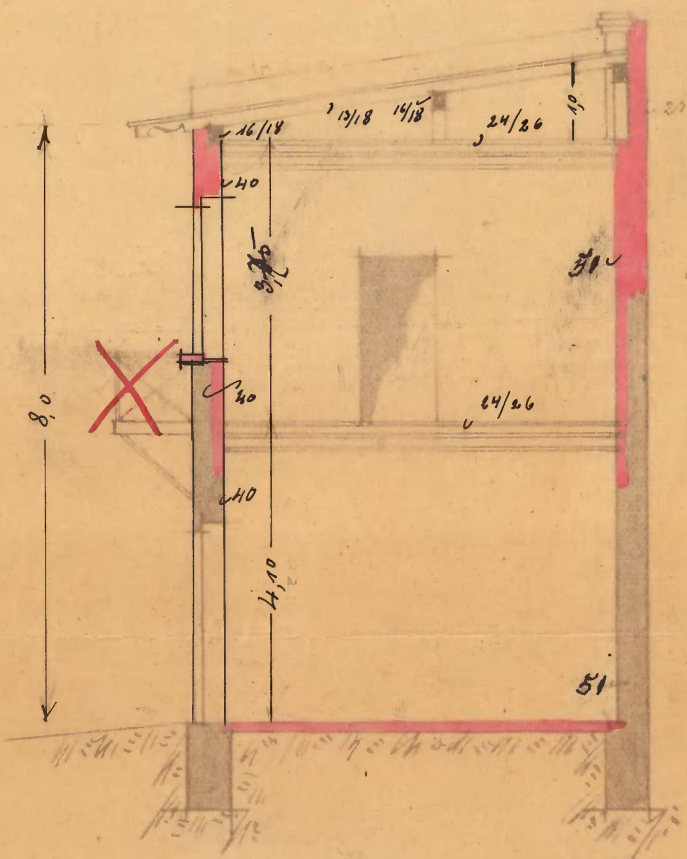
Schnitt A-B
