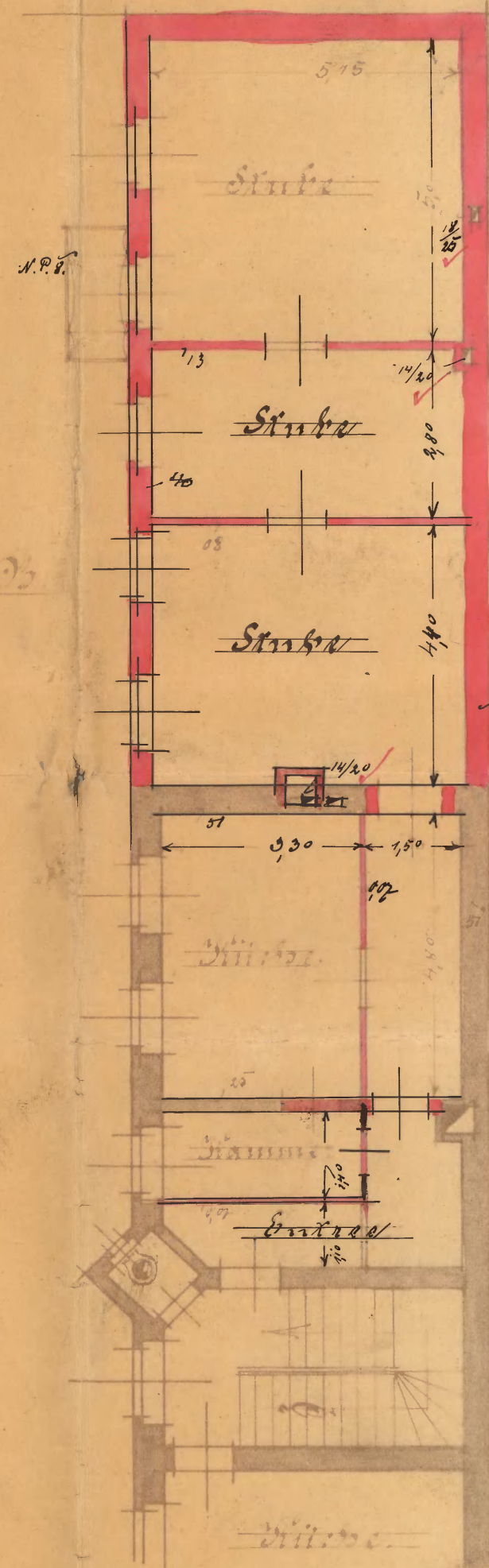
I. Obergeschoss
